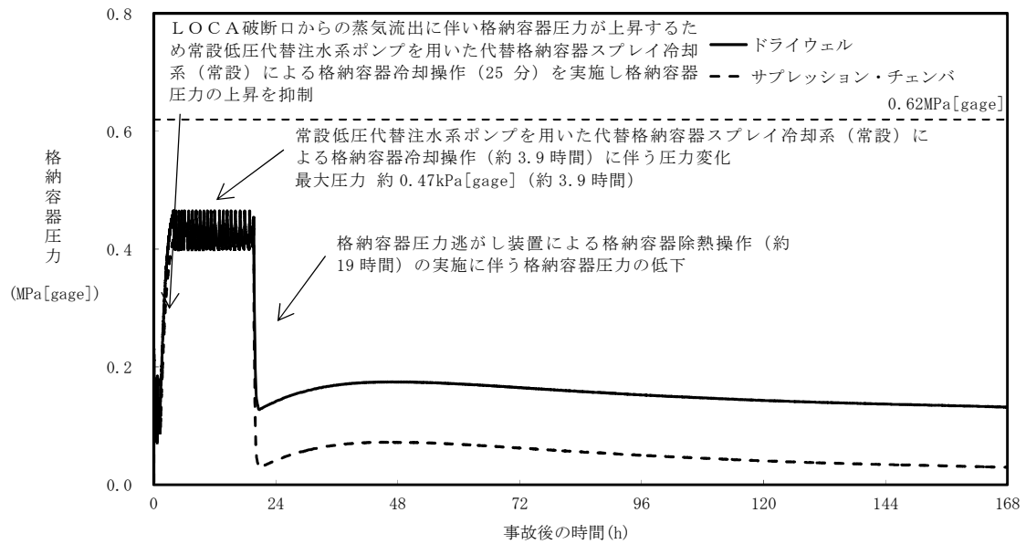
第 5.2.2.4 図 「雰囲気圧力・温度による静的負荷（格納容器過圧・過温破損）（代替循環冷却を使用しない場合）」における格納容器圧力の推移
