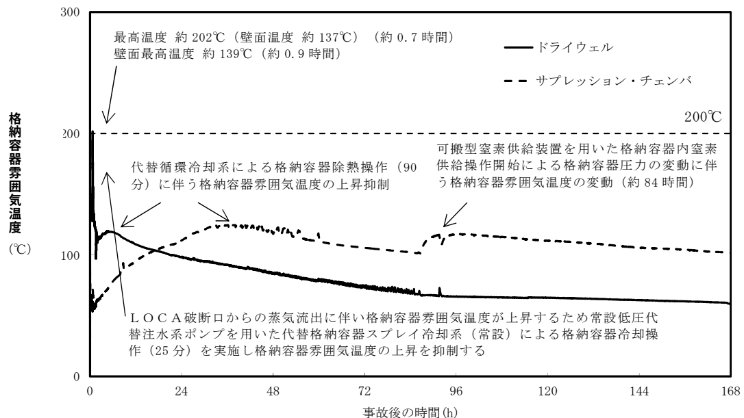
第 5.2.2.3 図 「雰囲気圧力・温度による静的負荷（格納容器過圧・過温破損）（代替循環冷却系を使用する場合）」における格納容器温度（気相部）の推移
