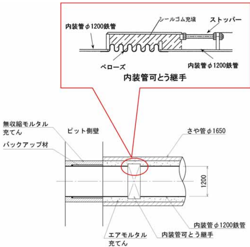
第3図 海水引込み管，緊急用海水管とピットとの接続部（イメージ図）
