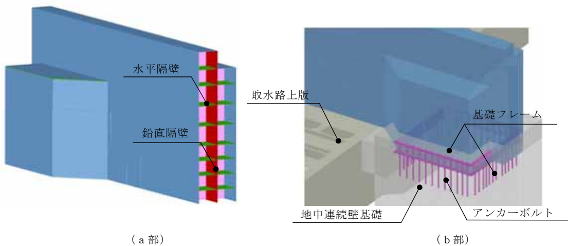
第 3.1-3 図 構造形式毎の防潮堤構造図 (1/4)
