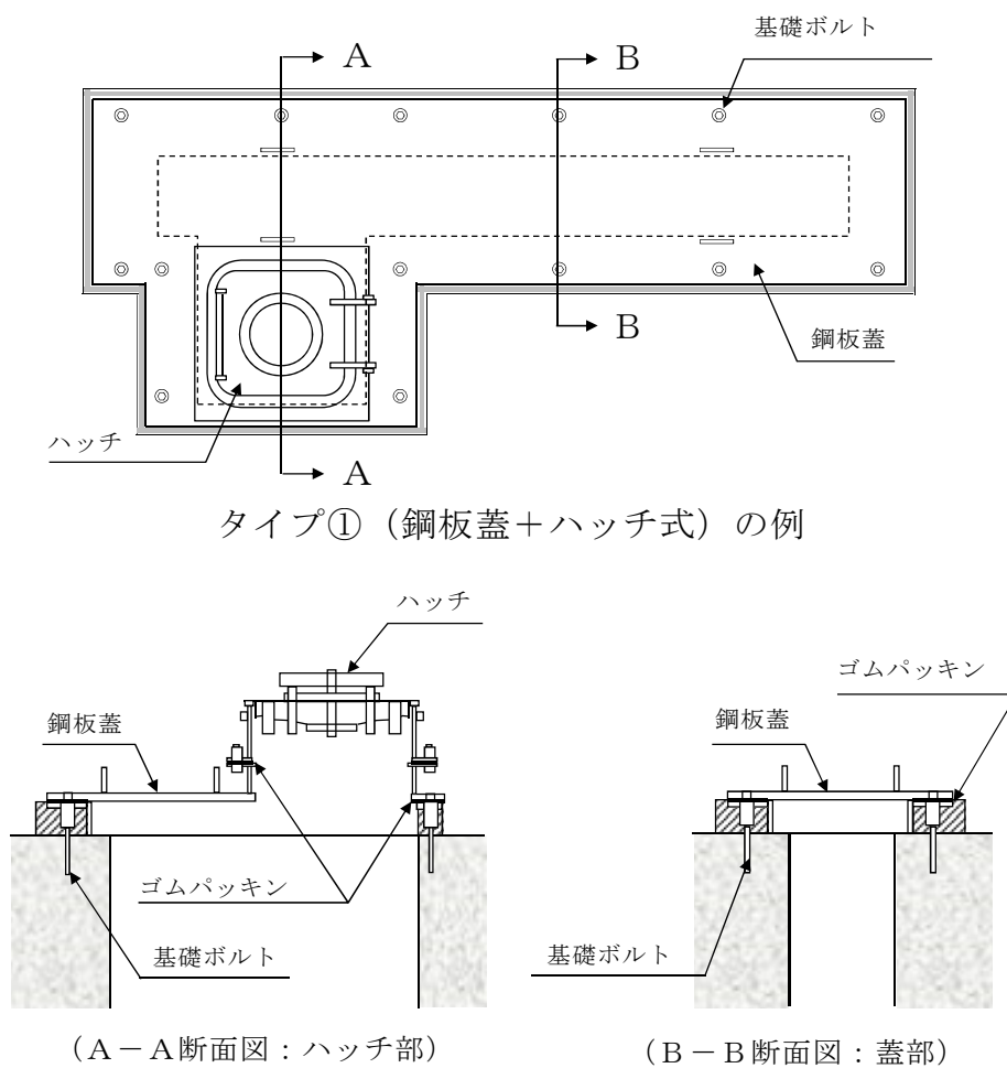
第 2. 2. 1-2 図 取水路点検用開口部浸水防止蓋構造図
