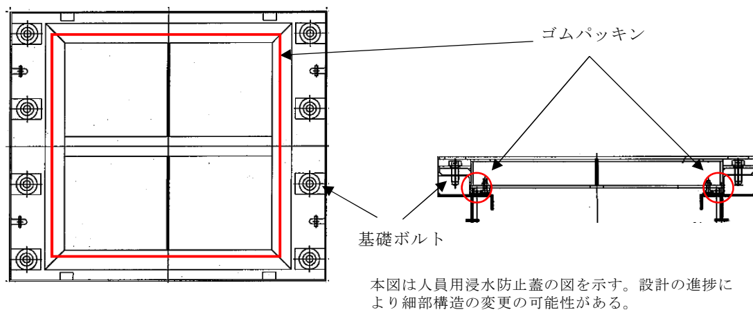
第 2. 2. 2-9 図 緊急用海水ポンプピット人員用開口部浸水防止蓋構造図
