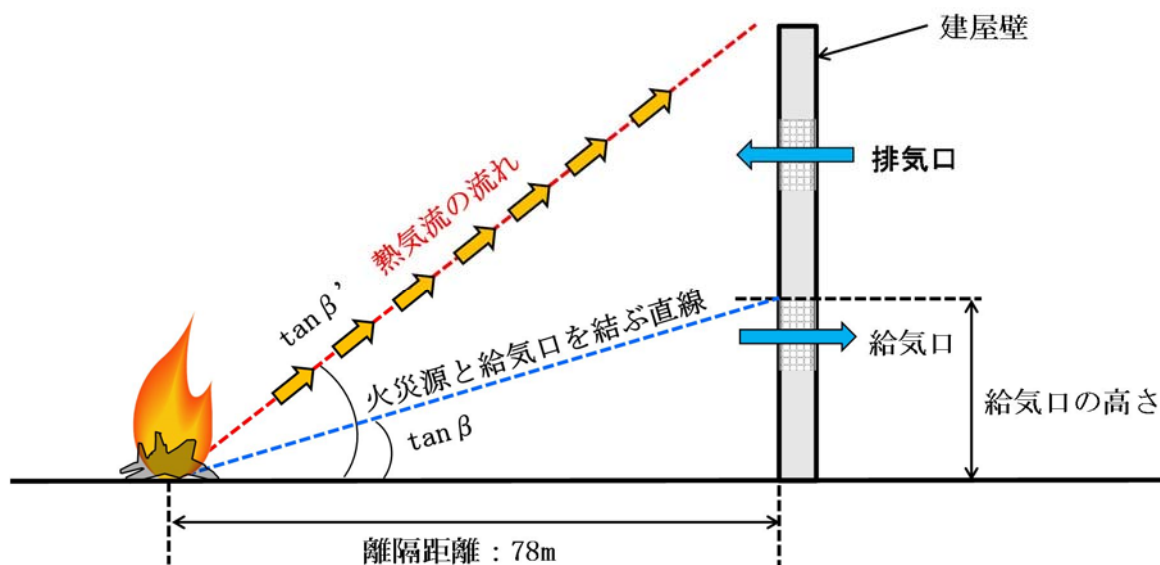
第5.8-1図 使用済燃料乾式貯蔵建屋の評価概念図
