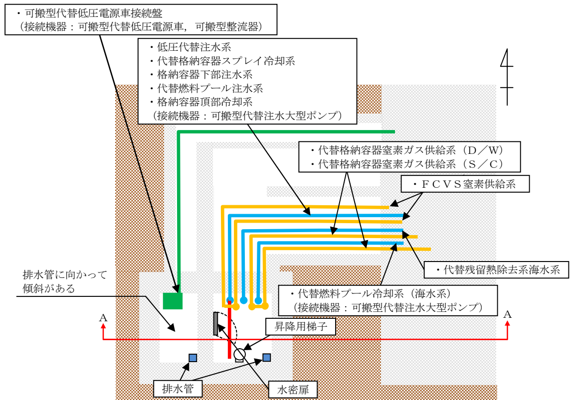
地下格納槽 上面図
