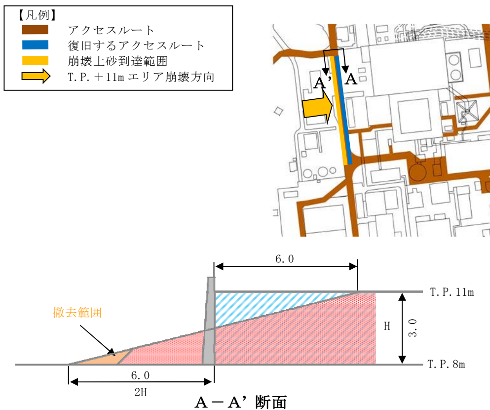
第 5.5.1-5 図 崩壊土砂撤去の考え方
