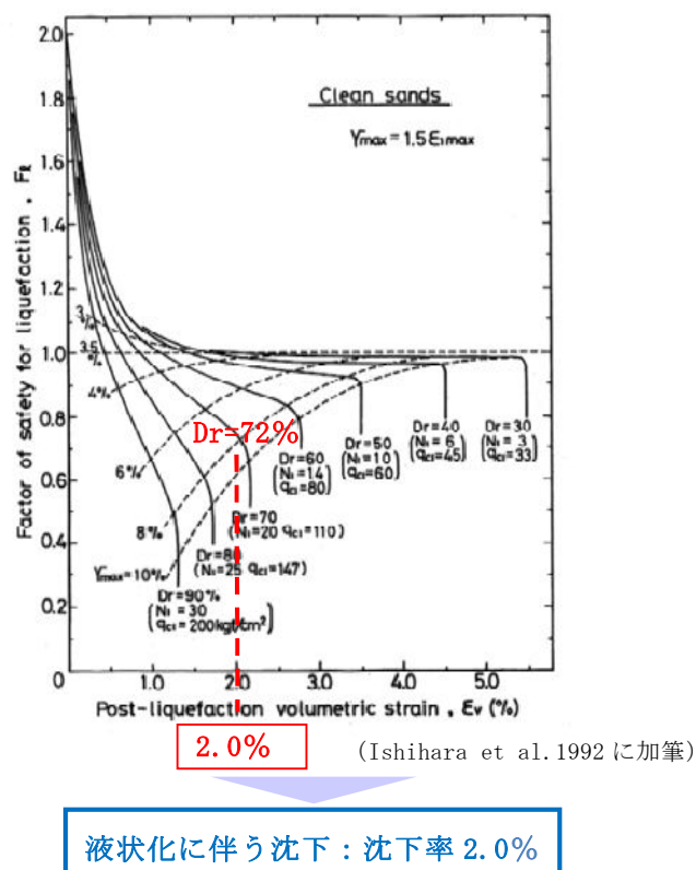
第 4. 3. 3-7 図 体積ひずみと液状化抵抗のj関係及び想定する沈下率 1. 0. 2-67
