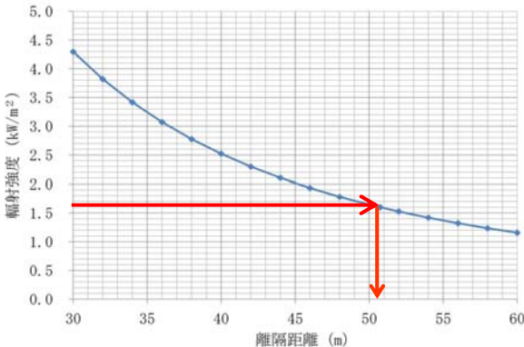
第 1 図 離隔距離と輻射強度の相関図
