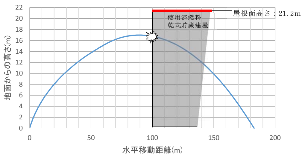
ロ) 鉛直方向の飛跡の例（上図㊸地点からの車両の例）
