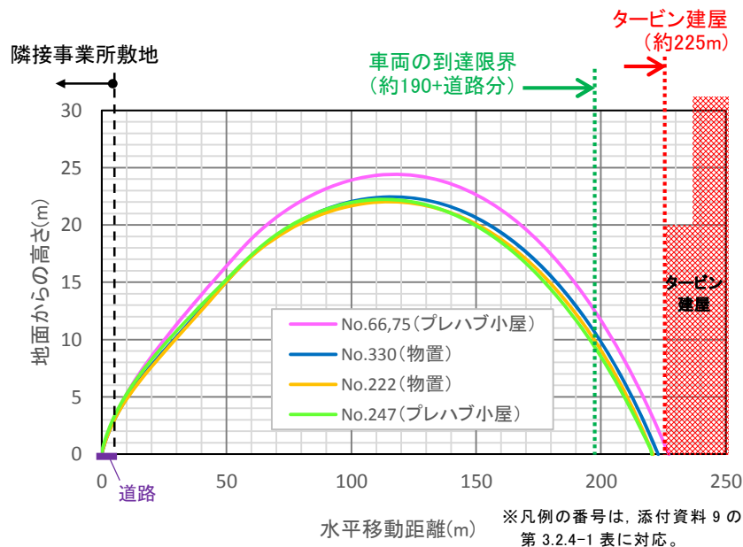
別図 7-1 隣接事業所南端からタービン建屋への飛来物の軌跡
