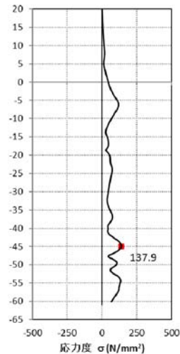
応答変位法解析結果
