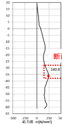
二次元有効応力解析(FLIP)
