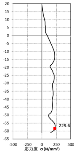
二次元有効応力解析(FLIP)
