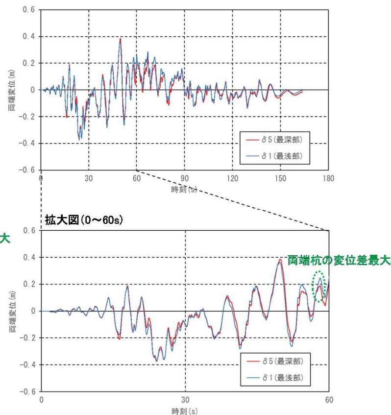
岩盤傾斜部(地点④, 豊浦標準砂を仮定したモデル) 地表面の両端杭位置の変位時刻歴
