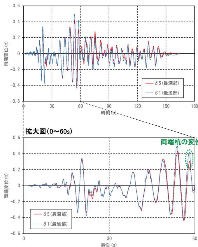
岩盤傾斜部(地点④, 原地盤モデル) 地表面の両端杭位置の変位時刻歴
