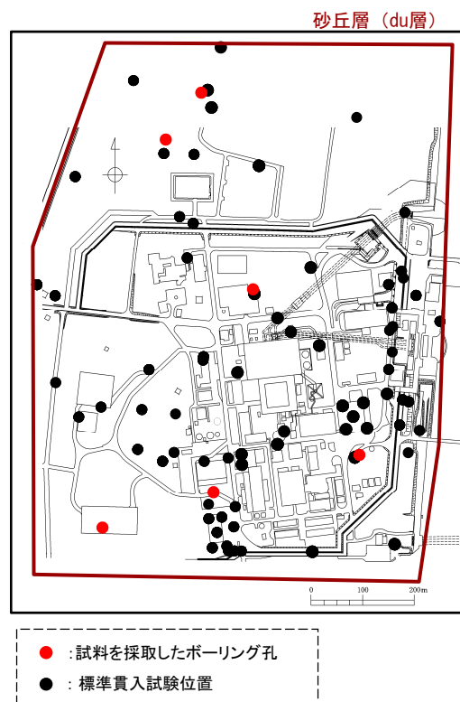
試料採取位置図
