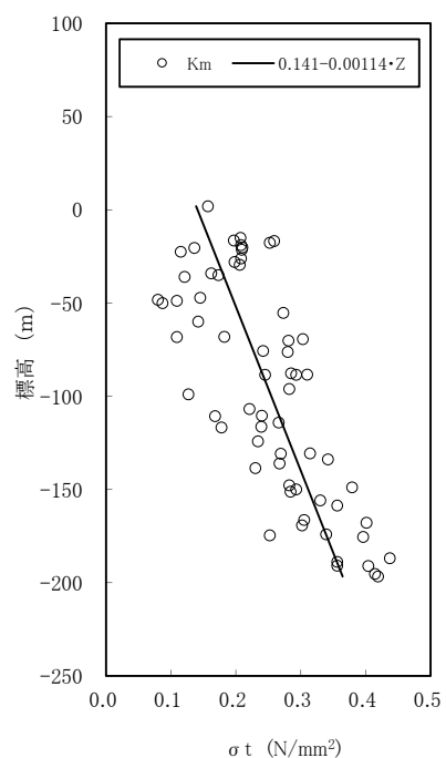
(圧裂試験)
