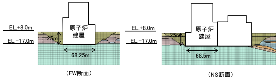
【原子炉建屋】
