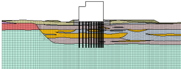
要素分割図
