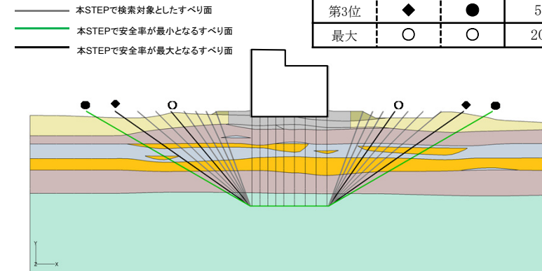
STEP2(角度の検索) (検索範囲内[左30°、右30°]~70°、5° 間隔)
