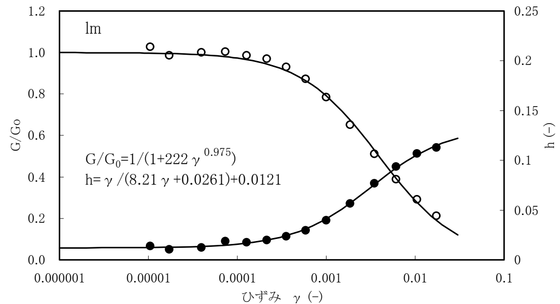
1m層の繰返し三軸試験結果
