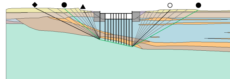
STEP2(角度の検索) (検索範囲内[左25°、右30°]~70°、5° 間隔)
