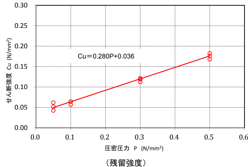
1m層のせん断強度及び残留強度
