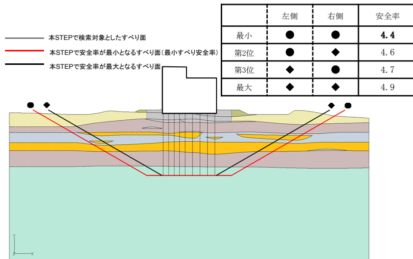
STEP3(水平方向の検索)
