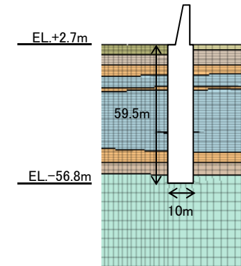
【鉄筋コンクリート防潮壁区画（北側）】
