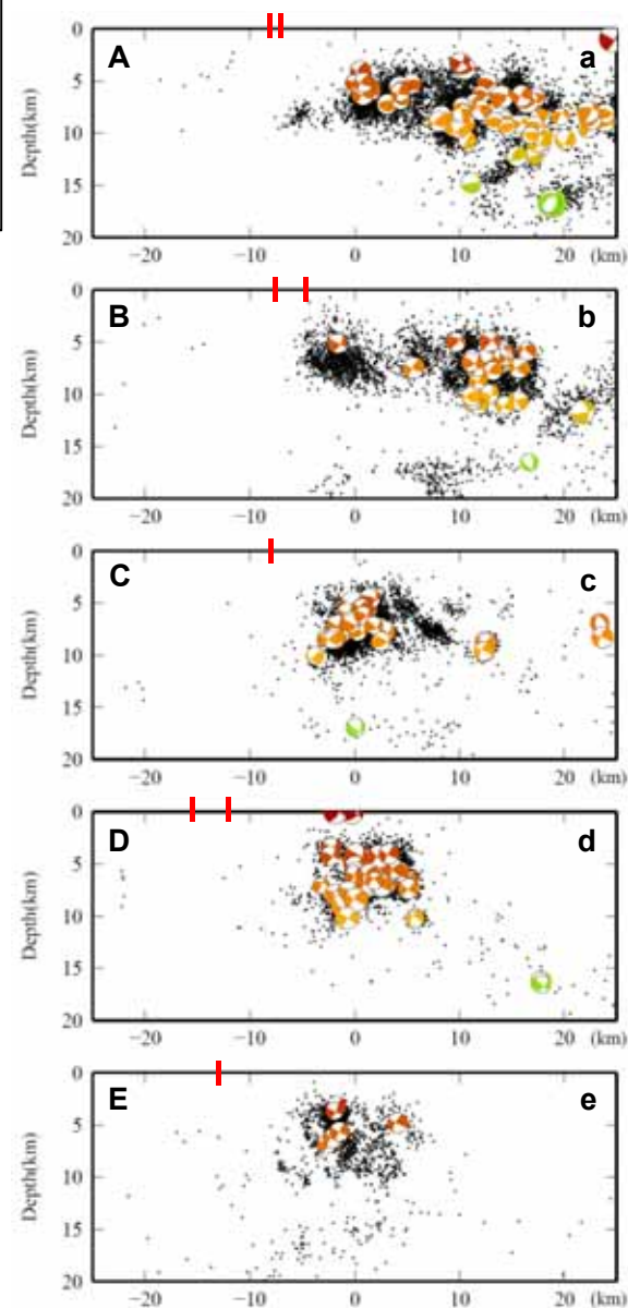
震源断面図 ( は地表での棚倉破砕帯の位置を示す)
