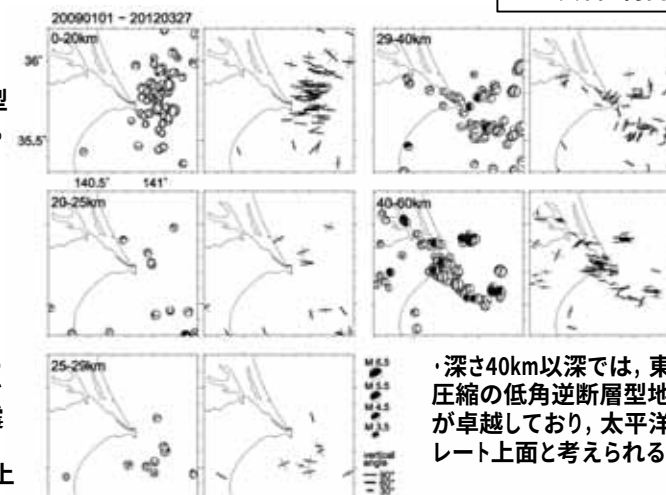
図3 深さ毎のCMT解(VR60%以上、6観測点以上)および地表面に投影した応力軸(T軸:黒、P軸:灰色)の分布。黒シンボルは小緯返し地震を示す。
