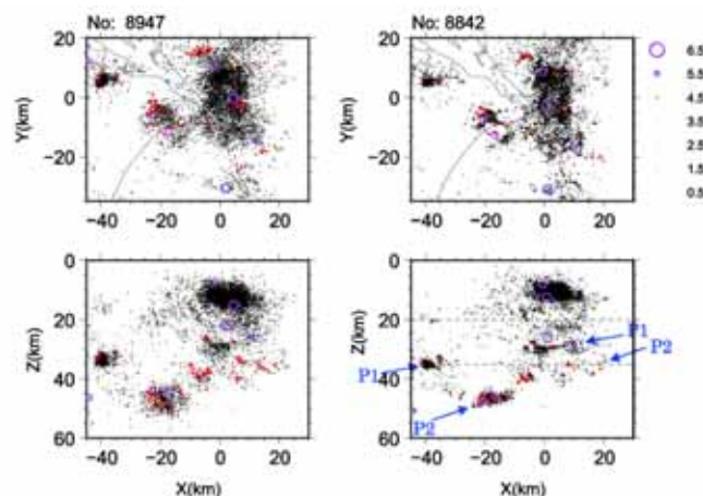
図2 高精度震源決定前後(左:決定前、右:決定後)の震央分布(上段)および鉛直断面図(下段)。図1(P.47)右図の赤線で示した矩形領域について示す。赤丸はM5.5以上の地震を、赤丸は小緯返し地震を示す。
