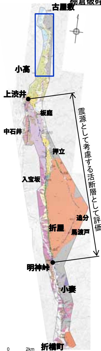
棚倉破砕帯東縁付近の推定活断層
