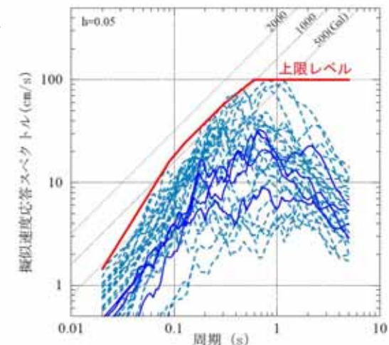
図8 震源を事前に特定できない地震による震源近傍の観測記録の水平応答スペクトルとその上限レベル (実線は 1997 年鹿児島県北西部地震の鶴田ダムのスペクトル、破線はスケリングの観点から確実に事前に震源を特定できるとは断定できないと判断した M_j6.5(M_w6.2) 以下の7地震のスペクトル)
