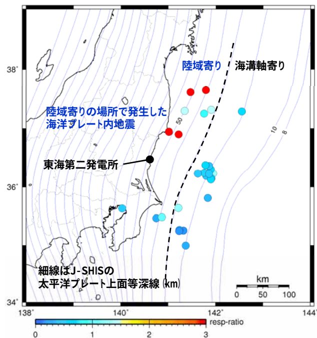
検討対象地震の震央分布 (海洋プレート内地震) (水平成分)
