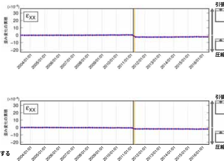
ひずみ変化の累積 (東海第二発電所敷地周辺)
