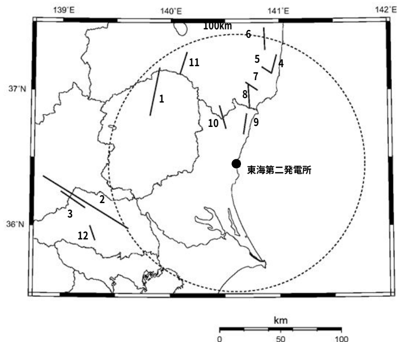
活断層分布 (推本参考モデル)
