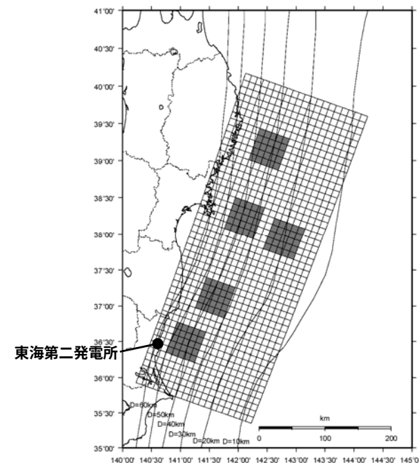
2011年東北地方太平洋沖型の地震の震源モデル
