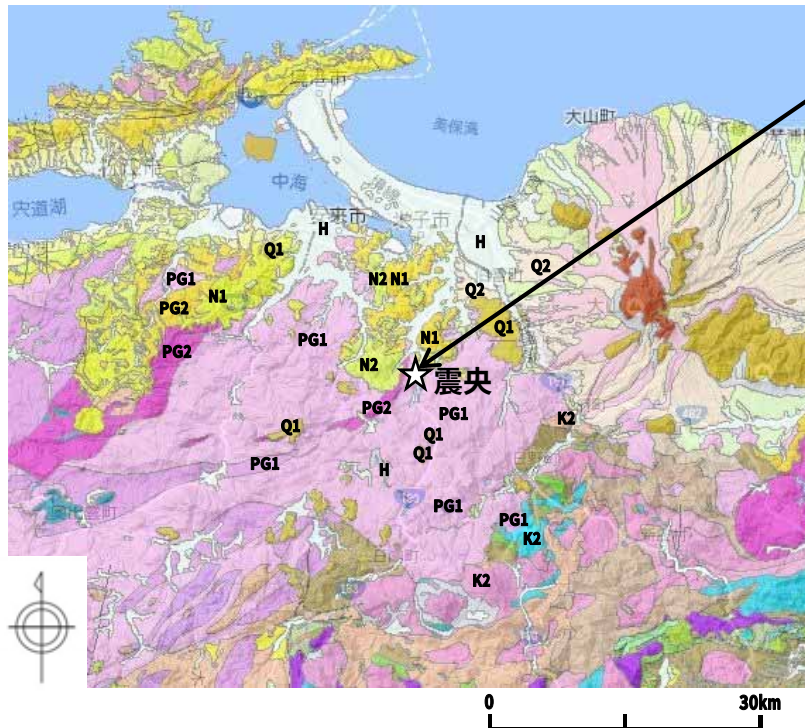
震源域周辺のシームレス地質図 (産業技術総合研究所, 地質図Naviに加筆)
