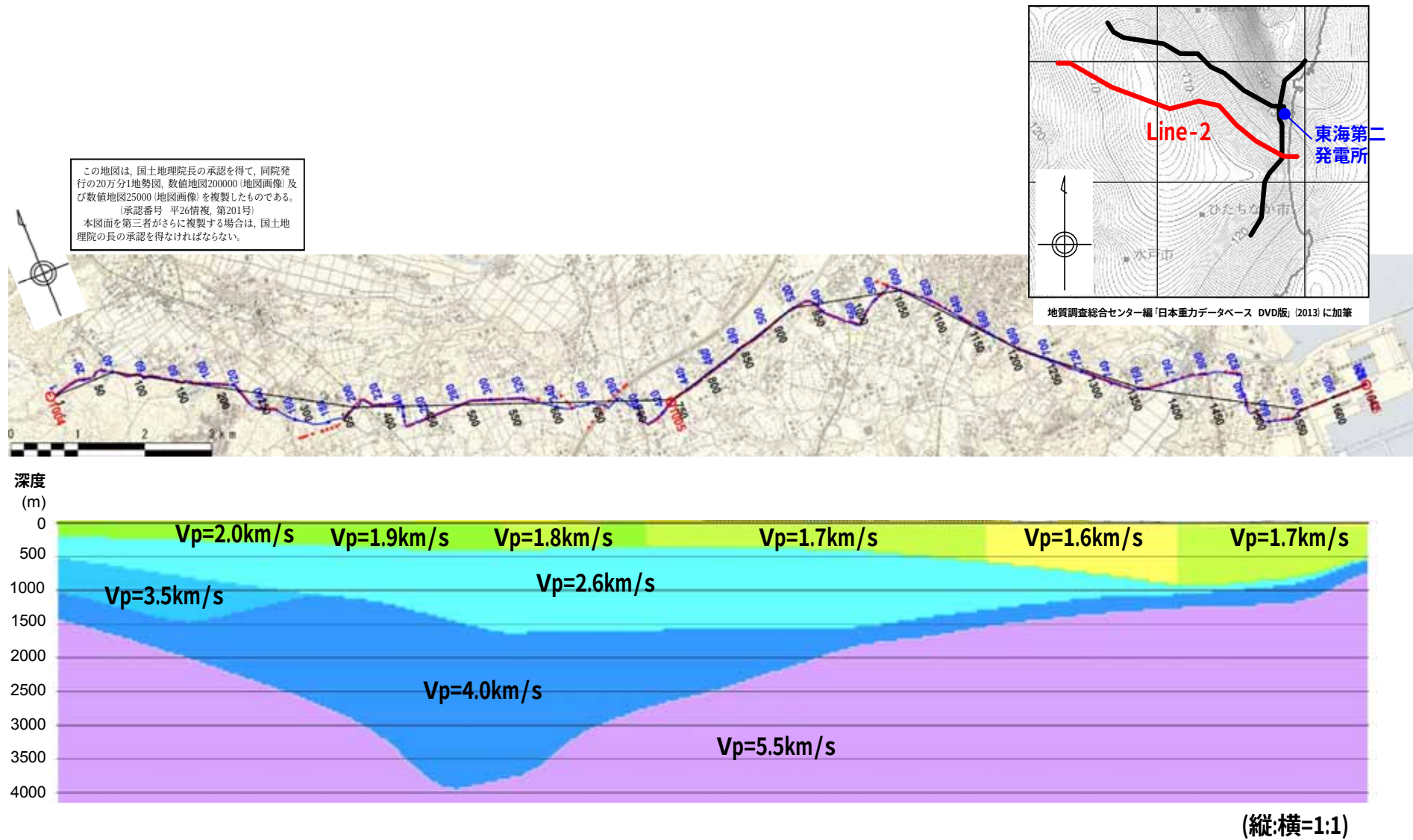
屈折法地震探査によるP波速度構造
