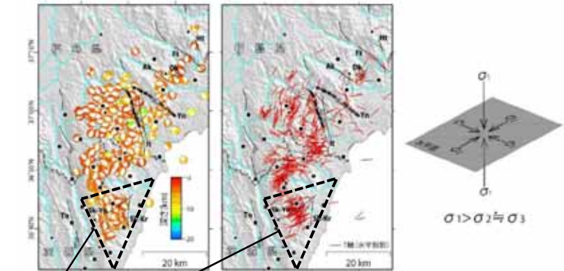
図 11 得られたメカニズム解と主軸の分布
