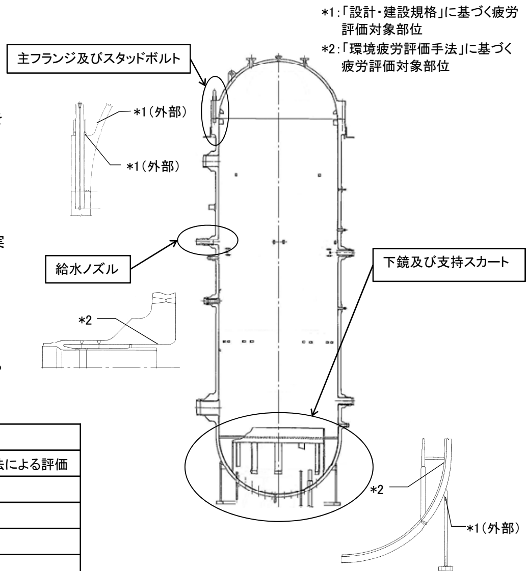
原子炉圧力容器の疲労評価結果
