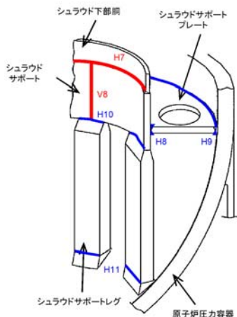
炉心シュラウド概略図
