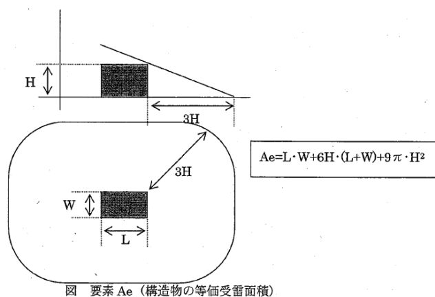
図 要素 A_e (構造物の等価受雷面積)
