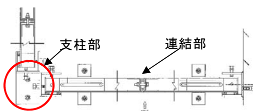
支柱レールの取付状況
