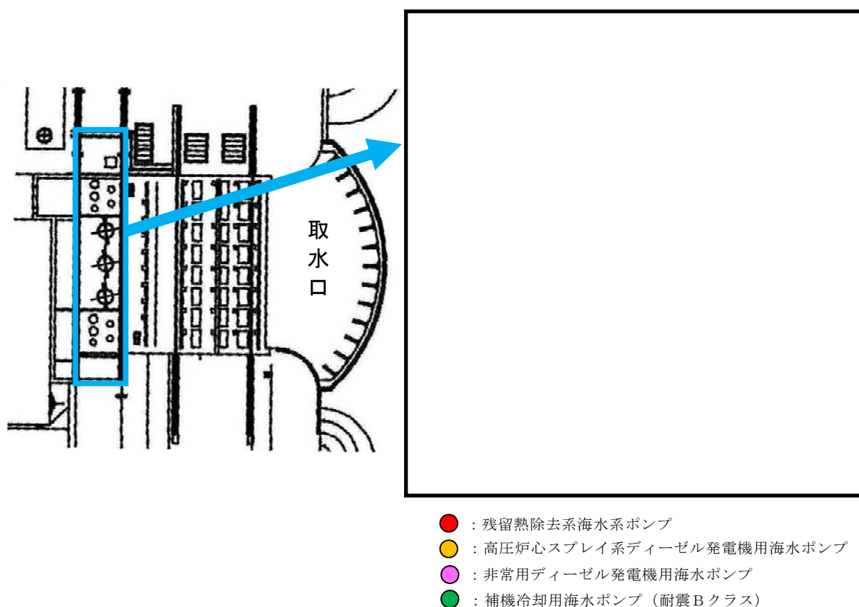
第 10-1 図 海水ポンプエリア平面図
