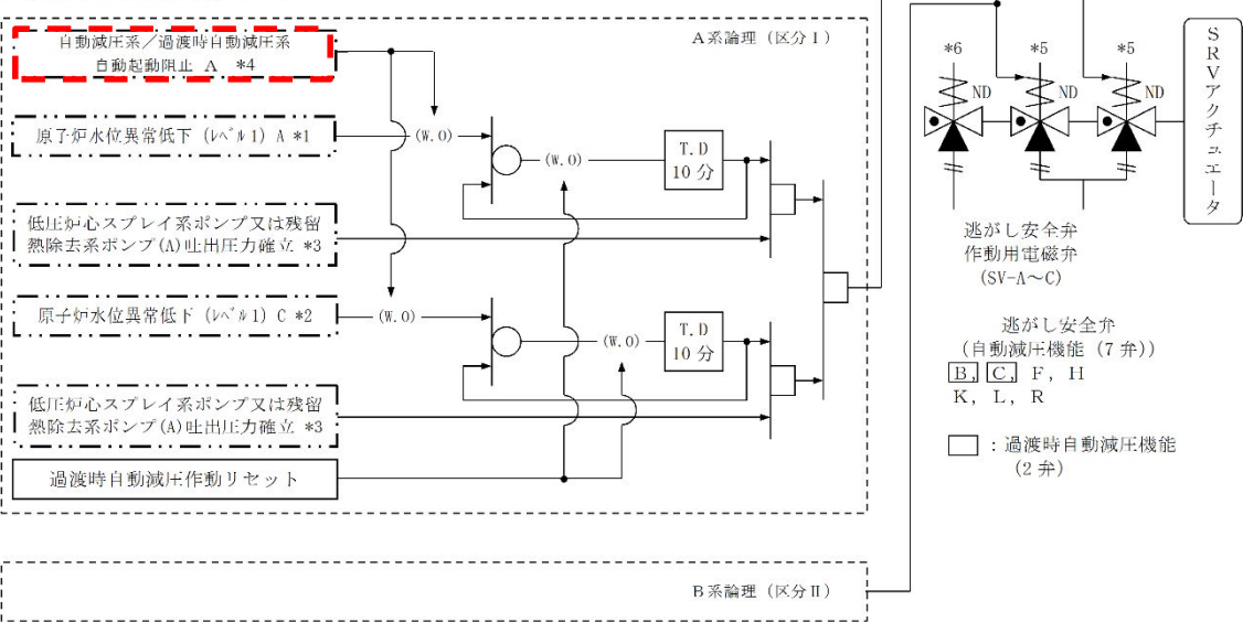
過渡時自動減圧機能論理回路
