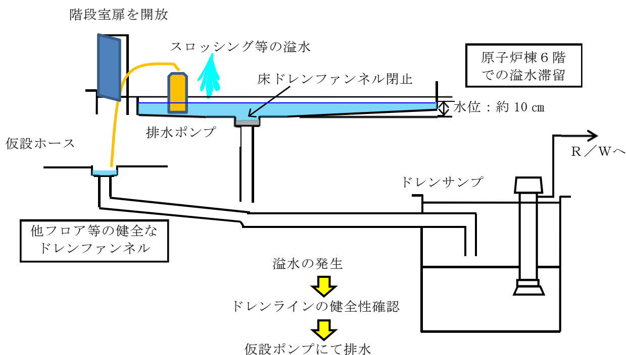
第 9 図 停止時の床ドレンファンネル閉止・堰の排水切欠き閉塞時における排水処理について
