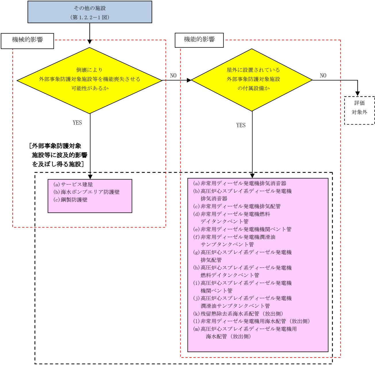
第 1. 2. 2-4 図 外部事象防護対象施設等に波及的影響を及ぼし得る施設 の抽出フロー
