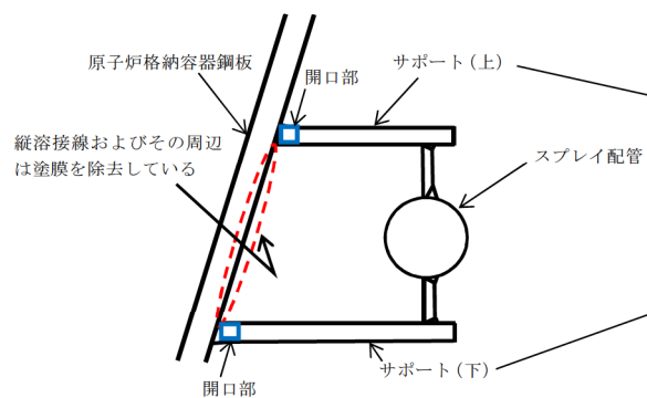
サポート断面概要図（イメージ図）
