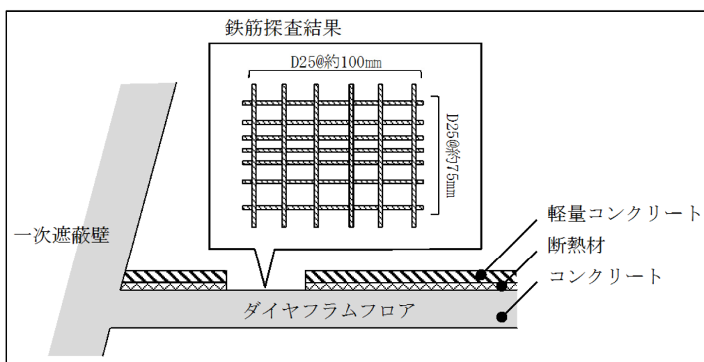
図 4. 1. 1-2 ダイヤフラムフロア概要図
