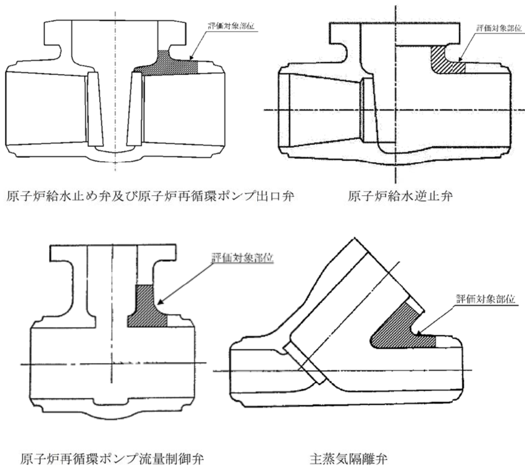
図 6-4 弁評価対象部位
