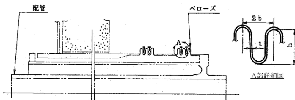
図 6-6 機械ペネトレーション（配管貫通部 ベローズ式）の形状
