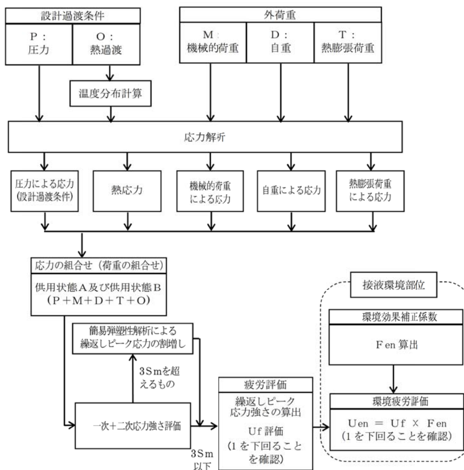
図3 疲労評価における応力解析の流れ (原子炉圧力容器のうちスタッドボルト以外，炉内構造物)
