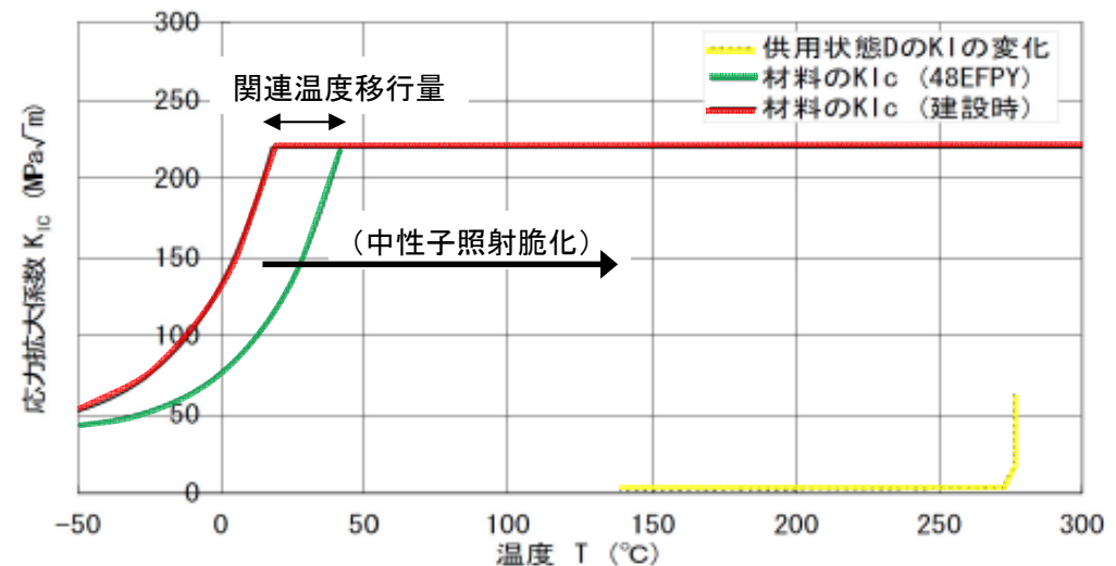
供用状態Dにおける原子炉圧力容器の加圧熱衝撃評価(BWR-5)
