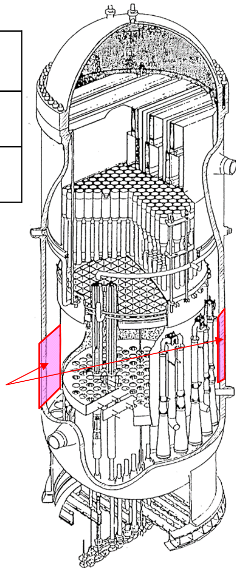
原子炉压力容器
