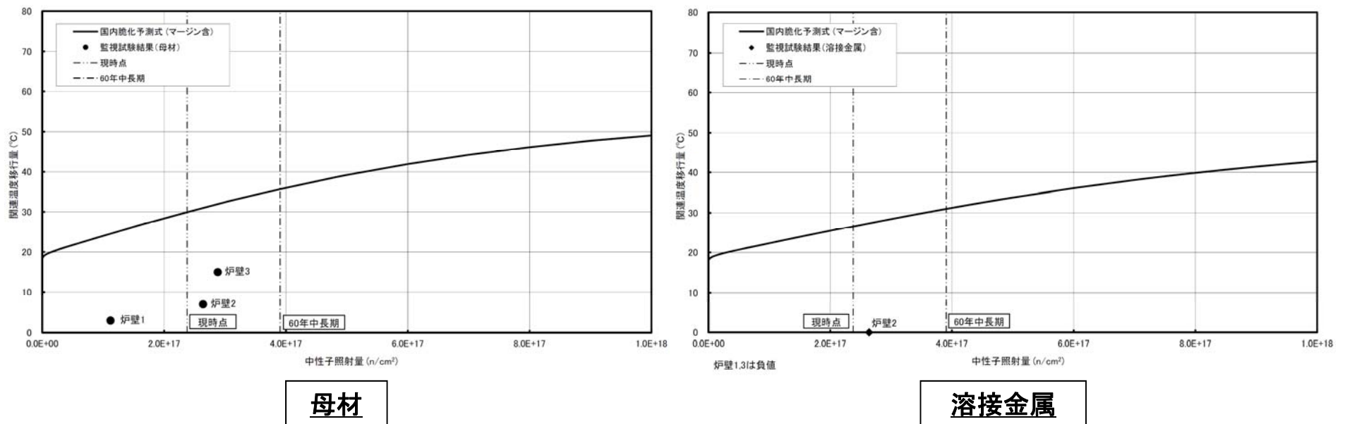
原子炉圧力容器胴部(炉心領域部)の中性子照射脆化に対する関連温度の 国内脆化予測法による予測と監視試験結果の関係
