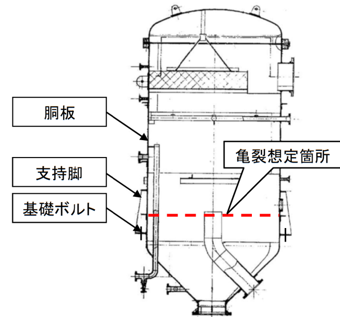
廃液濃縮器蒸発缶構造図
