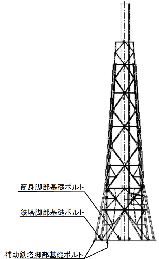
主排気筒概要図
