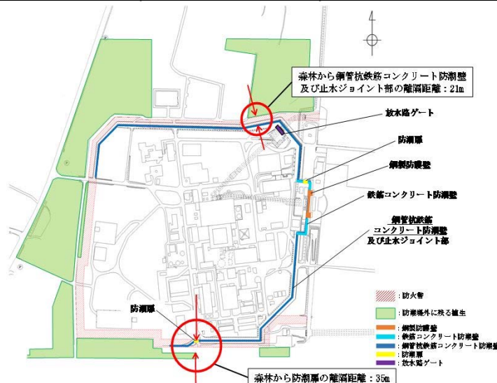
津波防護施設と森林との位置関係
