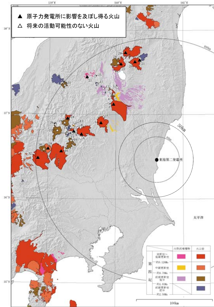
火山地質図
