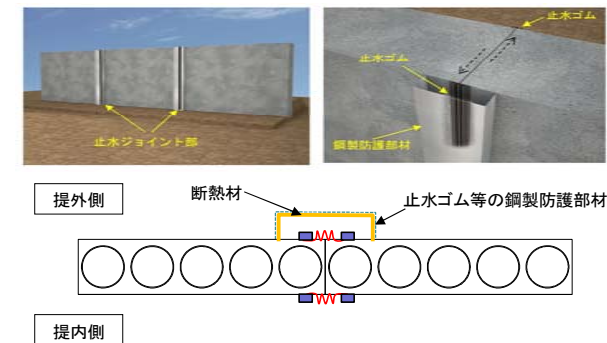
止水ジョイント部の概要図
