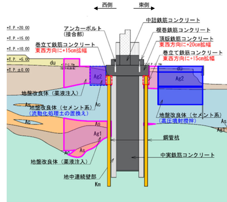
構造変更後 南基礎断面図
