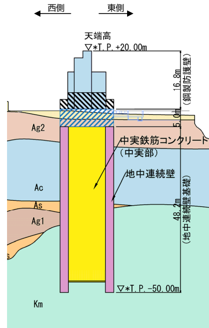
既工認 南基礎断面図
