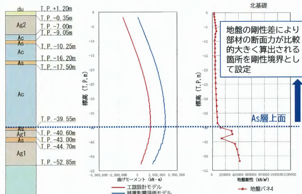
中実鉄筋コンクリートの堤軸直交方向 曲げモーメント図
