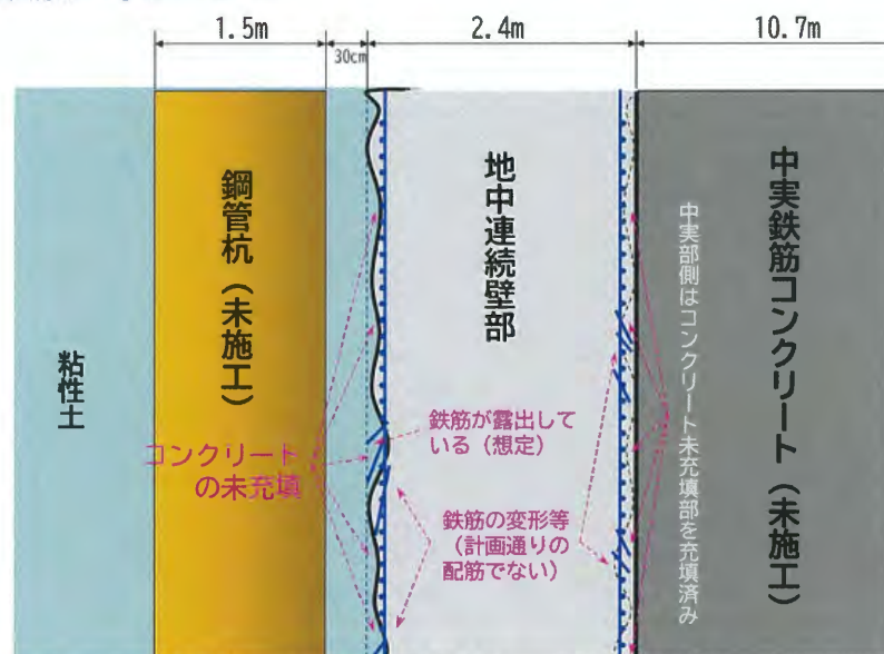
現状の不具合状況イメージ図
