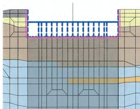
b-b断面
