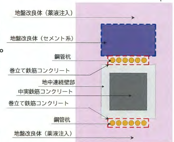
北基礎平面拡大図 （追加基礎＋地盤改良）
