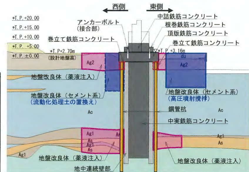
北基礎断面図
