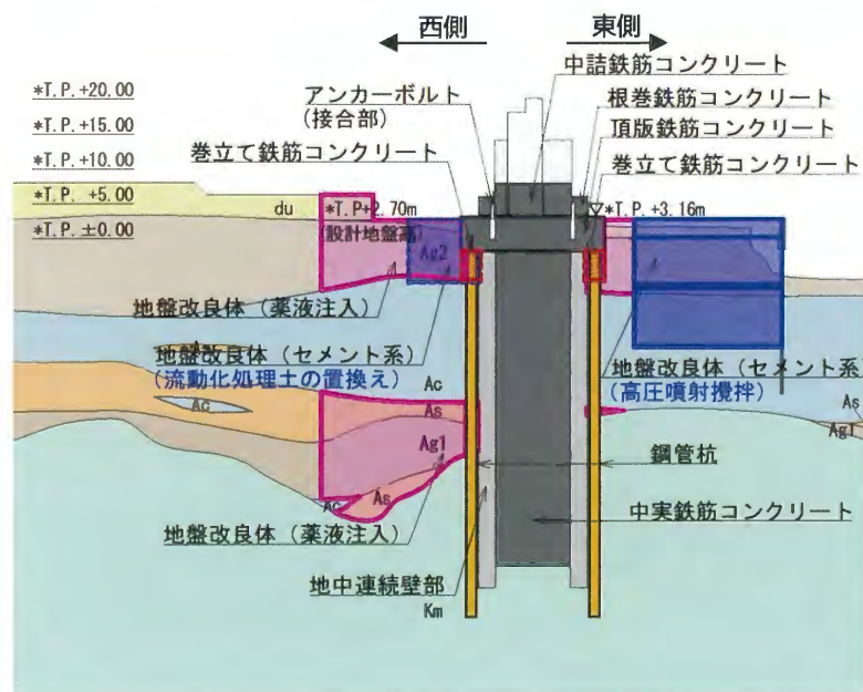
(b)-(b)断面図
