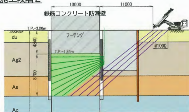
構造物直下の地盤改良の施工方法の例
