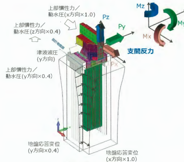
荷重モデル
