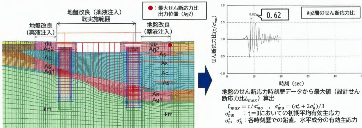
最大せん断応力比の抽出
