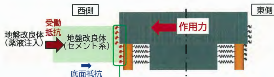
断面図
