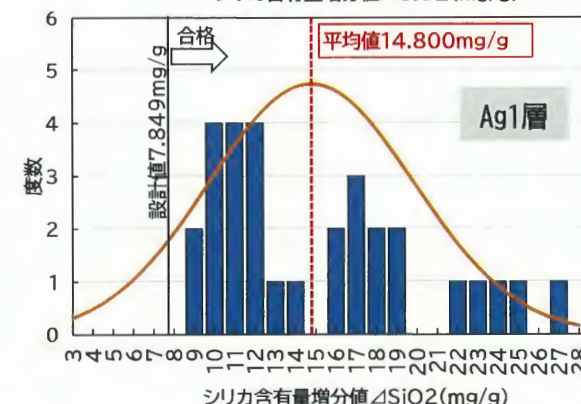
既施工箇所のシリカ含有量増分値測定結果
