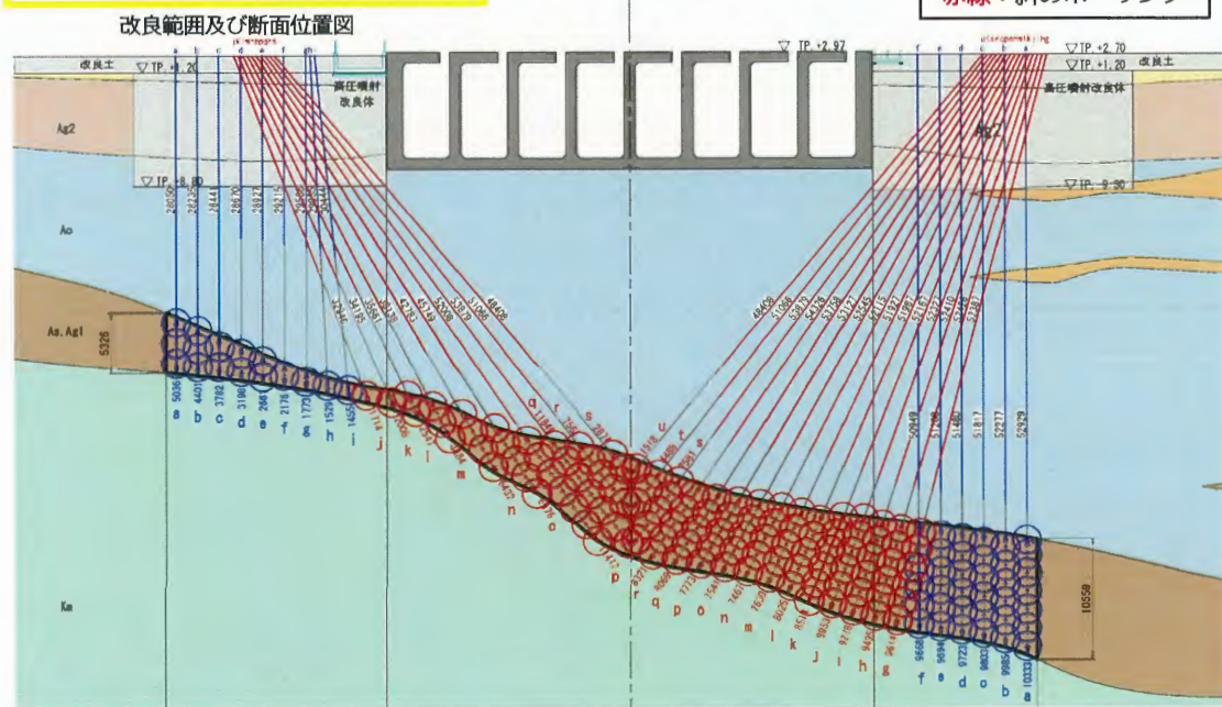
地盤改良（薬液注入）の配置
