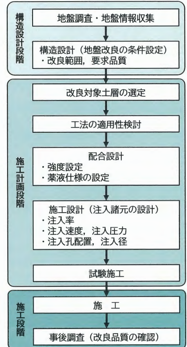
地盤改良（薬液注入）設計フロー
