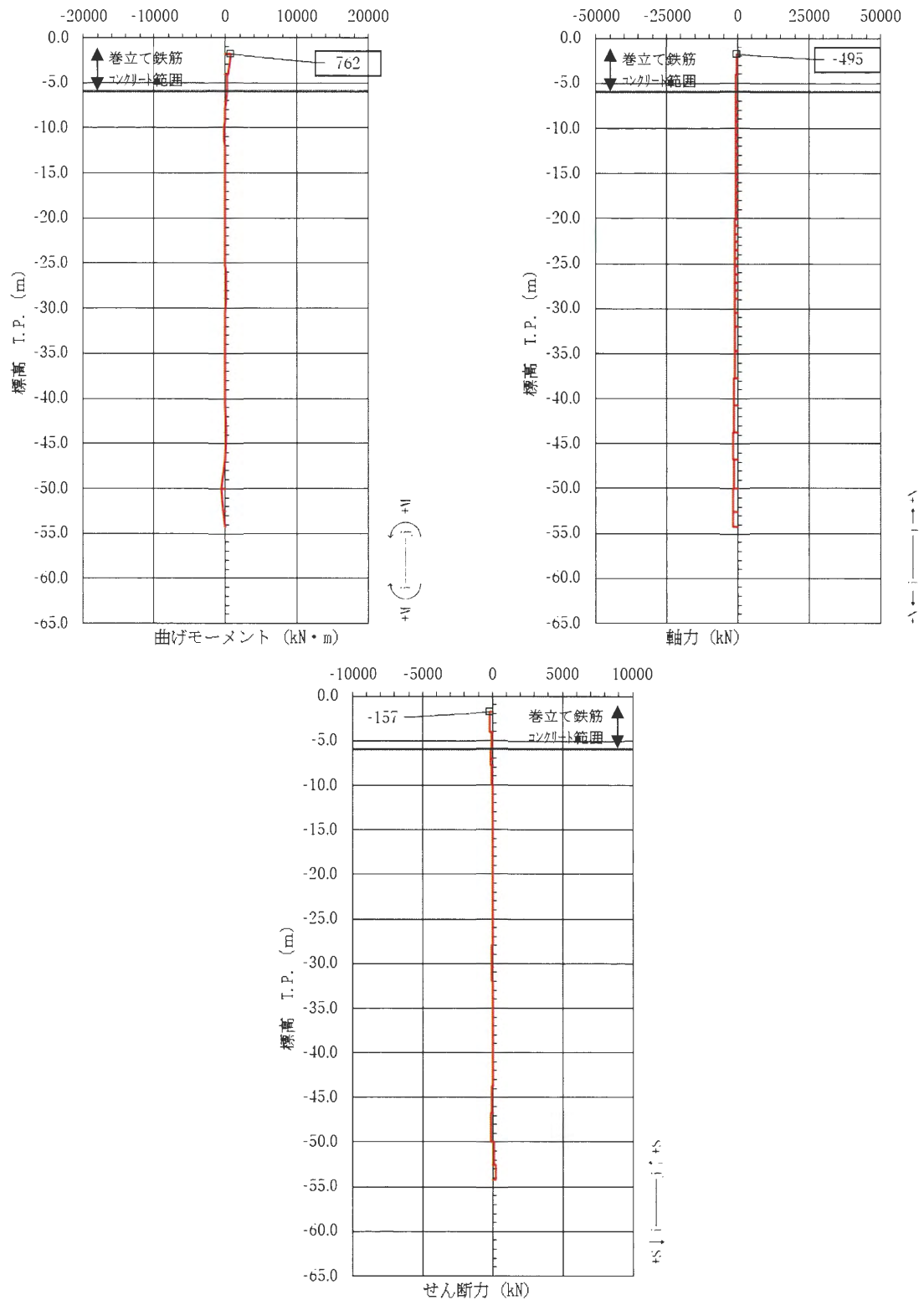
図 3.2-48 巻立て鉄筋コンクリート内の鋼管杭の曲げ軸力照査 (引張) が最も厳しい時刻の断面力図 (①-①断面, 南基礎 端部) ( S_s - 3.1 [H+, V+] t = 9.13 s) (地盤ケース③: 地盤物性のばらつきを考慮 ( -1\sigma ) した解析ケース)
