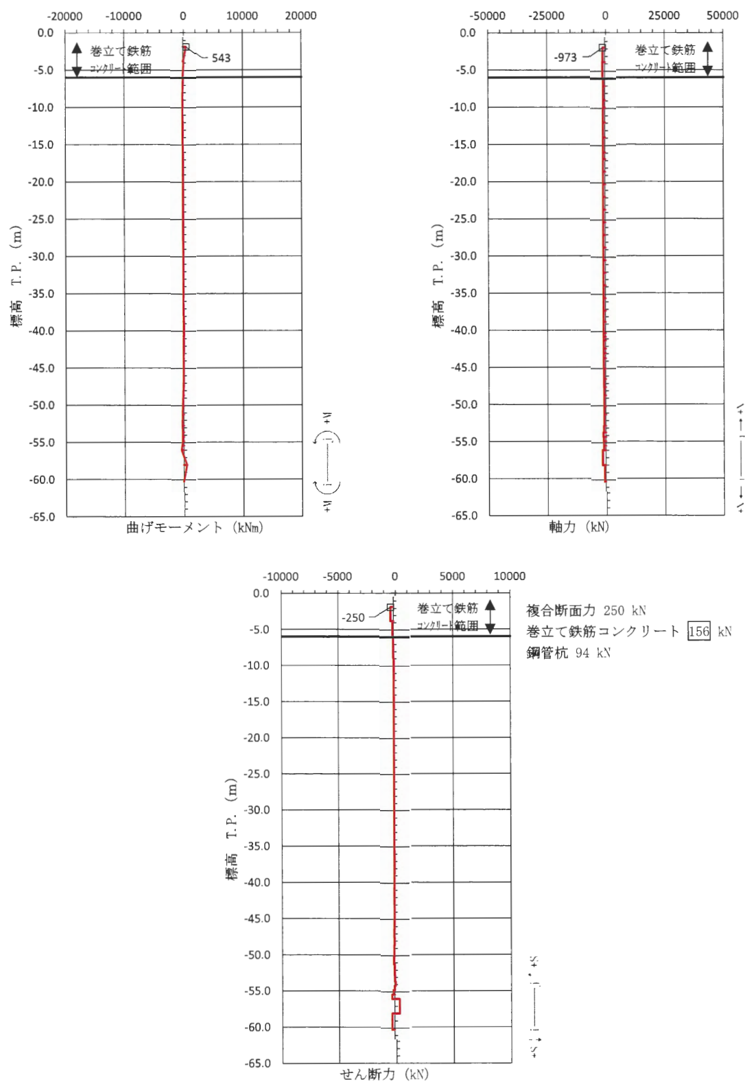
図 3.2-42 鉄筋コンクリートのせん断照査が最も厳しい時刻の断面力図 (①-①断面, 北基礎 端部)
