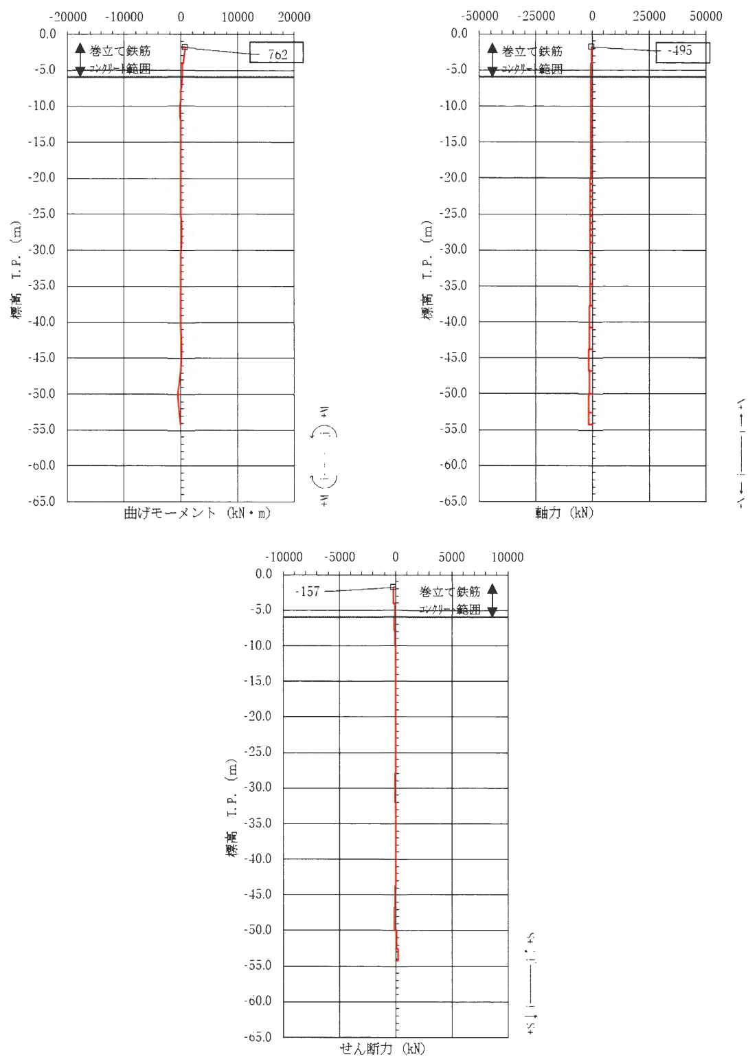
図 3.2-67 鉄筋の曲げ軸力照査が最も厳しい時刻の断面力図 (①-①断面, 南基礎 端部)
