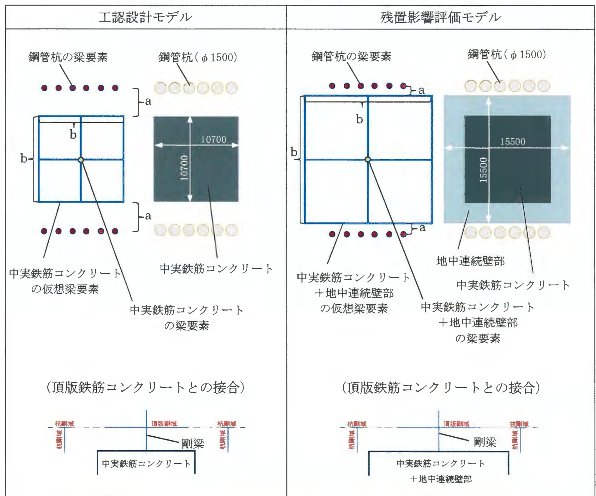
A-A断面
