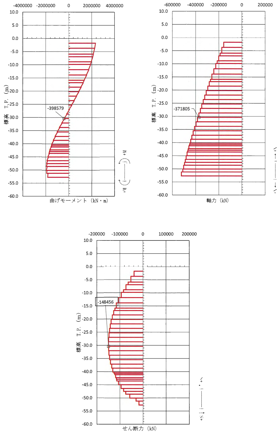
図 3.2-12 鉄筋コンクリートのせん断照査が最も厳しい時刻の断面力図 (①-①断面, 北基礎)
