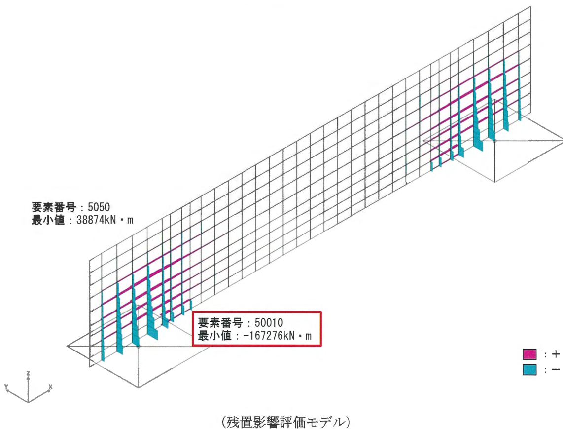
図 3.2-95 主部材の最大断面力分布図 (ねじりモーメントTQ)
