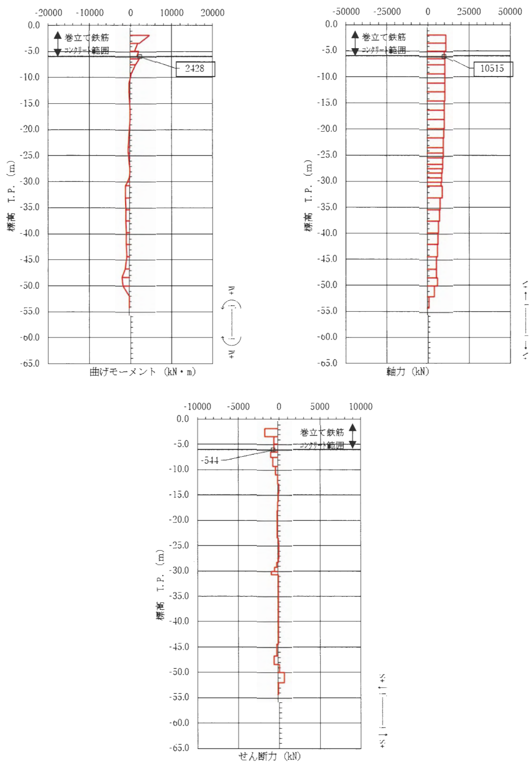
図 3.2-21 鋼管杭の曲げ軸力照査 (引張) が最も厳しい時刻の断面力図 (③-③断面, 南基礎)
