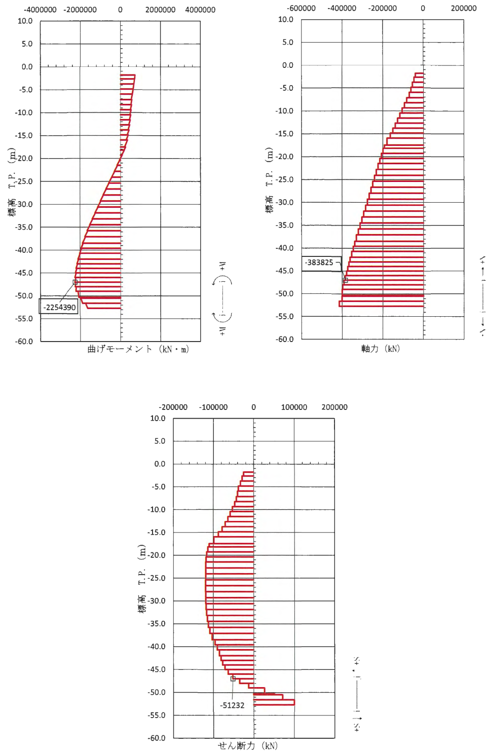
図 3.2-8 コンクリートの曲げ軸力照査が最も厳しい時刻の断面力図 (②-②断面, 北基礎) (S_s - 3.1 [H+, V+] \quad t = 8.93 \text{ s}) (地盤ケース③: 地盤物性のばらつきを考慮 ( -1\sigma ) した解析ケース)
