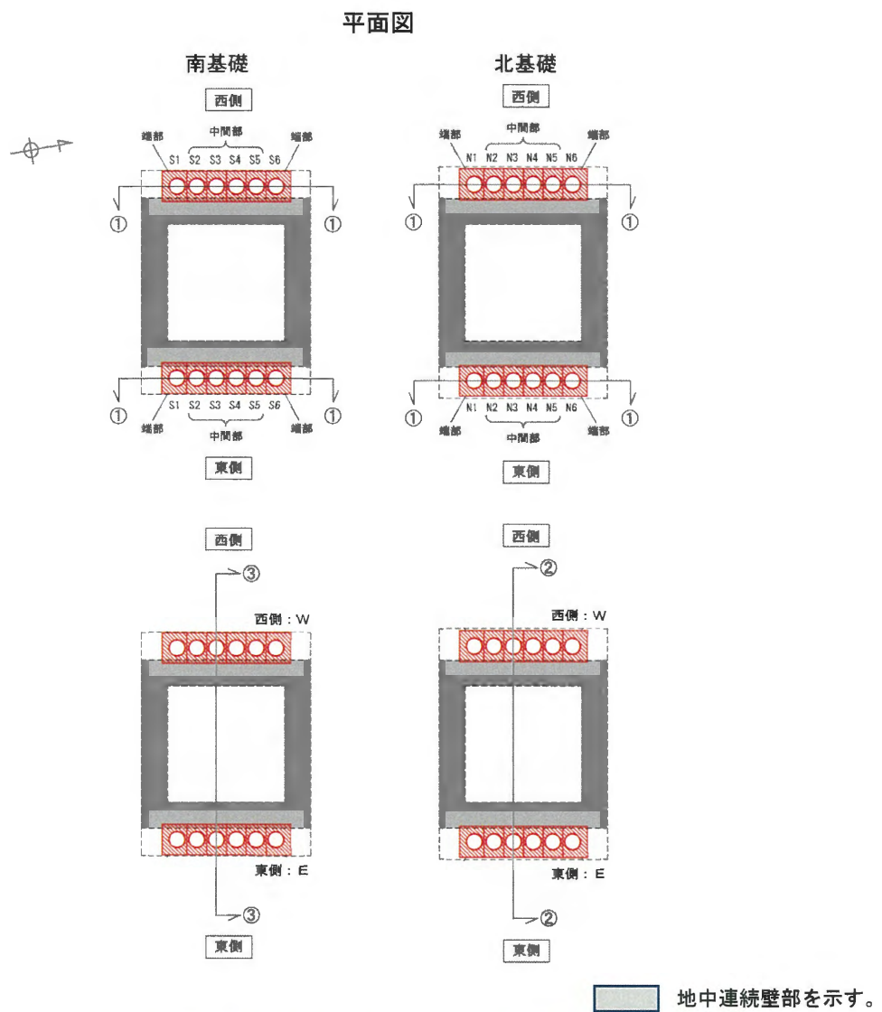
図 3.2-29 評価位置及び杭記号位置図（巻立て鉄筋コンクリート）
