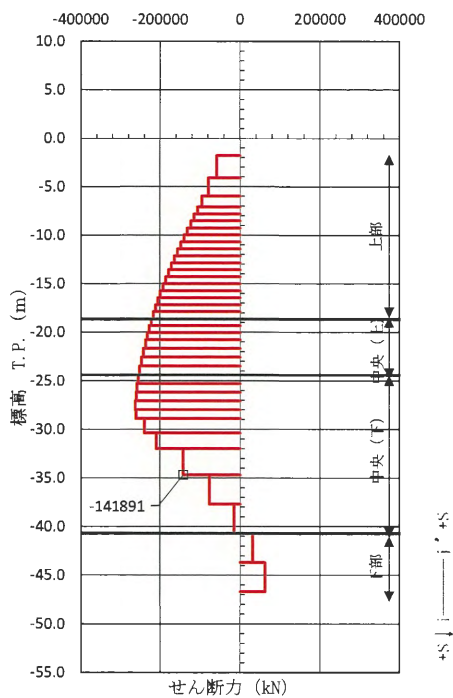
図 3.2-3 鉄筋の曲げ軸力照査が最も厳しい時刻の断面力図 (①-①断面, 南基礎 中央 (下)) (S_s - 31 [H+, V+] t = 8.84 \text{ s}) (地盤ケース④: 敷地に存在しない豊浦標準砂の液状化強度特性により 地盤を強制的に液状化させることを仮定した解析ケース)
