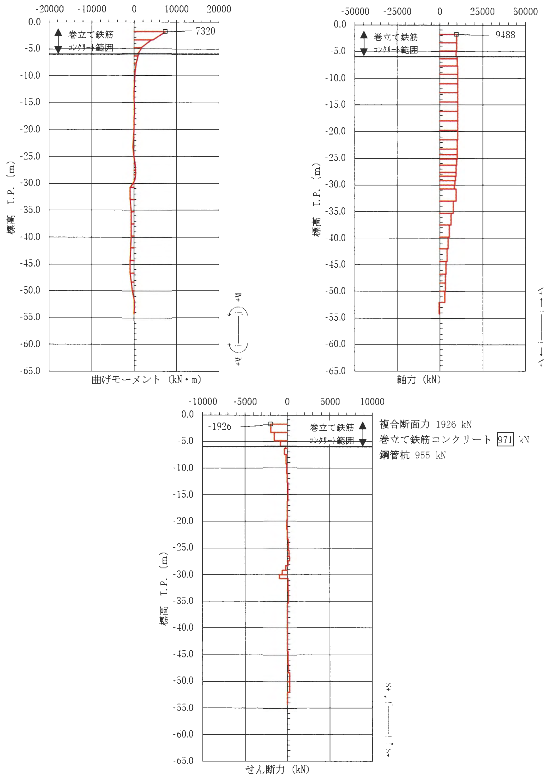
図 3.2-43 鉄筋コンクリートのせん断照査が最も厳しい時刻の断面力図 (③-③断面, 南基礎 西側) (S s-D 1 [H-, V-] t=23.10 s)
