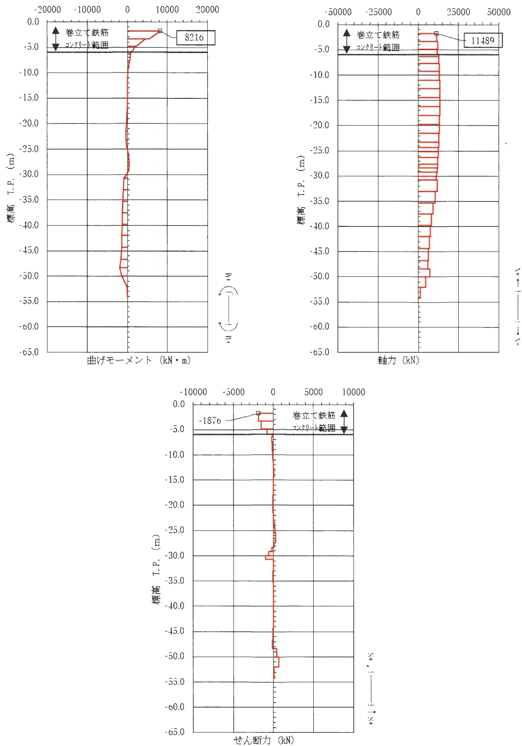
図 3.2-37 鉄筋の曲げ軸力照査が最も厳しい時刻の断面力図 (③-③断面, 南基礎 西側) ( S_s-D1 [H-, V-] t=26.96 s)
