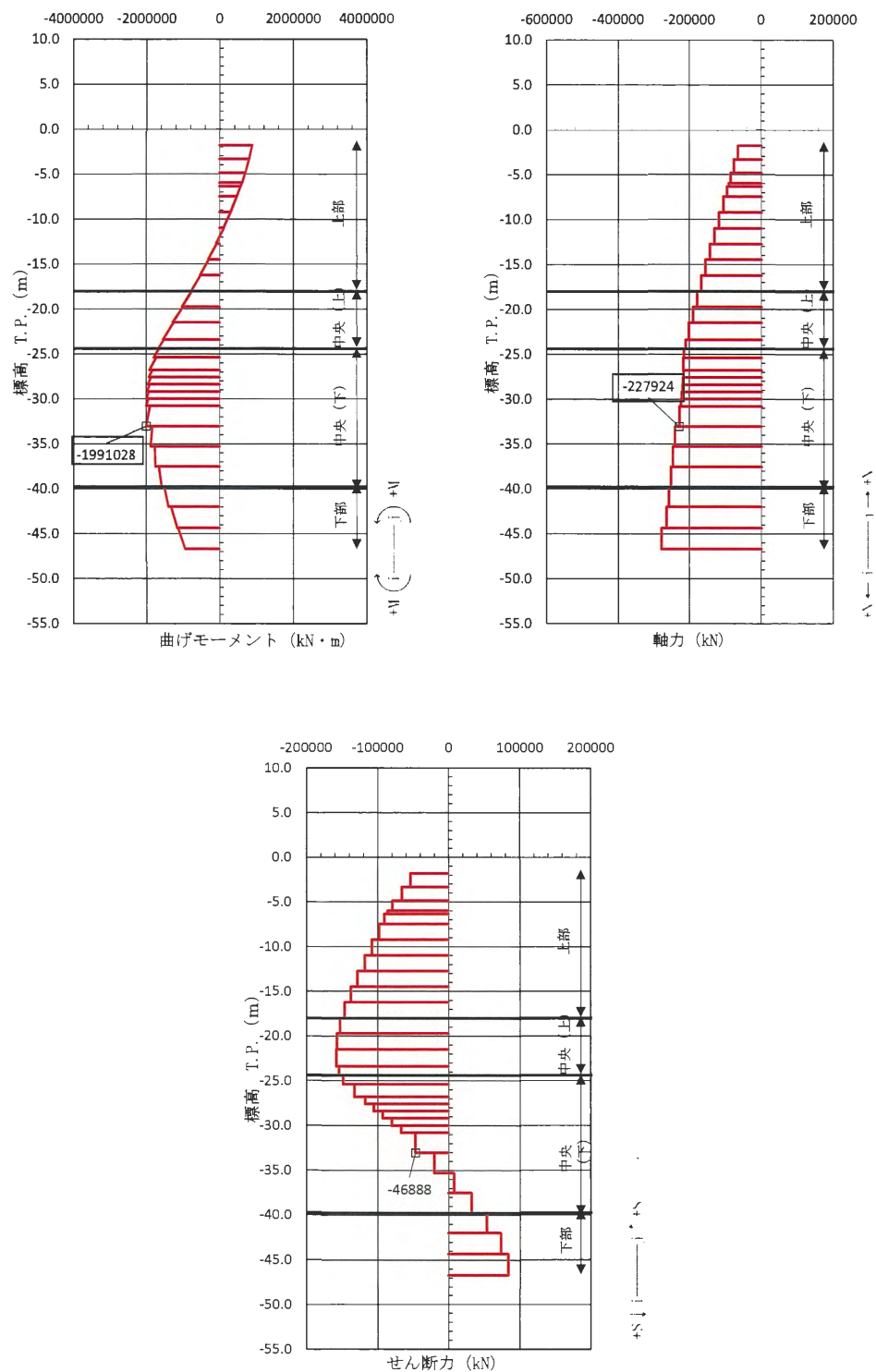
図 3.2-6 コンクリートの曲げ軸力照査が最も厳しい時刻の断面力図 (③-③断面, 南基礎 中央 (下))
