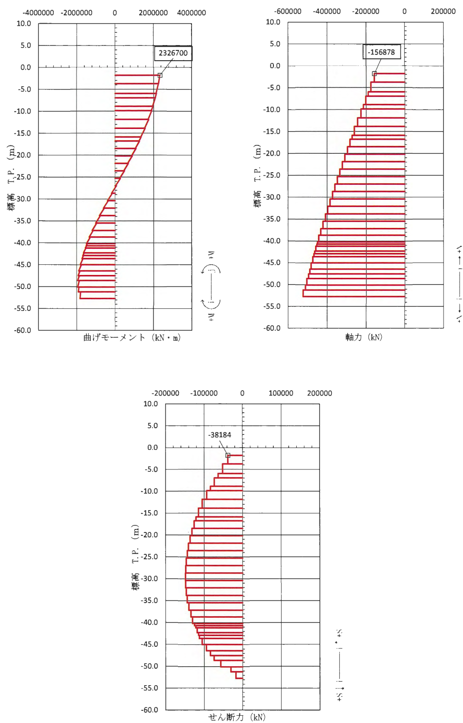
図 3.2-5 鉄筋の曲げ軸力照査が最も厳しい時刻の断面力図 (①-①断面, 北基礎)
