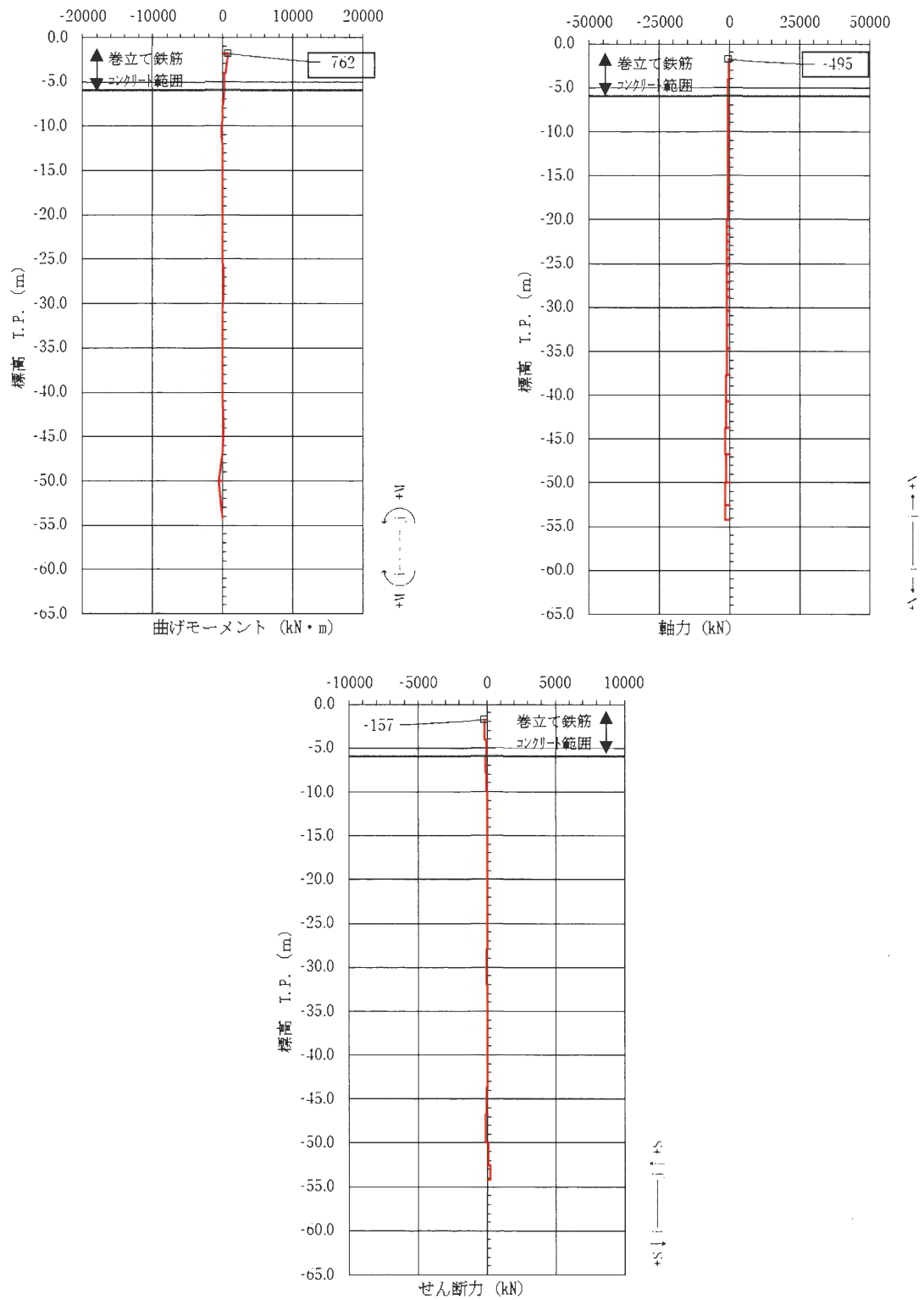
図 3.2-35 鉄筋の曲げ軸力照査が最も厳しい時刻の断面力図 (①-①断面, 南基礎 端部) (S s -3 1 [H+, V+] t=9.13 s) (地盤ケース③: 地盤物性のばらつきを考慮 (-1σ) した解析ケース)
