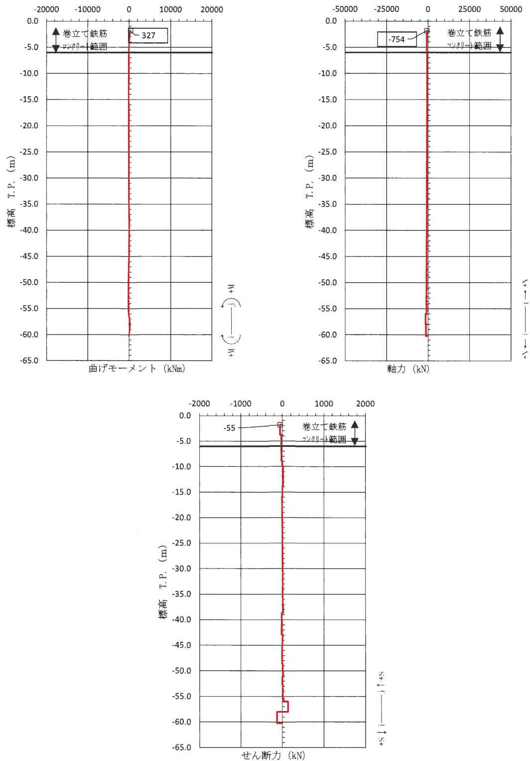
図 3.2-78 鉄筋の曲げ軸力照査が最も厳しい時刻の断面力図 (①-①断面, 北基礎 中間部) (S_s - 3.1 [H+, V+] t = 9.65 \text{ s}) (地盤ケース③: 地盤物性のばらつきを考慮 ( -1\sigma ) した解析ケース)
