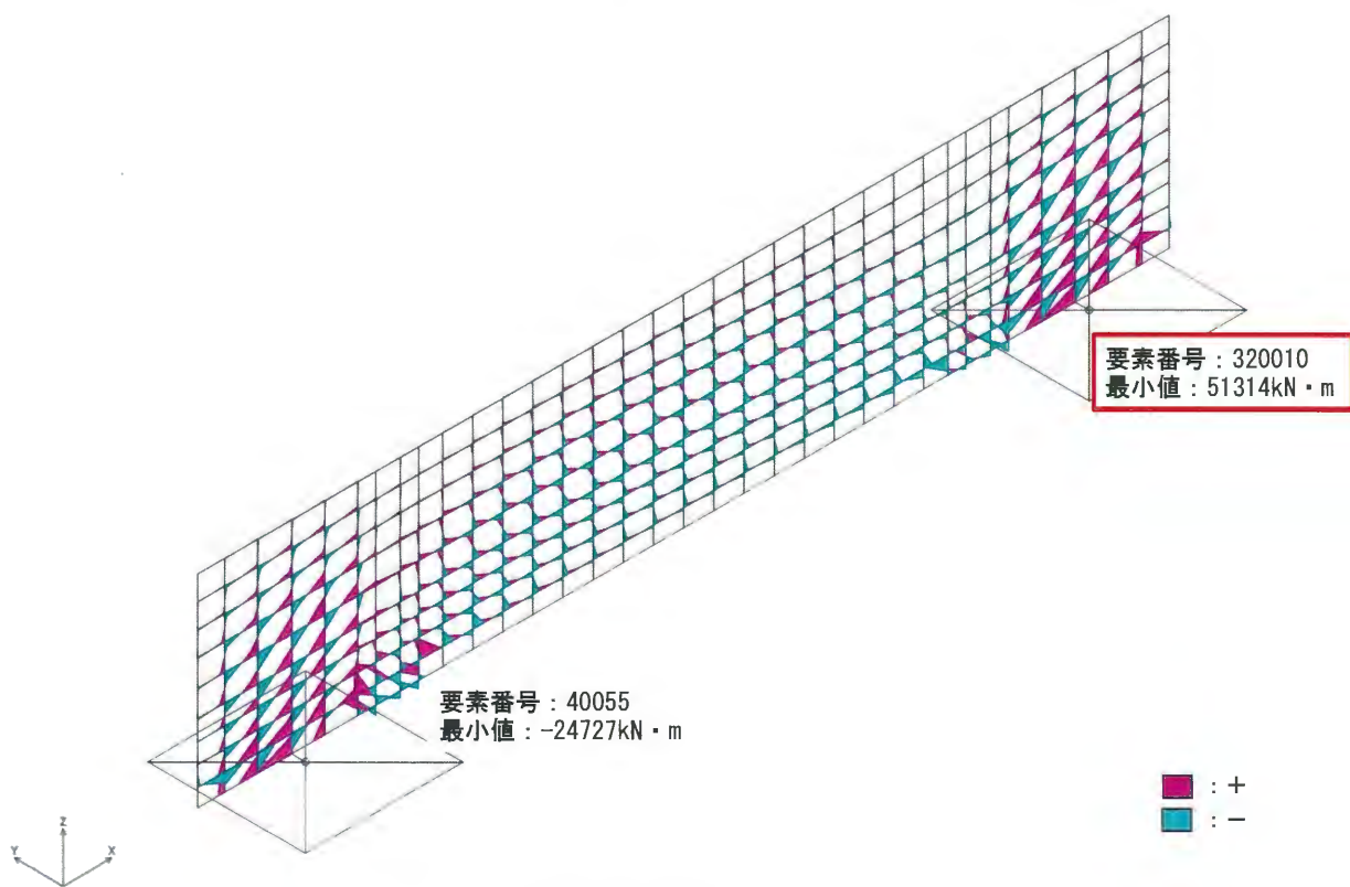
図 3.2-91 主部材の最大断面力分布図 (面内曲げモーメントM2)
