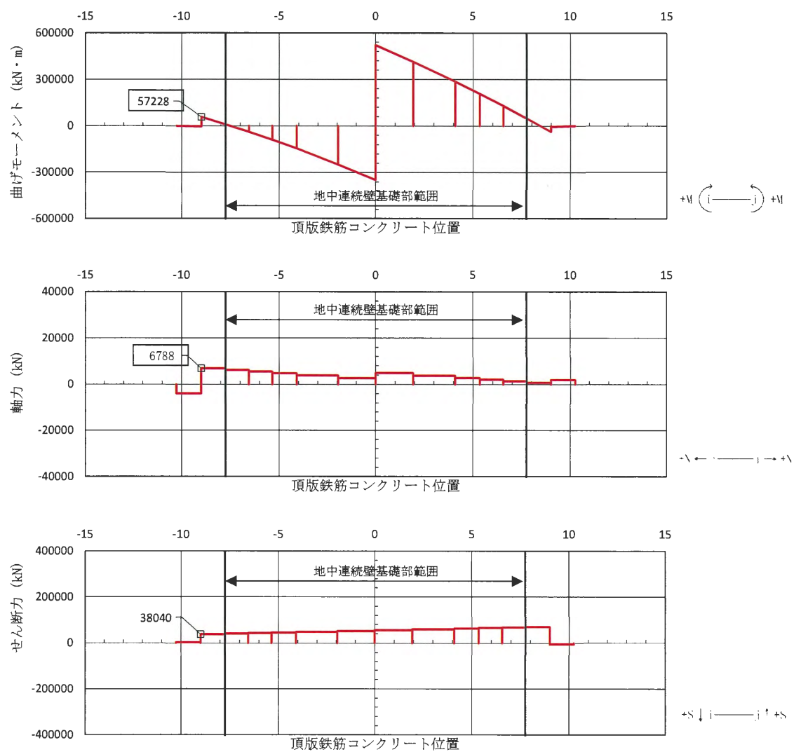
図 3.2-85 鉄筋の曲げ軸力照査が最も厳しい時刻の断面力図 (②-②断面, 北基礎 西側) ( S_s - 3.1 [H+, V+] t = 8.93 s)
