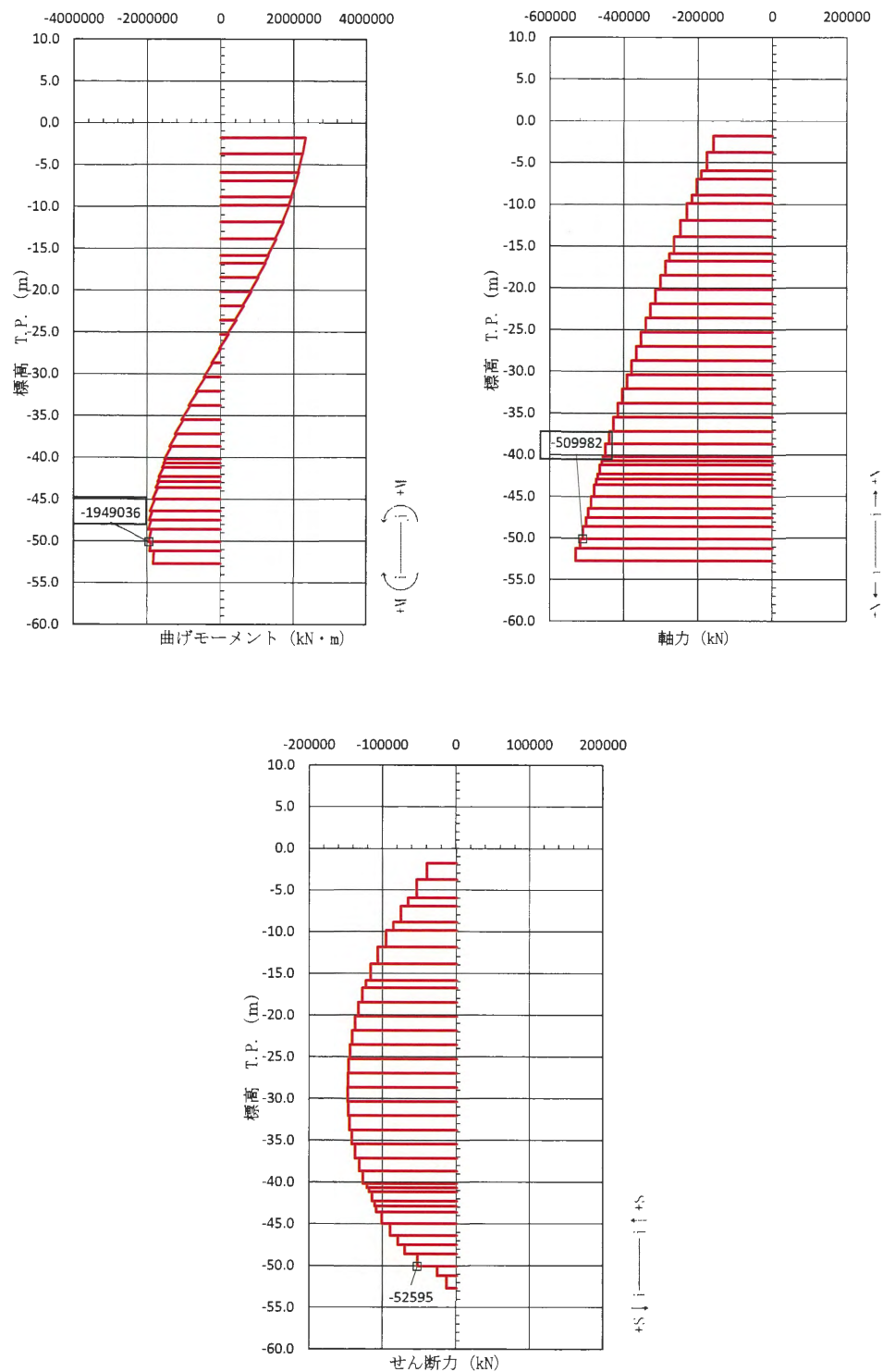
図 3.2-4 コンクリートの曲げ軸力照査が最も厳しい時刻の断面力図 (①-①断面, 北基礎) (S_s - 3.1 [H+, V+] t = 8.82 \text{ s}) (地盤ケース④: 敷地に存在しない豊浦標準砂の液状化強度特性により 地盤を強制的に液状化させることを仮定した解析ケース)
