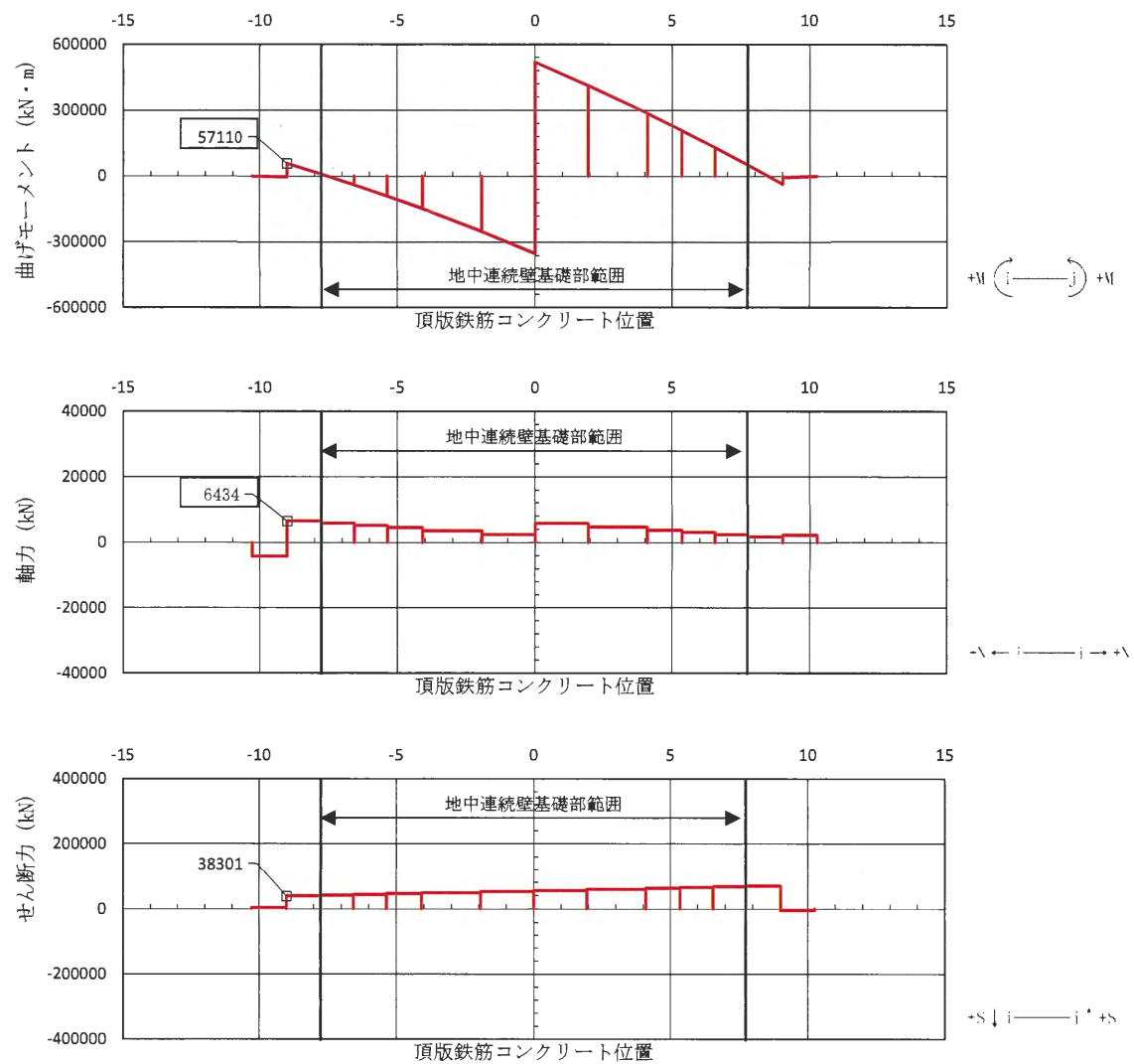
図 3.2-83 コンクリートの曲げ軸力照査が最も厳しい時刻の断面力図（②-②断面，北基礎 西側） （S s -31 [H+, V+] t=8.95 s）
