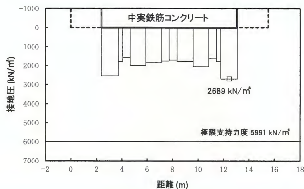
図 3.2-109 ①-①断面南基礎地盤の最大接地圧分布図 ( S_s-31 [H+, V+]) (地盤ケース①：原地盤に基づく液化化強度特性を用いた解析ケース)
