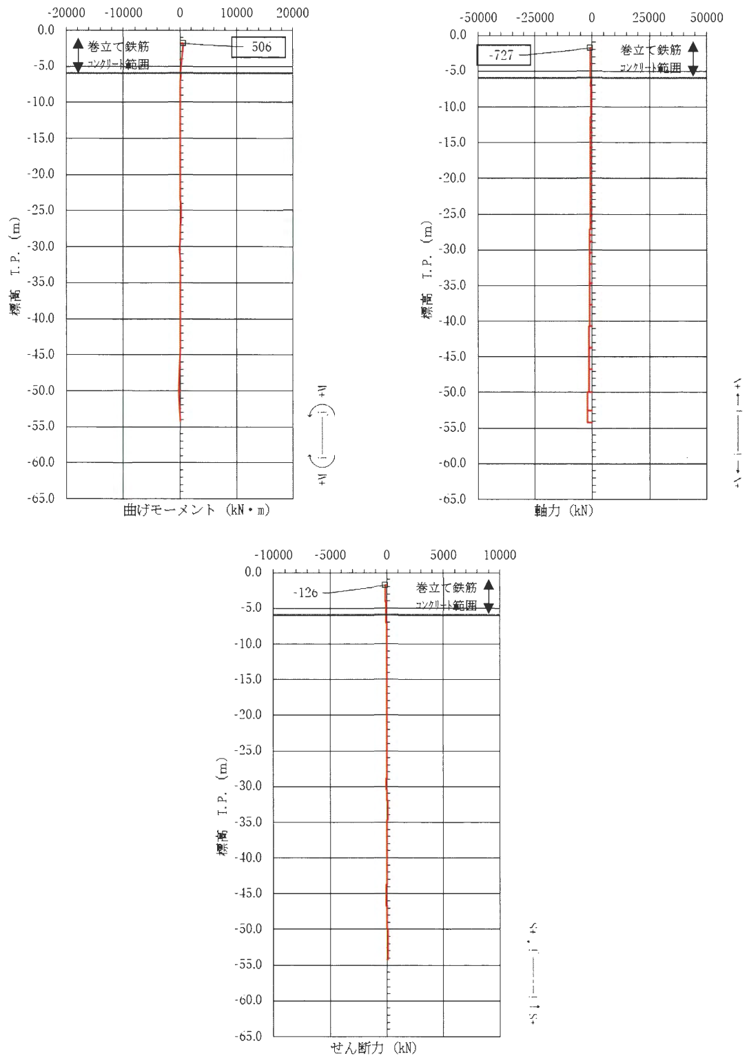
図 3.2-31 コンクリートの曲げ軸力照査が最も厳しい時刻の断面力図 (①-①断面, 南基礎 中間部) (S s -31 [H+, V+] t=9.10 s) (地盤ケース③: 地盤物性のばらつきを考慮 (-1σ) した解析ケース)
