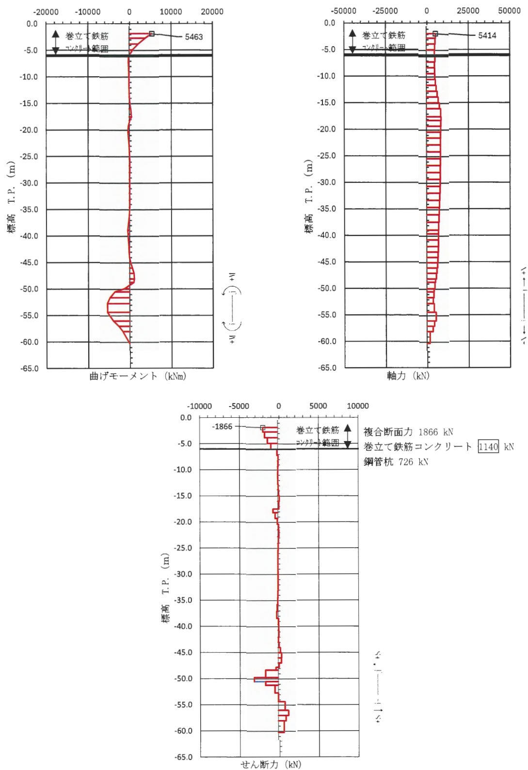
図 3.2-44 鉄筋コンクリートのせん断照査が最も厳しい時刻の断面力図 (②-②断面, 北基礎 西側) (S s - 31 [H+, V+] t = 8.94 s)
