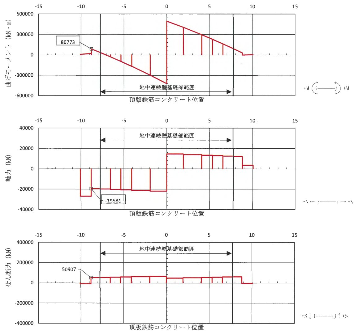
図 3.2-82 コンクリートの曲げ軸力照査が最も厳しい時刻の断面力図（③-③断面，南基礎 西側） (S_s - D1 [H-, V-] \quad t = 27.06 \text{ s})
