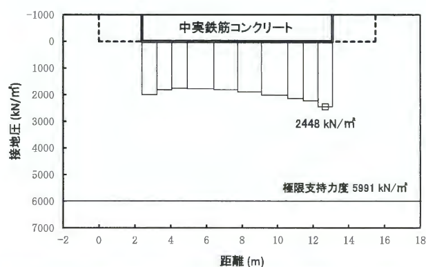
図 3.2-125 ③-③断面南基礎地盤の最大接地圧分布図 (S s -D1 [H-, V-])
