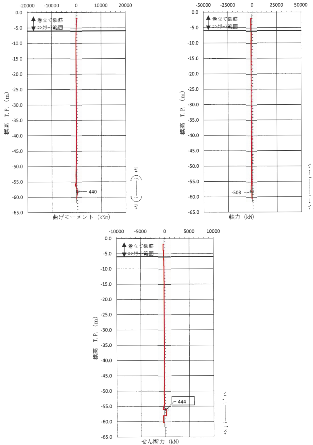
図 3.2-26 鋼管杭のせん断照査が最も厳しい時刻の断面力図 (①-①断面, 北基礎)
