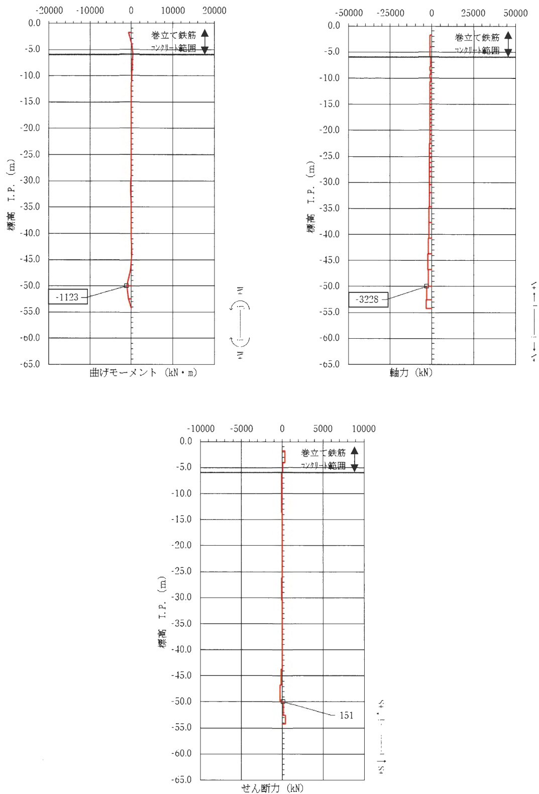
図 3.2-16 鋼管杭の曲げ軸力照査 (圧縮) が最も厳しい時刻の断面力図 (①-①断面, 南基礎) ( S_s - 3.1 [H+, V+] t = 8.85 s)
