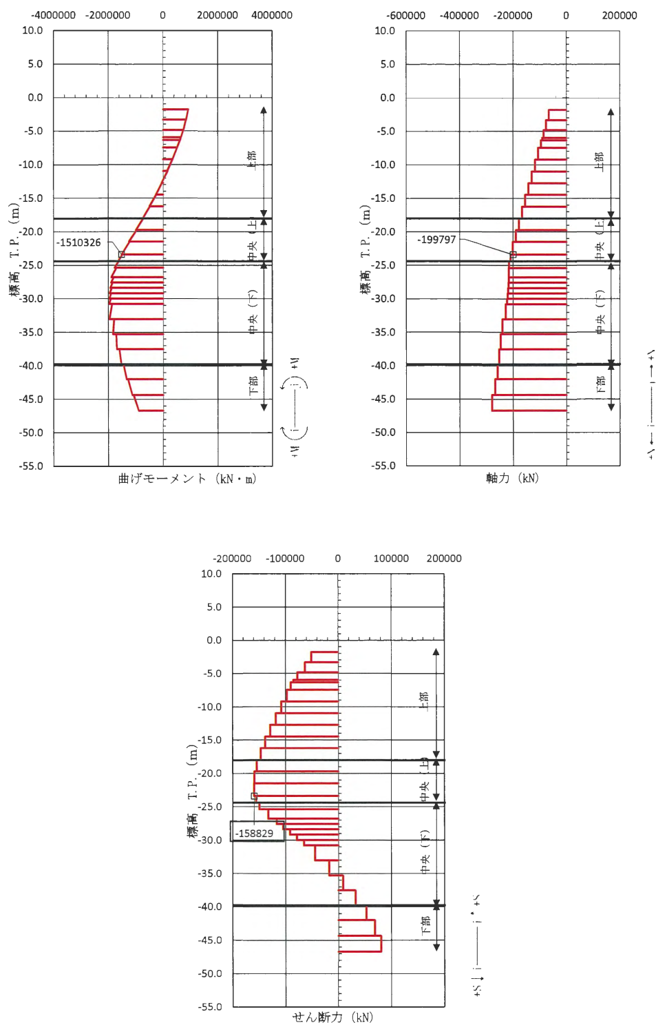
図 3.2-13 鉄筋コンクリートのせん断照査が最も厳しい時刻の断面力図 (③-③断面, 南基礎 中央 (上)) ( S_s-D1 [H-, V-] t=68.78 s) (地盤ケース③: 地盤物性のばらつきを考慮 ( -1\sigma ) した解析ケース)
