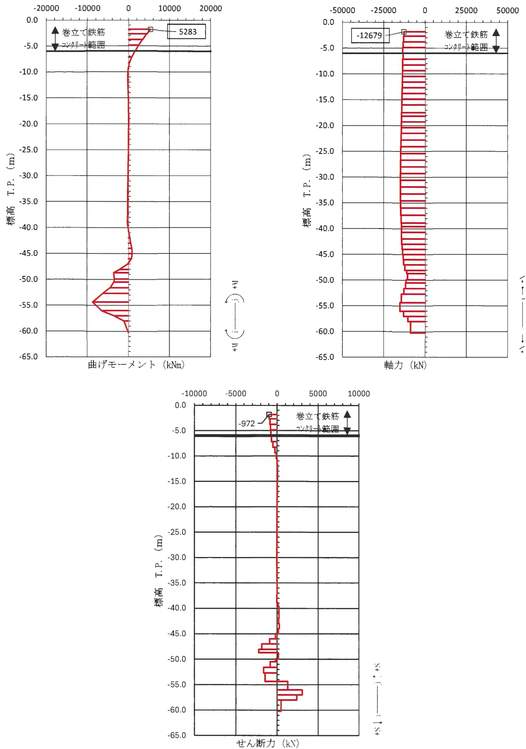
図 3.2-34 コンクリートの曲げ軸力照査が最も厳しい時刻の断面力図 (②-②断面, 北基礎 東側) ( S_s-31 [H+, V+] t=8.85 s)
