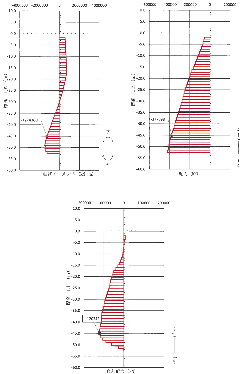
図 3.2-14 鉄筋コンクリートのせん断照査が最も厳しい時刻の断面力図 (②-②断面, 北基礎)
