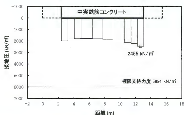
図 3.2-126 ③-③断面南基礎地盤の最大接地圧分布図 (S s -D1 [H-, V-])
