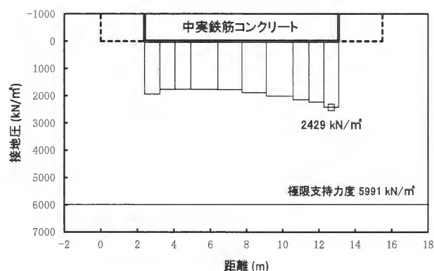
図 3.2-124 ③-③断面南基礎地盤の最大接地圧分布図 (S s -D1 [H-, V-])
