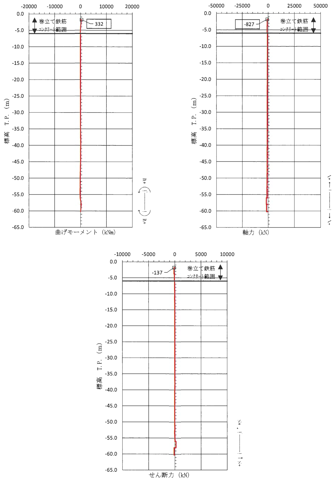
図 3.2-74 コンクリートの曲げ軸力照査が最も厳しい時刻の断面力図 (①-①断面, 北基礎 中間部)
