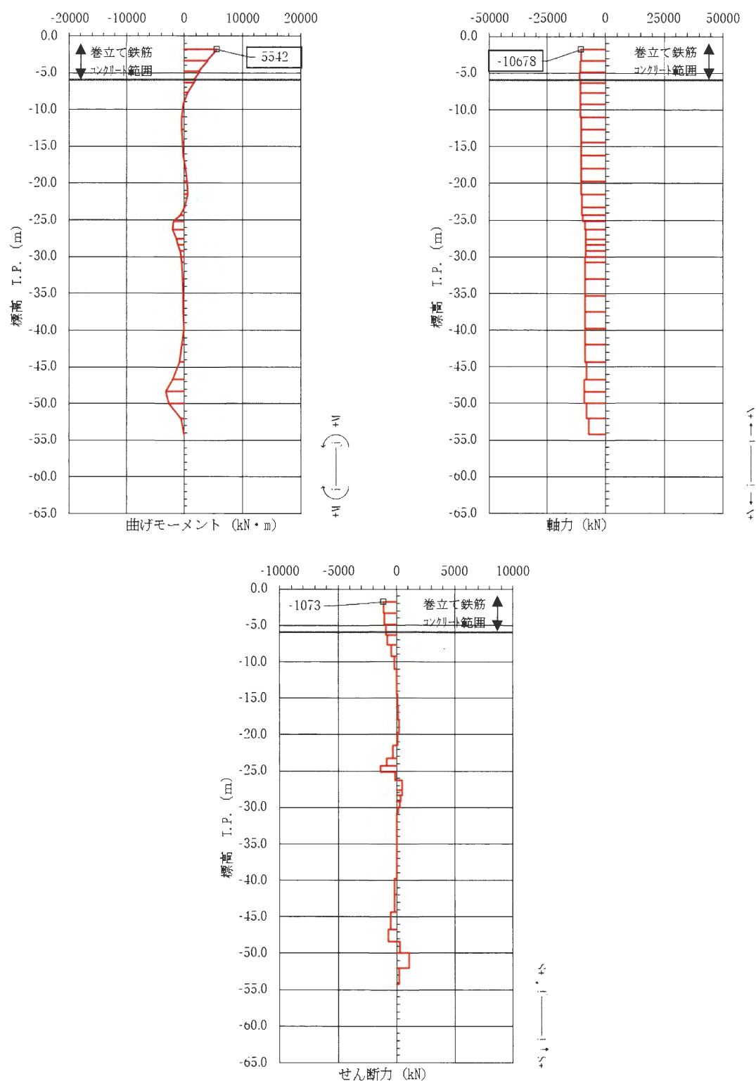
図 3.2-75 コンクリートの曲げ軸力照査が最も厳しい時刻の断面力図 (③-③断面, 南基礎 東側) (S_s - D1 [H-, V-] \ t = 60.51 \text{ s}) (地盤ケース③: 地盤物性のばらつきを考慮 ( -1\sigma ) した解析ケース)
