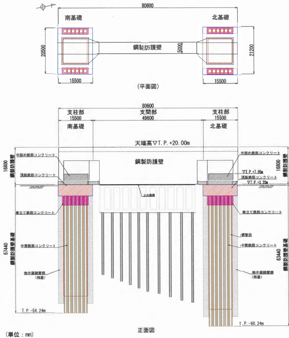
図 2.5-7 防潮堤 (鋼製防護壁) の全体構造図
