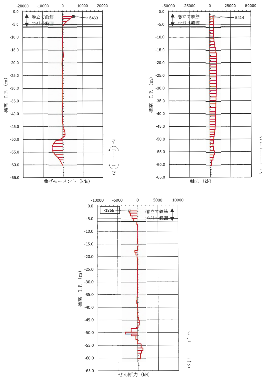
図 3.2-60 巻立て鉄筋コンクリート内の鋼管杭のせん断照査が最も厳しい時刻の断面力図
