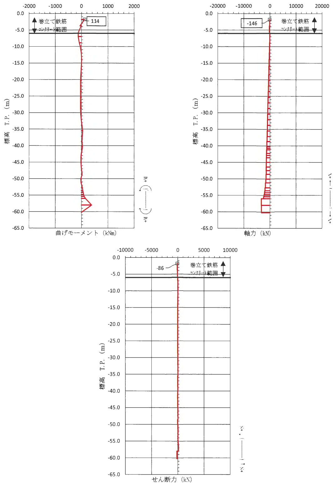
図 3.2-68 鉄筋の曲げ軸力照査が最も厳しい時刻の断面力図 (①-①断面, 北基礎 端部)
