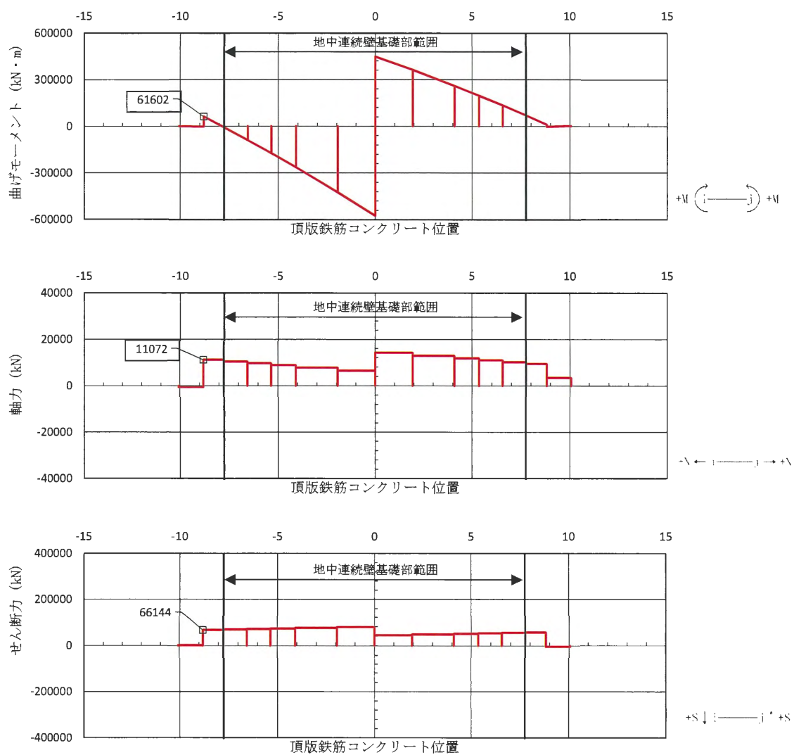
図 3.2-84 鉄筋の曲げ軸力照査が最も厳しい時刻の断面力図 (③-③断面, 南基礎 西側) (S_s - D1 [H-, V-] \quad t = 26.87 \text{ s}) (地盤ケース②: 地盤物性のばらつきを考慮 (+1 \sigma ) した解析ケース)
