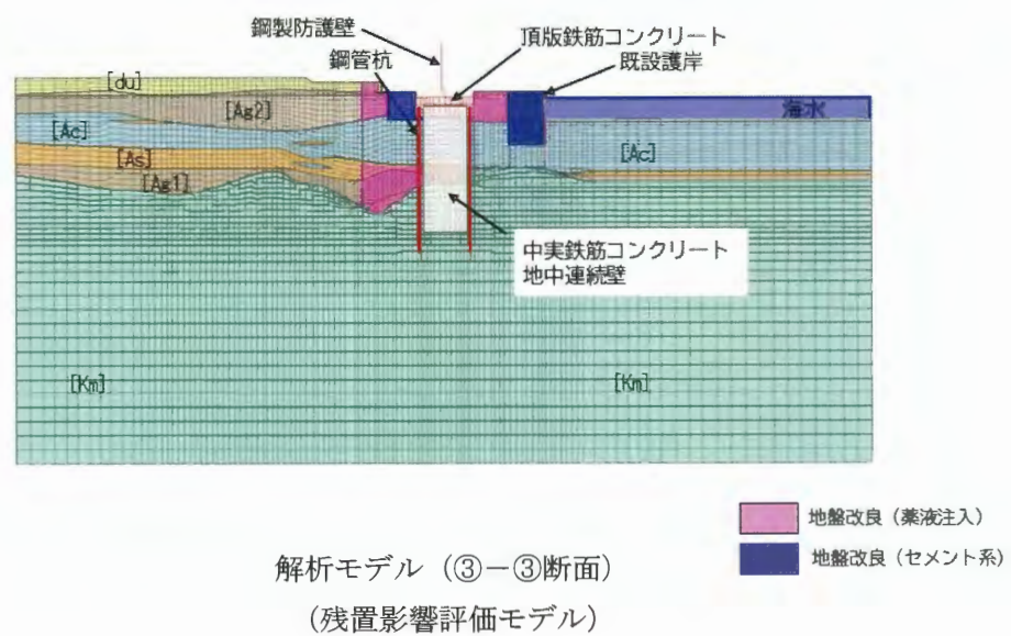
図 3.1-6 解析モデルの比較 (③-③断面)
