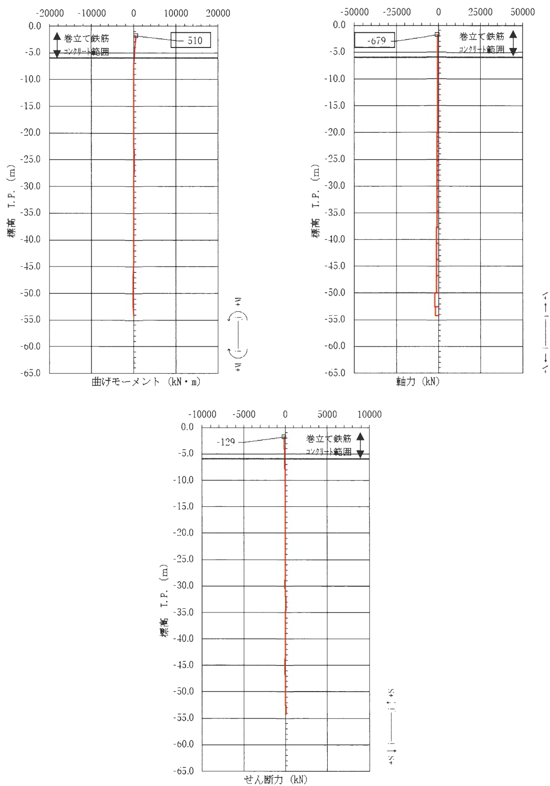
図 3.2-73 コンクリートの曲げ軸力照査が最も厳しい時刻の断面力図 (①-①断面, 南基礎 中間部) (S_s - 3.1 \text{ [H+, V+]} t = 9.13 \text{ s}) (地盤ケース③: 地盤物性のばらつきを考慮 ( -1\sigma ) した解析ケース)
