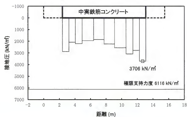
図 3.2-127 ②-②断面北基礎地盤の最大接地圧分布図 ( S_s-31 [H+, V+]) (地盤ケース①：原地盤に基づく液状化強度特性を用いた解析ケース)
