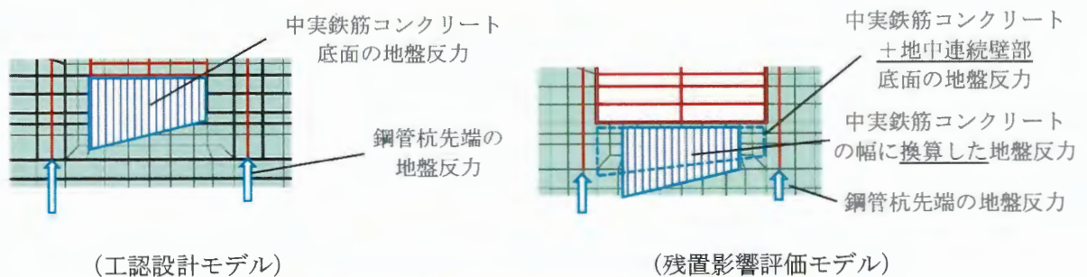
図 2.5-6 支持性能評価のイメージ図
