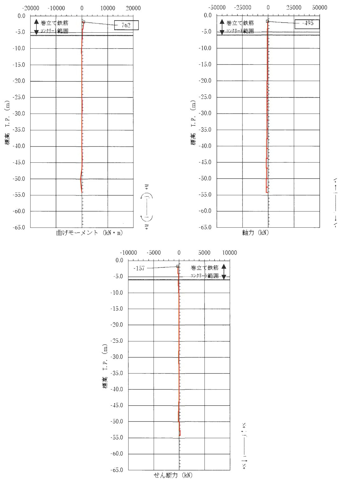
図 3.2-77 鉄筋の曲げ軸力照査が最も厳しい時刻の断面力図 (①-①断面, 南基礎 端部)
