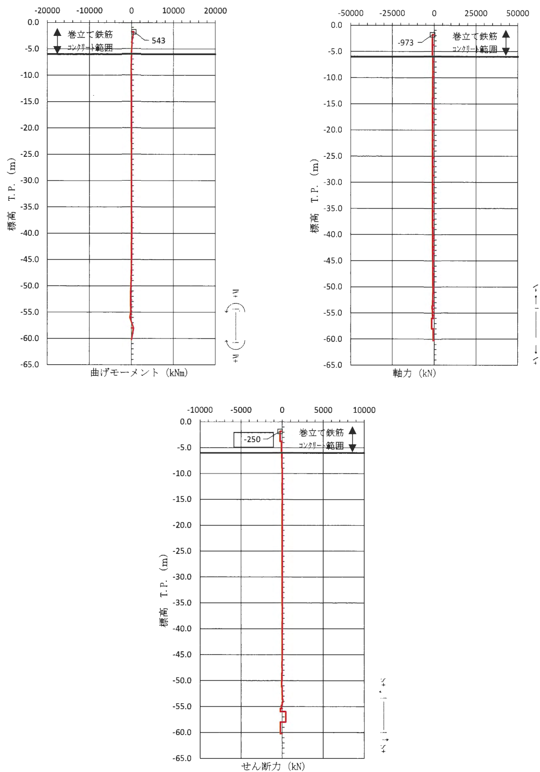
図 3.2-58 巻立て鉄筋コンクリート内の鋼管杭のせん断照査が最も厳しい時刻の断面力図 (①-①断面, 北基礎 端部) (S s - 3 1 [H+, V+] t=9.55 s) (地盤ケース②: 地盤物性のばらつきを考慮 (+1σ) した解析ケース)
