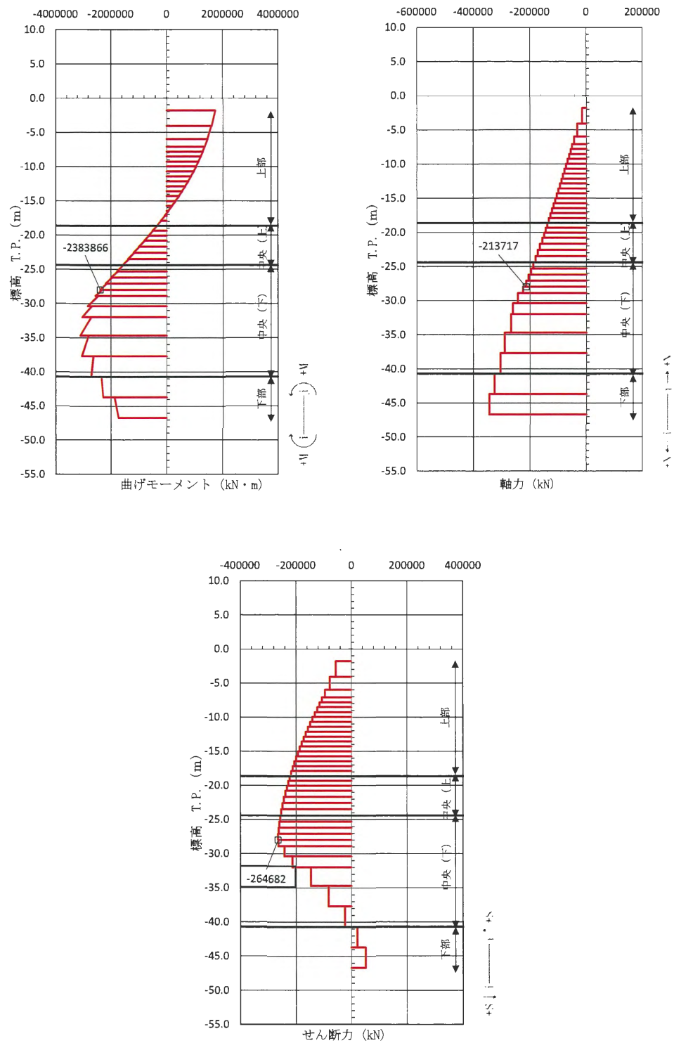
図 3.2-11 鉄筋コンクリートのせん断照査が最も厳しい時刻の断面力図
