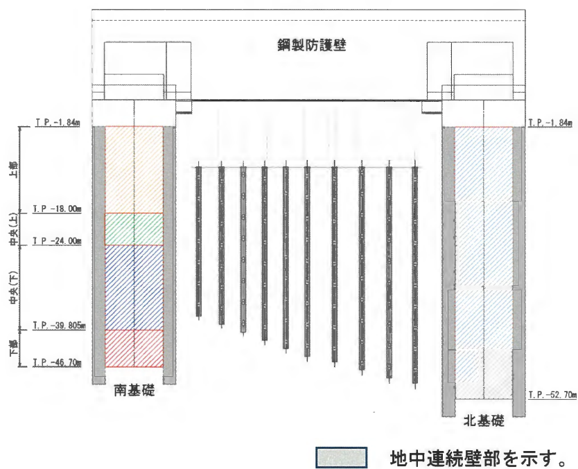
図 4.2-1 評価位置図（中実鉄筋コンクリート）
