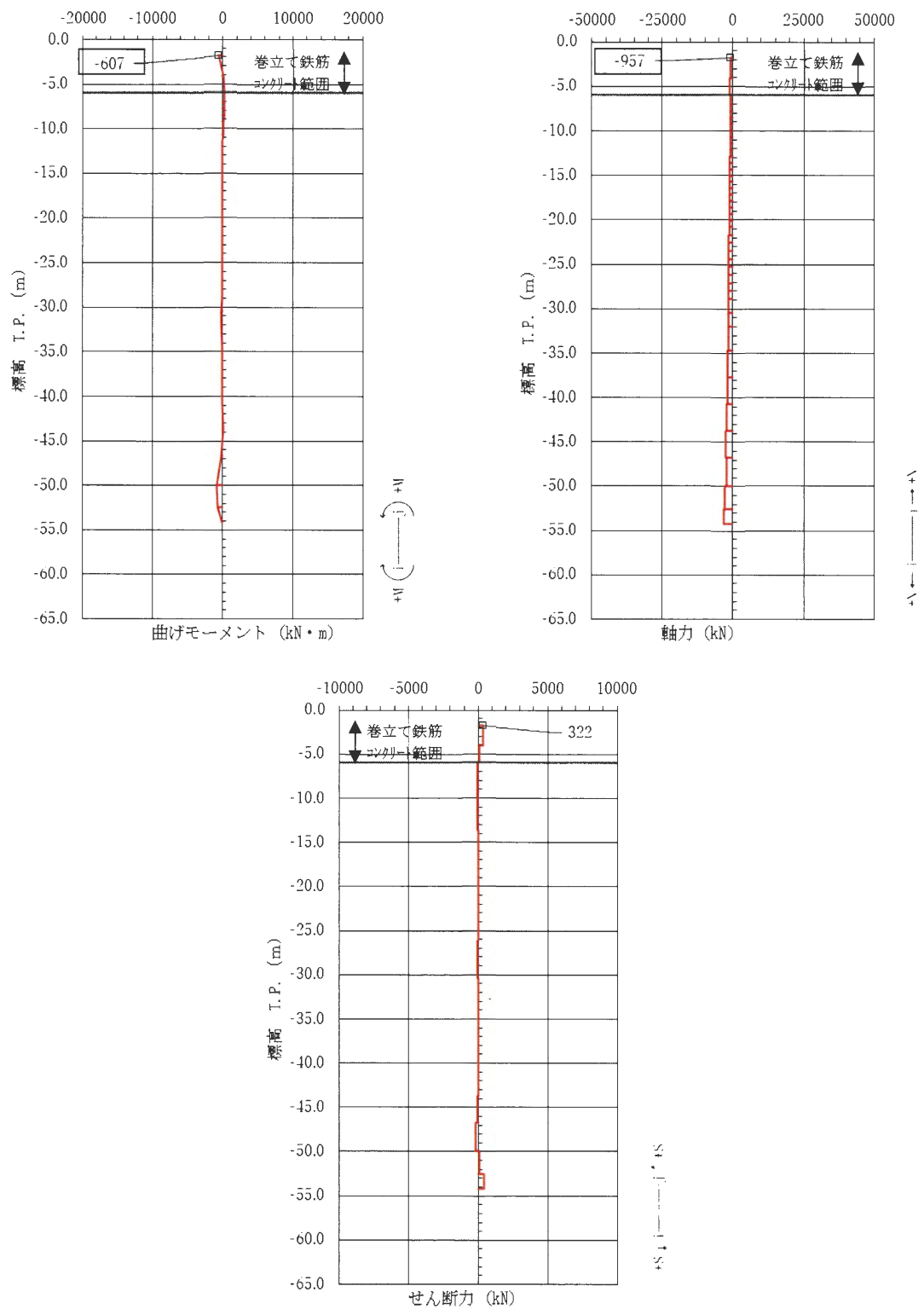
図 3.2-63 コンクリートの曲げ軸力照査が最も厳しい時刻の断面力図 (①-①断面, 南基礎 端部) (S_s - 3.1 \text{ [H+, V+]} t = 8.82 \text{ s}) (地盤ケース②: 地盤物性のばらつきを考慮 (+1 \sigma ) した解析ケース)
