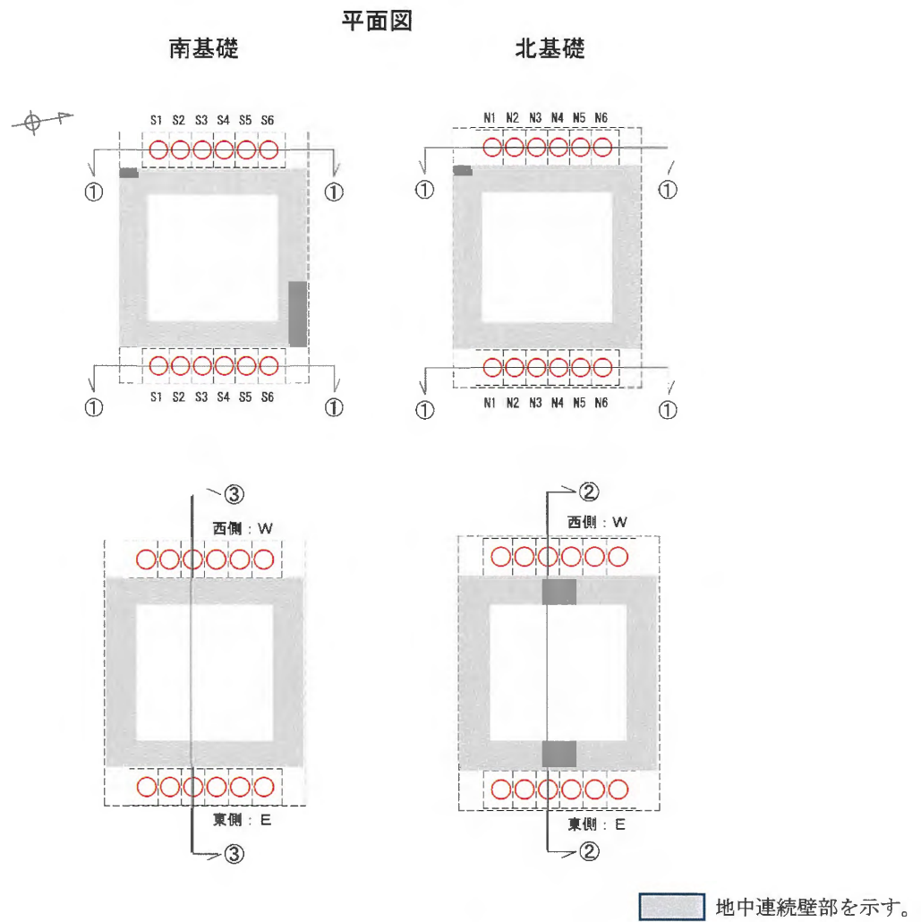
図 3.2-108 杭記号位置図（鋼管杭）
