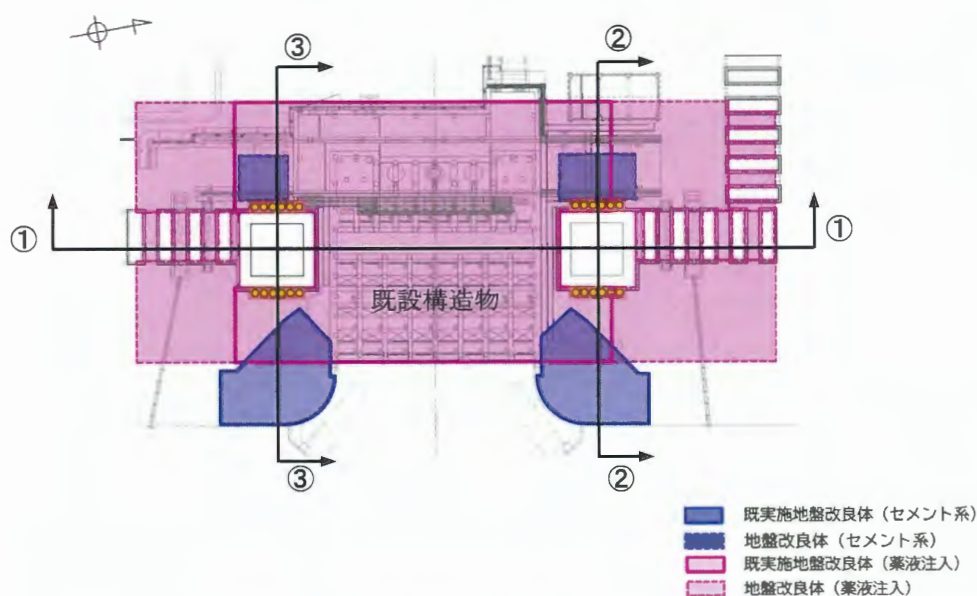
図 3.1-3 解析断面位置図
