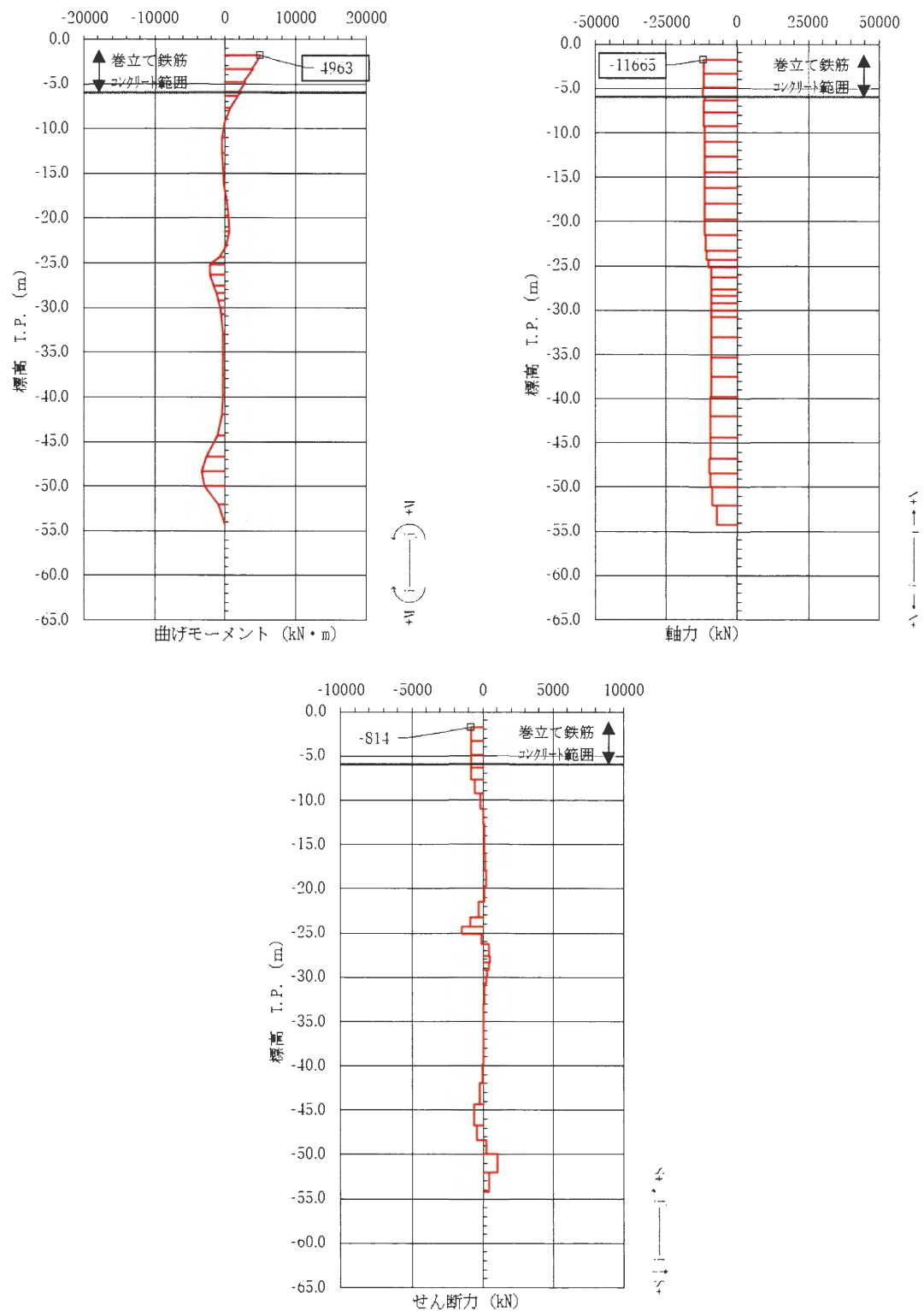
図 3.2-65 コンクリートの曲げ軸力照査が最も厳しい時刻の断面力図 (③-③断面, 南基礎 東側) ( S_s-D1 [H-, V-] t=53.95 s)
