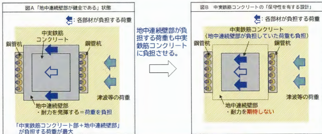
図 2.5-5 中実鉄筋コンクリートの荷重負担
