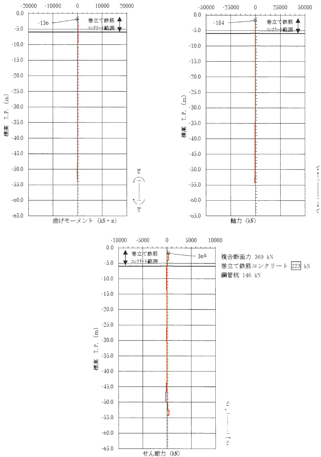
図 3.2-41 鉄筋コンクリートのせん断照査が最も厳しい時刻の断面力図 (①-①断面, 南基礎 端部) (S s - 3 1 [H+, V+] t = 8.82 s)
