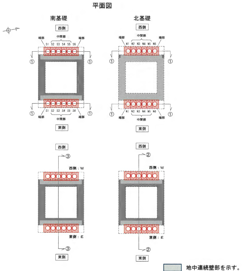
図 3.2-39 評価位置及び杭記号位置図（巻立て鉄筋コンクリート）
