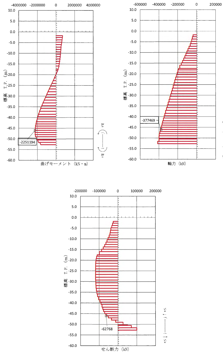
図 3.2-9 鉄筋の曲げ軸力照査が最も厳しい時刻の断面力図 (②-②断面, 北基礎) (S_s - 3.1 [H+, V+] \quad t = 8.93 \text{ s}) (地盤ケース③: 地盤物性のばらつきを考慮 ( -1\sigma ) した解析ケース)
