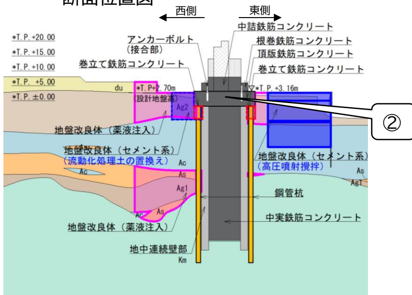
(b)-(b)断面図
