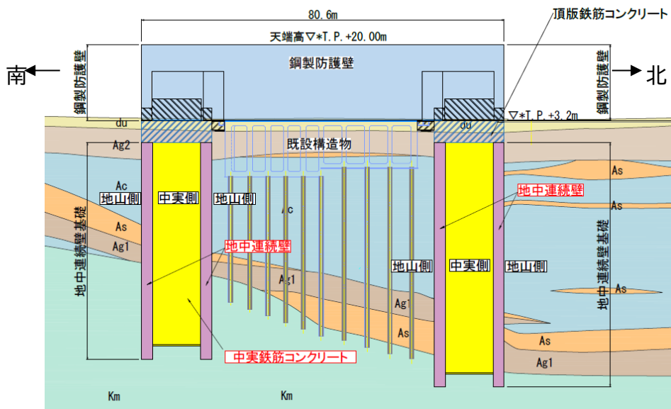
防潮堤（鋼製防護壁，既工認）
