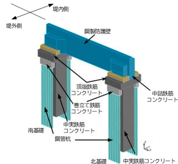
防潮堤（鋼製防護壁）の各構成部位
