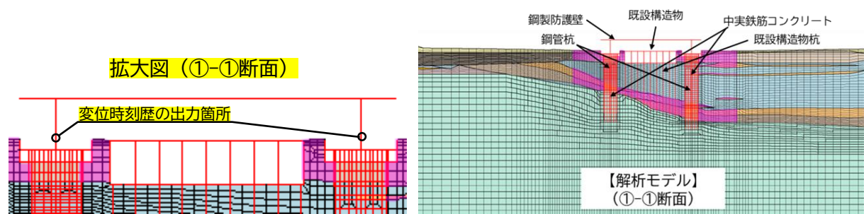
2次元FEMモデル（鋼製防護壁基礎）
