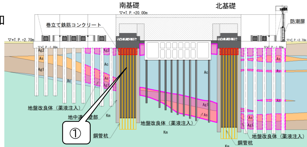
(a)-(a)断面図
