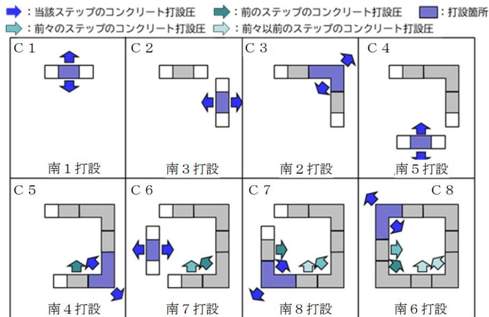
構築ステップごとのコンクリート打設に伴う地盤への 施工圧力の蓄積履歴 (南基礎の例)
