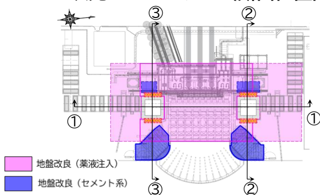
2次元FEMモデル（断面位置図）
