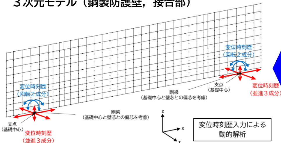
3次元モデル（鋼製防護壁，接合部）
