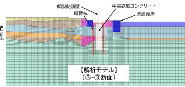
拡大図（③-③断面）
