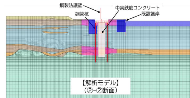
拡大図（②-②断面）
