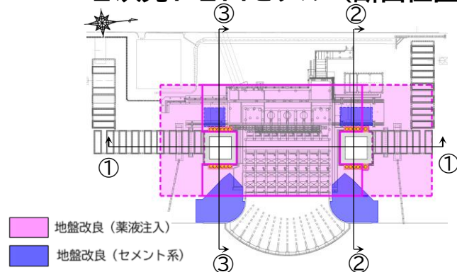
2次元FEMモデル（断面位置図）
