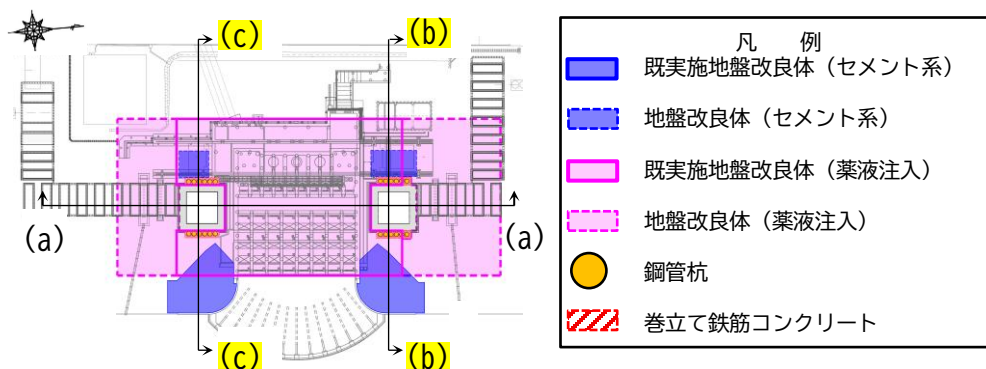
断面位置図
