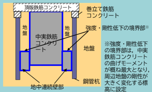
【部分欠損モデル】
