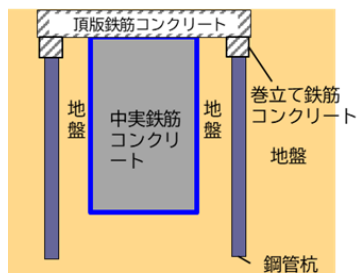
【工認設計モデル】
