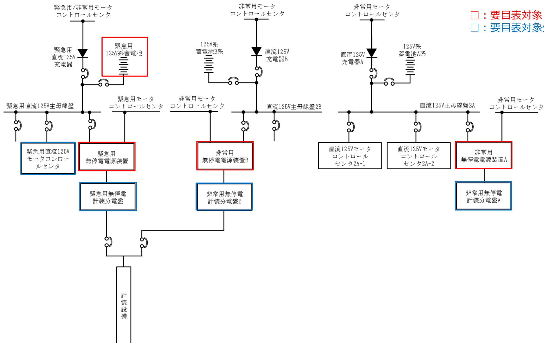
参考 1 図 1 単線結線図
