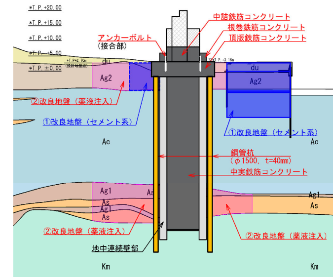
北基礎断面図※1
