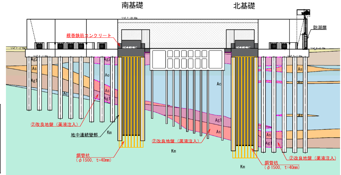
(a)-(a)断面図※1
