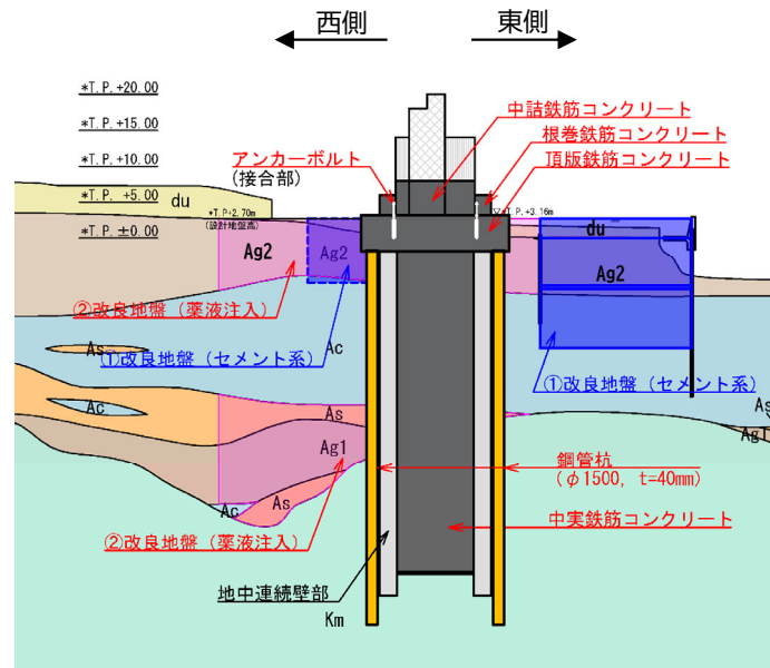
(b)-(b)断面図※1
