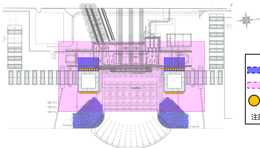
平面図※1（改良範囲図）
