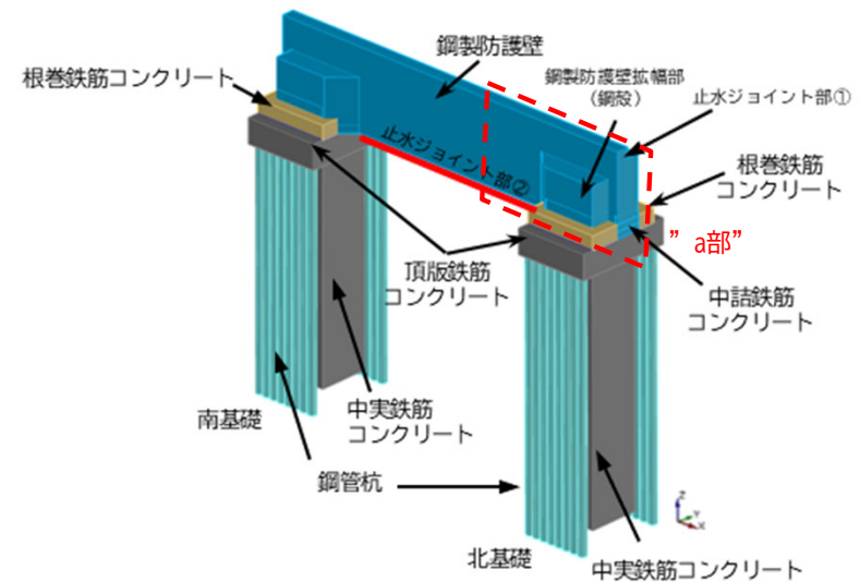
鋼製防護壁全体の構造図（鳥瞰図）
