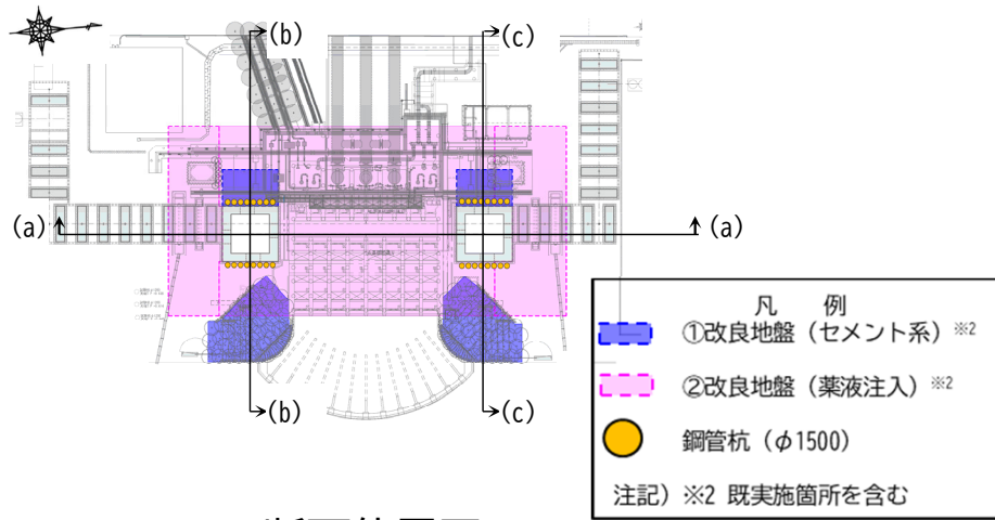
断面位置図
