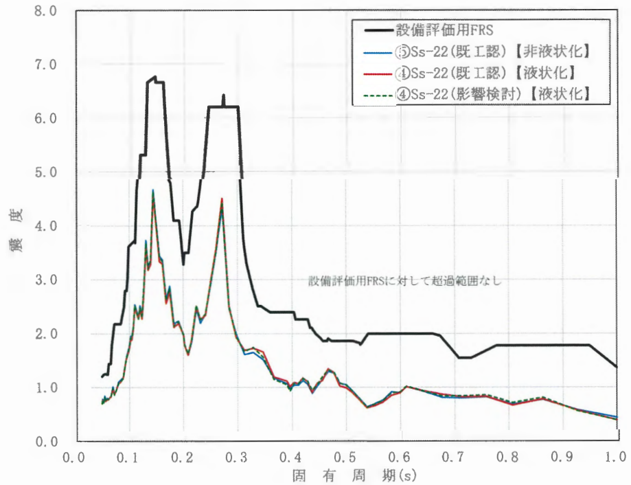
図 2.4.1-11 FRSの比較結果（鉛直方向 EL.-3.357m h=2.0%）
