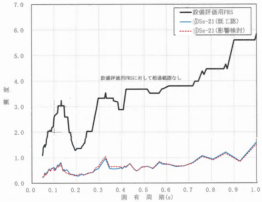
図 2.4.2-20 FRS の比較結果 (地盤ケース㉔, 水平方向, EL. -6.49m, h=2.0%)
