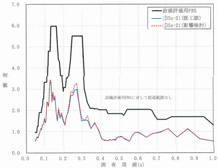
図 2.4.2-23 FRS の比較結果 (地盤ケース㊸, 鉛直方向, EL. -7.40m, h=2.0%)
