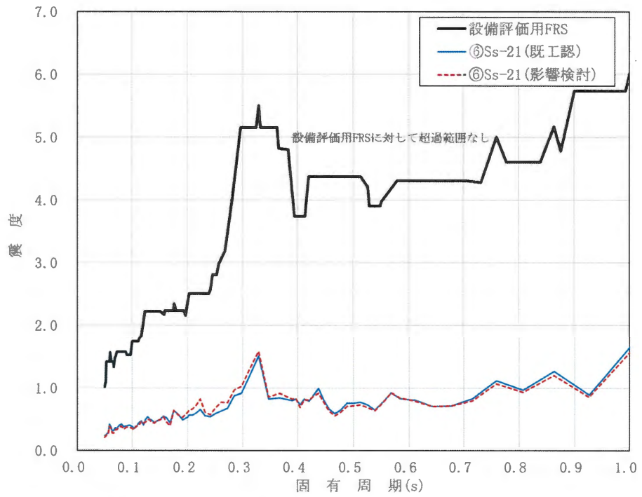
図 2.4.2-18 FRS の比較結果（地盤ケース㊸，水平方向，EL. 0.30m，h=2.0%）
