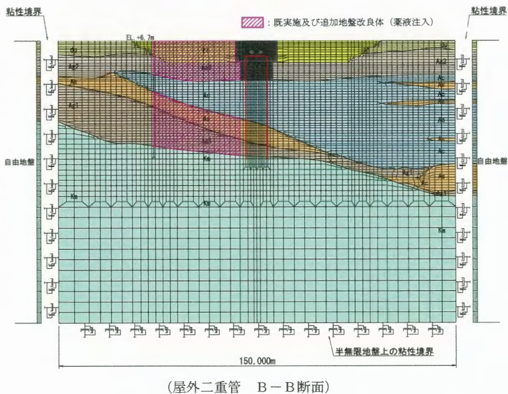
参考図4-2 影響検討モデル図 (再掲)
