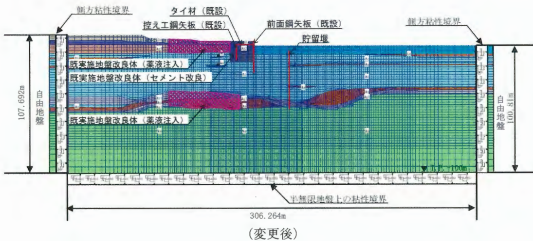
図 5.2-2(2) 解析モデル図 (EW-2 断面)
