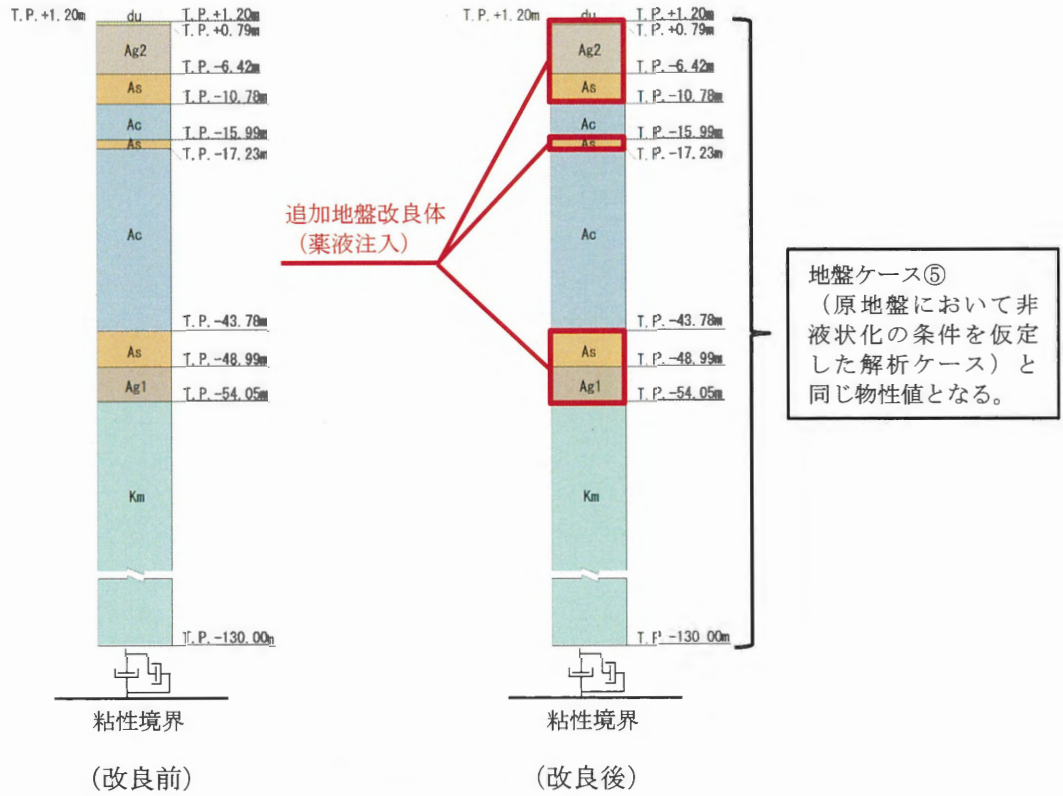
図 1.4-2 追加地盤改良体を考慮した1次元地盤応答解析モデル
