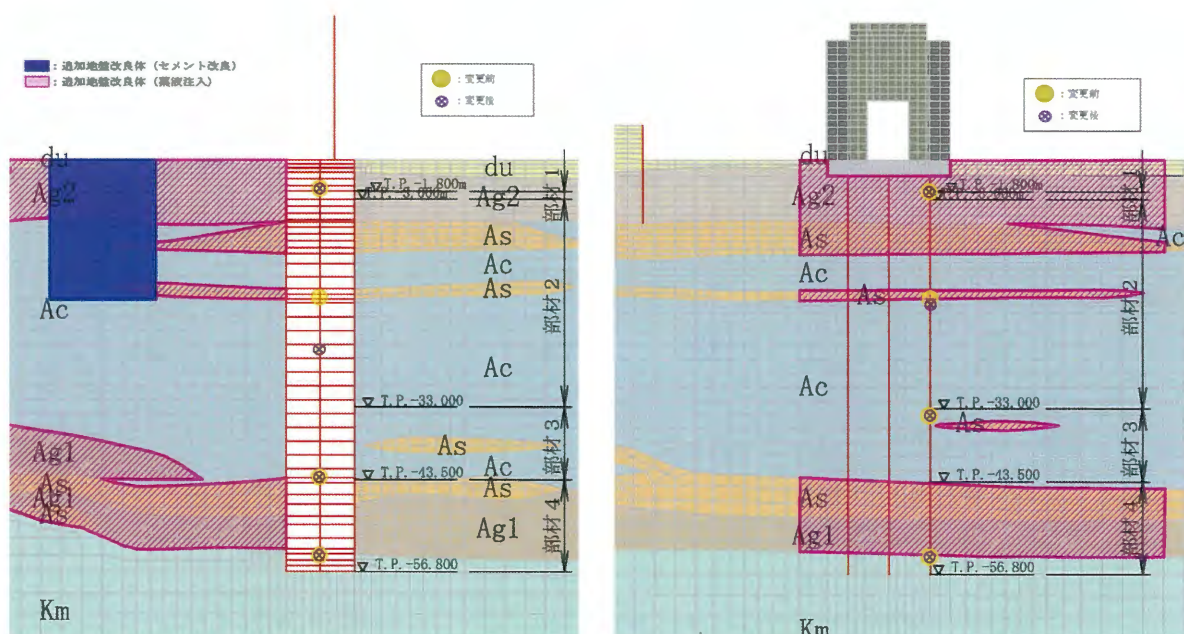
(①-①断面)
