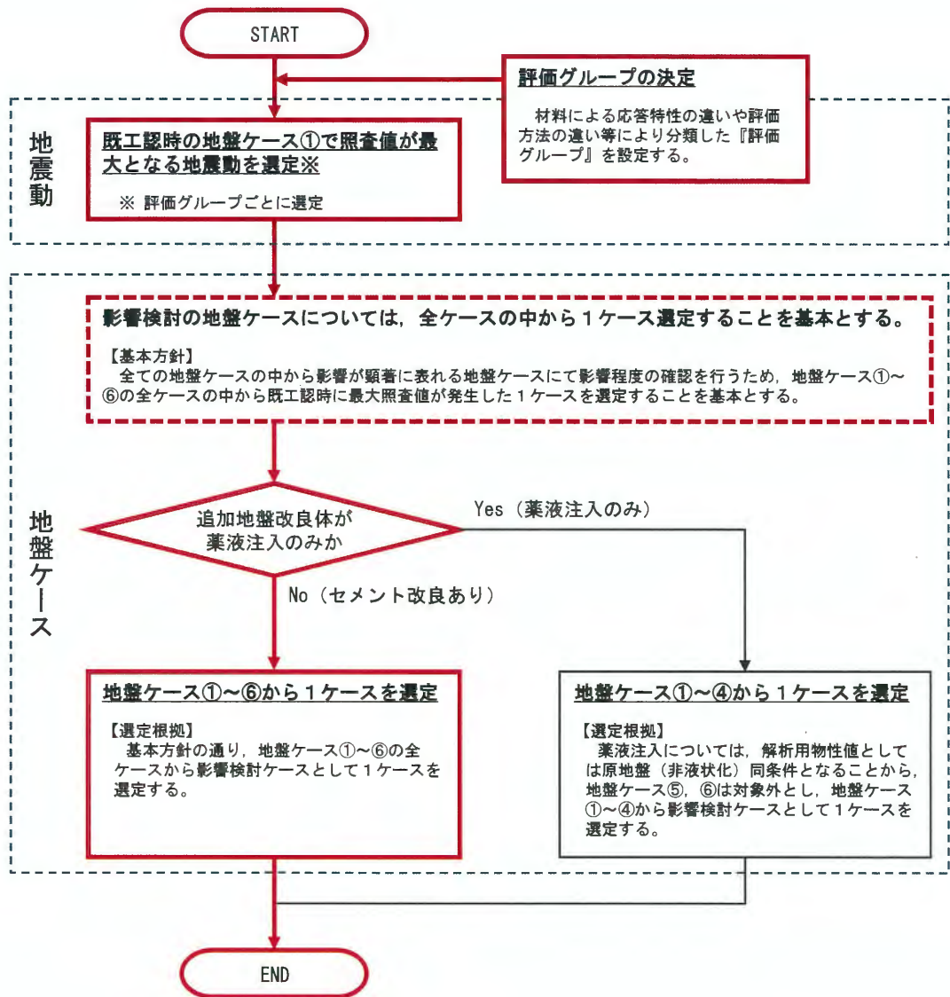
図 3. 3-1 (1) 施設評価の影響検討ケースの選定ルート 防潮堤（鉄筋コンクリート防潮壁） (①-①断面)
