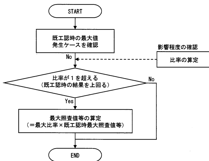
図 1.3-6 最大値の検討における検討フロー
