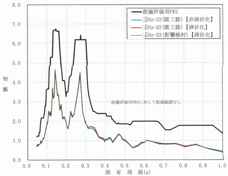
図 2.4.1-13 FRSの比較結果 (鉛直方向 EL.-4.848m h=2.0%)
