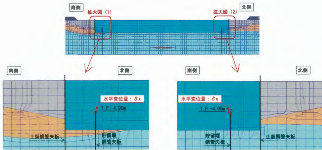
(NS-1 断面)
