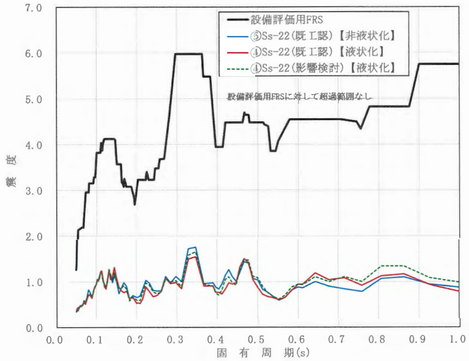
図 2.4.1-6 FRSの比較結果 (水平方向 EL.0.218m h=2.0%)
