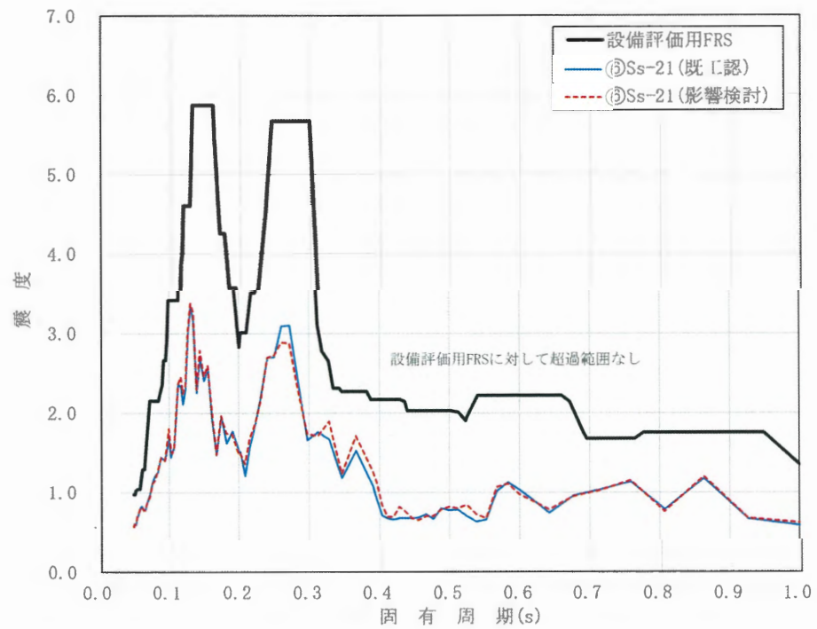
図 2.4.2-25 FRS の比較結果 (地盤ケース㉔, 鉛直方向, EL. -7.46m, h=2.0%)
