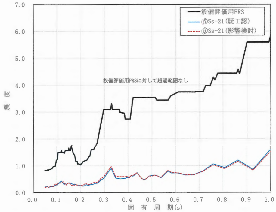
図 2.4.2-22 FRS の比較結果 (地盤ケース㊸, 水平方向, EL. -7.40m, h=2.0%)
