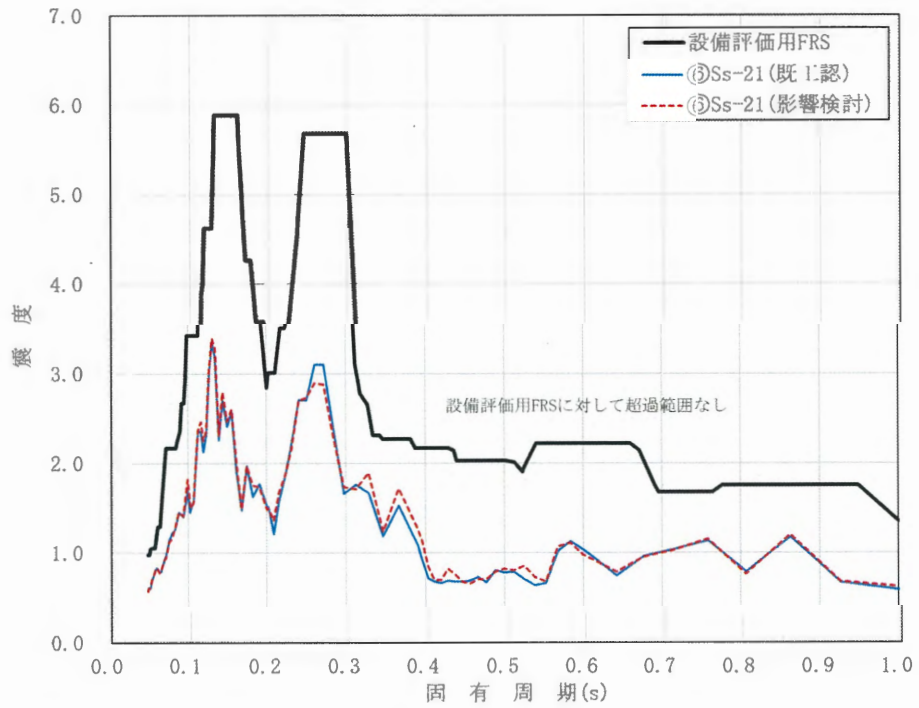
図 2.4.2-21 FRS の比較結果 (地盤ケース㉔, 鉛直方向, EL. -6.49m, h=2.0%)
