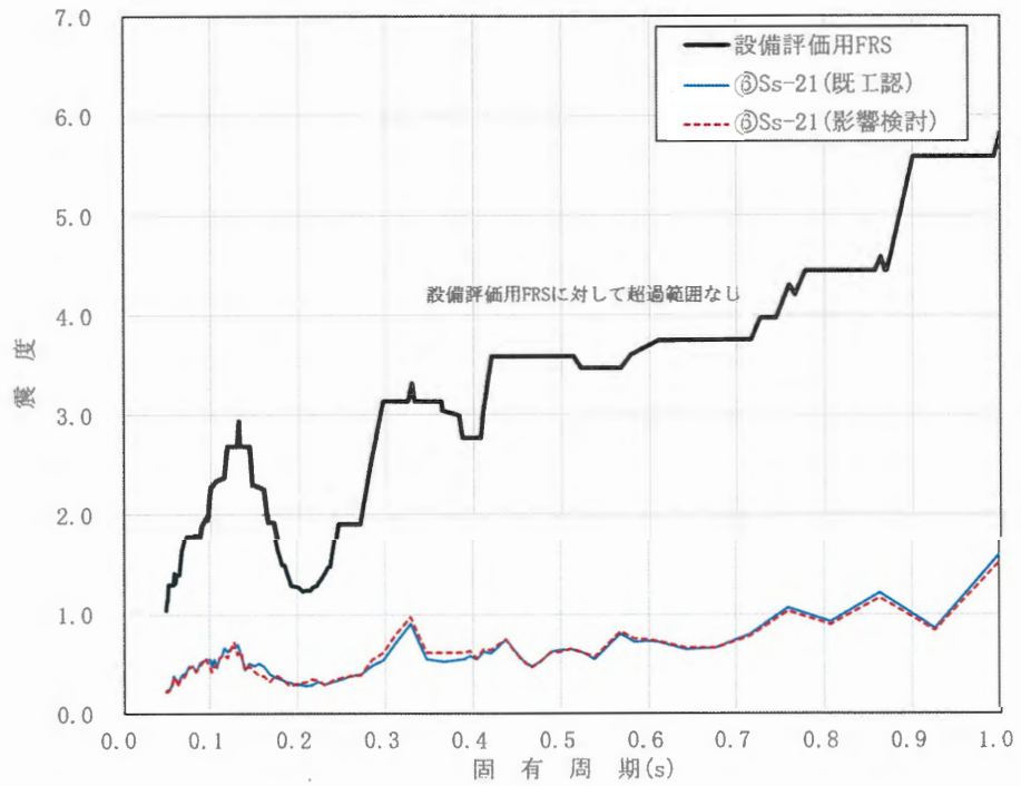
図 2.4.2-24 FRS の比較結果 (地盤ケース㉔, 水平方向, EL. -7.46m, h=2.0%)
