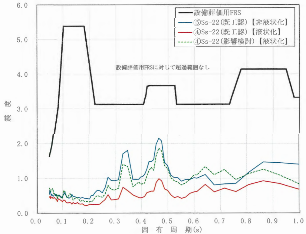
図 4.4-2 FRSの比較結果 (水平方向 h=2.0%)
