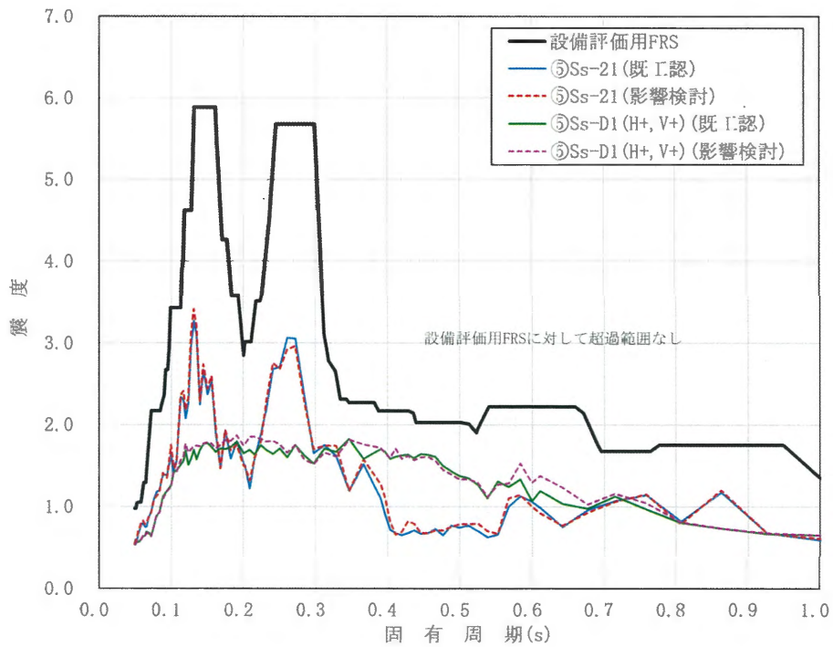
図 2.4.2-13 FR S の比較結果 (地盤ケース㊦, 鉛直方向, EL. -6.49m, h=2.0%)
