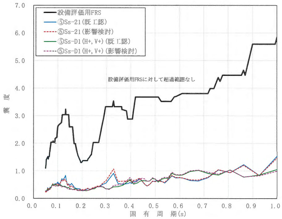
図 2.4.2-12 FR S の比較結果 (地盤ケース㊦, 水平方向, EL. -6.49m, h=2.0%)
