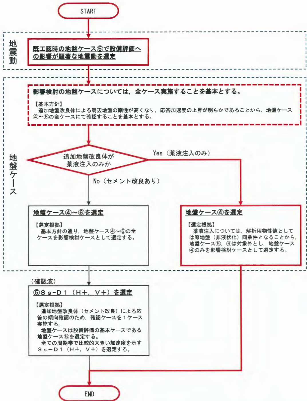
参考図 2-4(2) 設備評価における影響検討ケース選定フロー（結果） ②-②断面，③-③断面及び④-④断面
