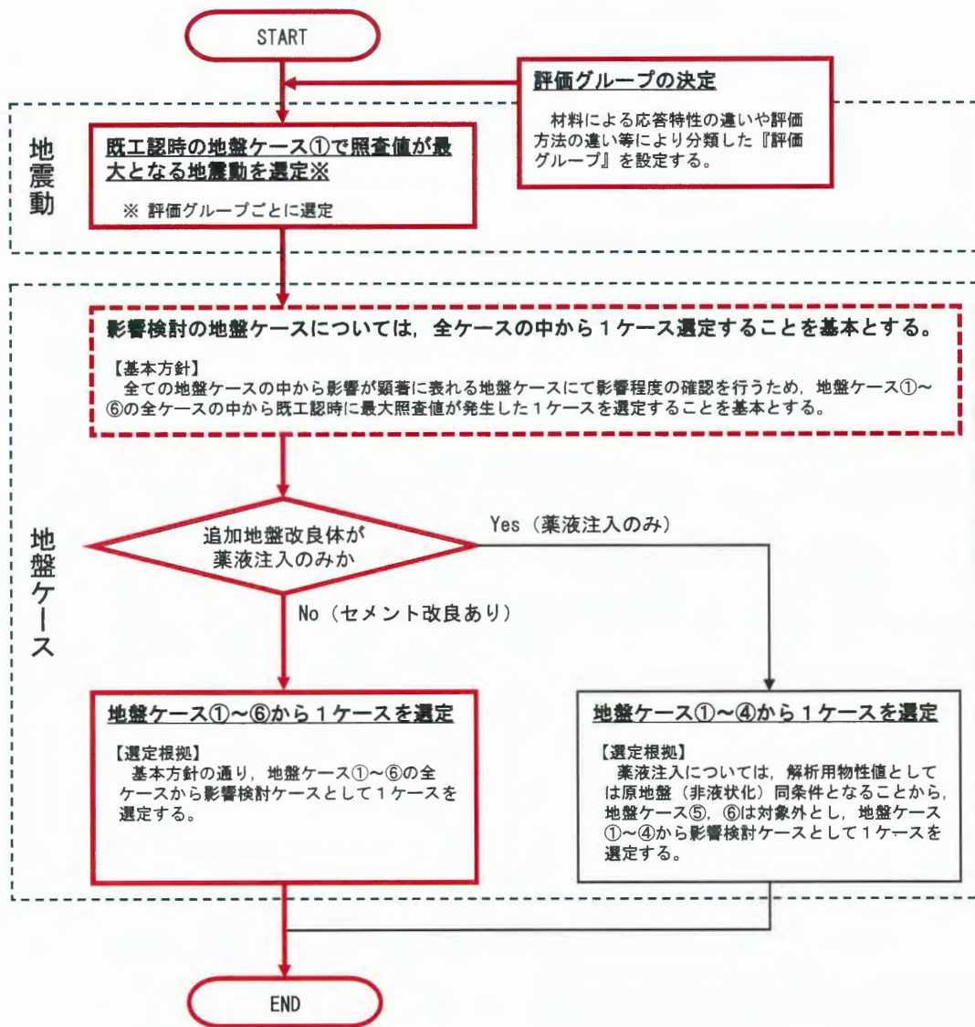
図 2.3-1(2) 施設評価の影響検討ケースの選定ルート 取水構造物 (④-④断面)
