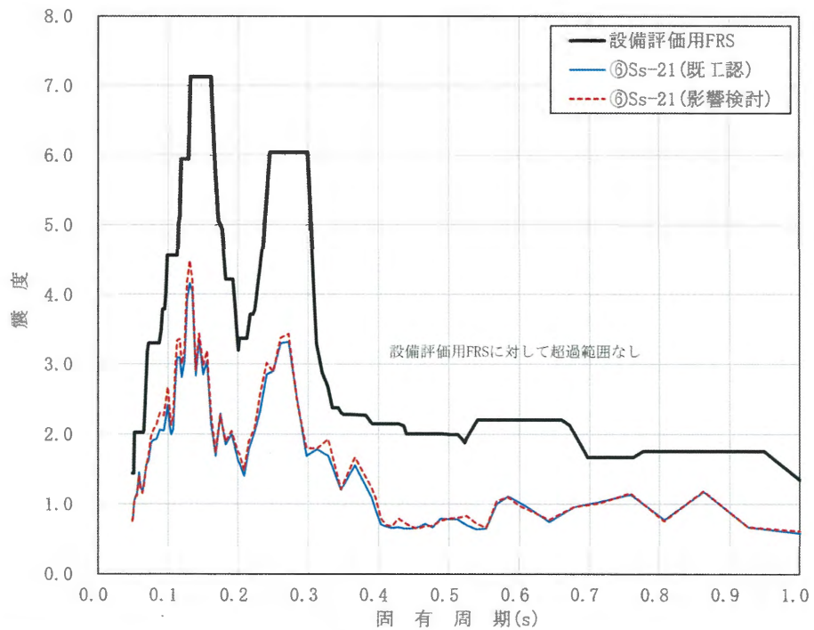
図 2.4.2-19 FRS の比較結果（地盤ケース㊸，鉛直方向，EL. 0.30m，h=2.0%）
