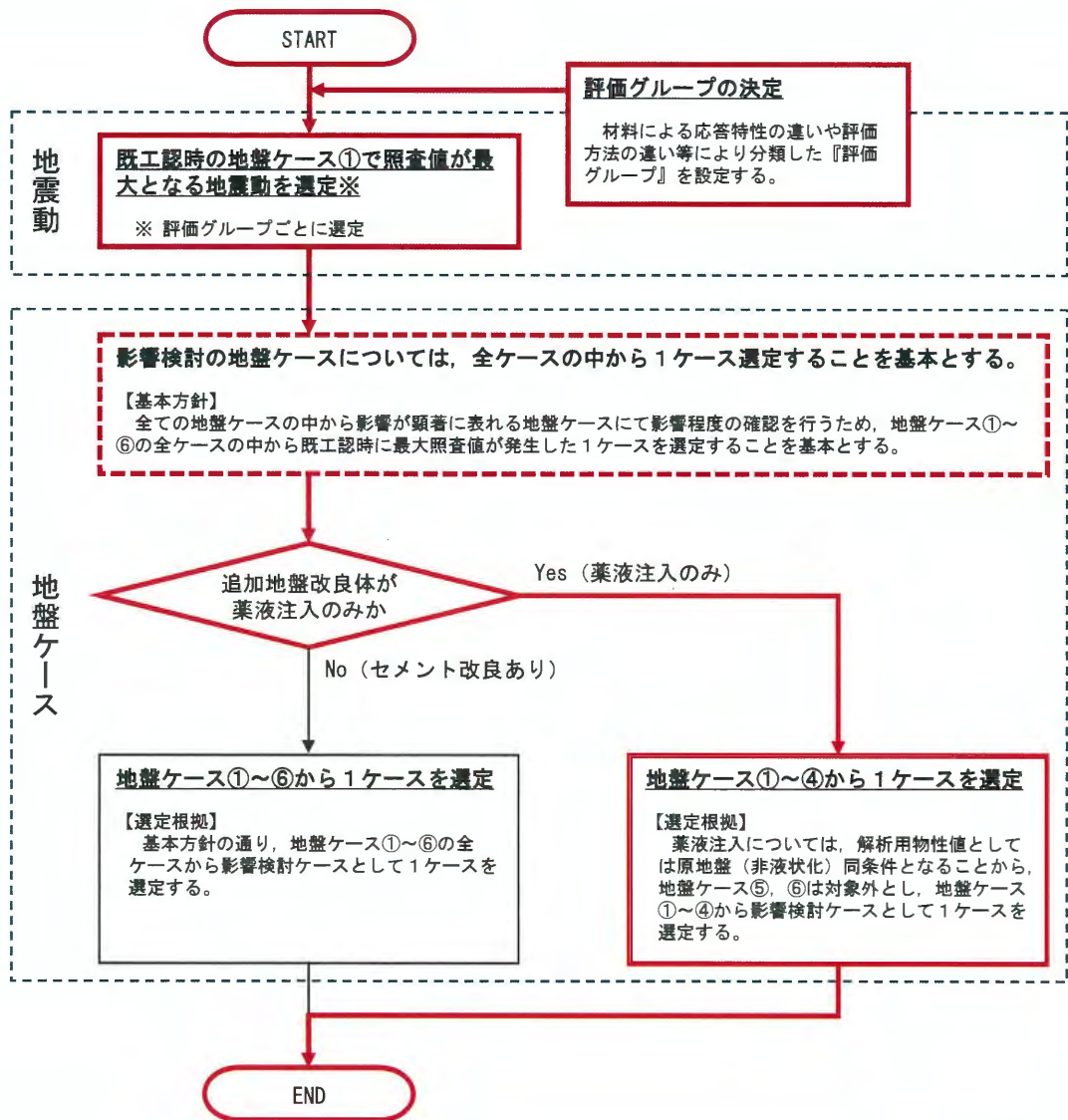
図 2.3-1(1) 施設評価の影響検討ケースの選定ルート 取水構造物 (①-①断面)
