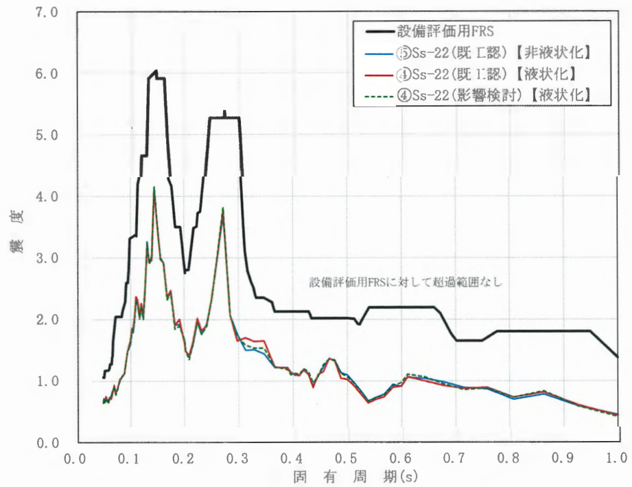
図 2.4.1-7 FRSの比較結果 (鉛直方向 EL.0.218m h=2.0%)
