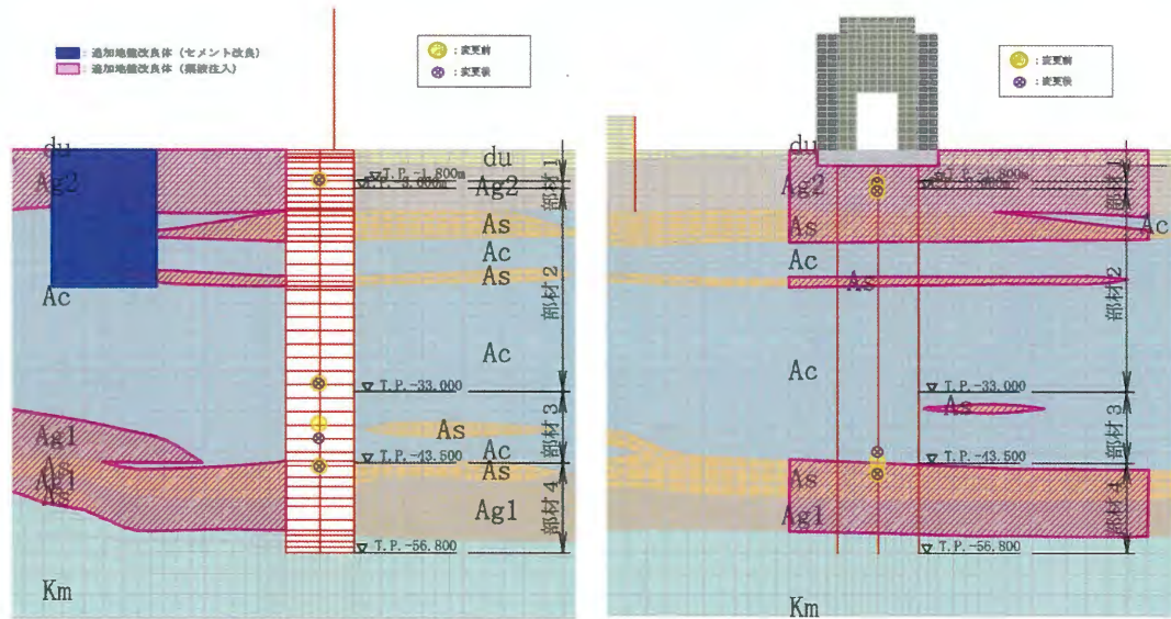
(①-①断面)
