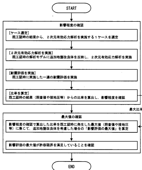
図 1.3-1 施設の耐震評価による影響検討フロー
