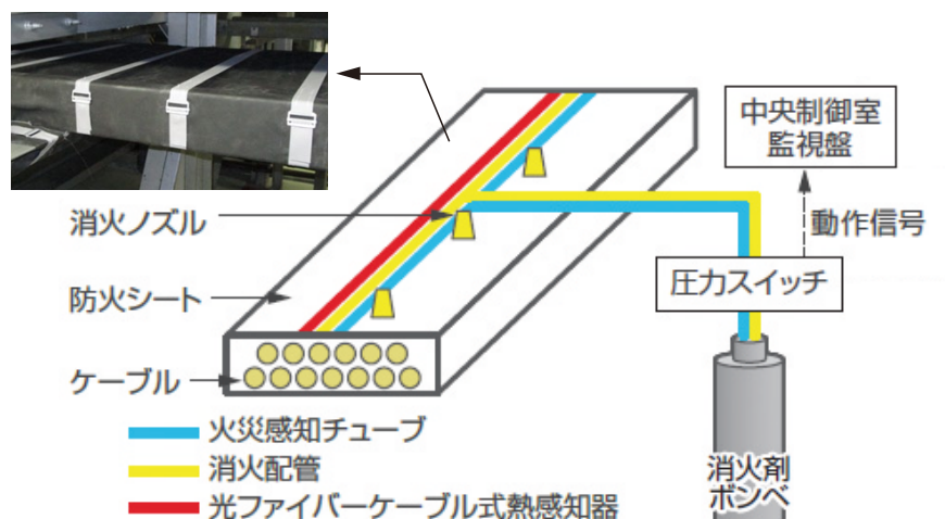
図3 ケーブルトレイ（複合体）内の消火設備
