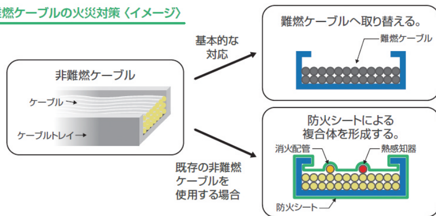
図2 ケーブルの火災発生防止対策
