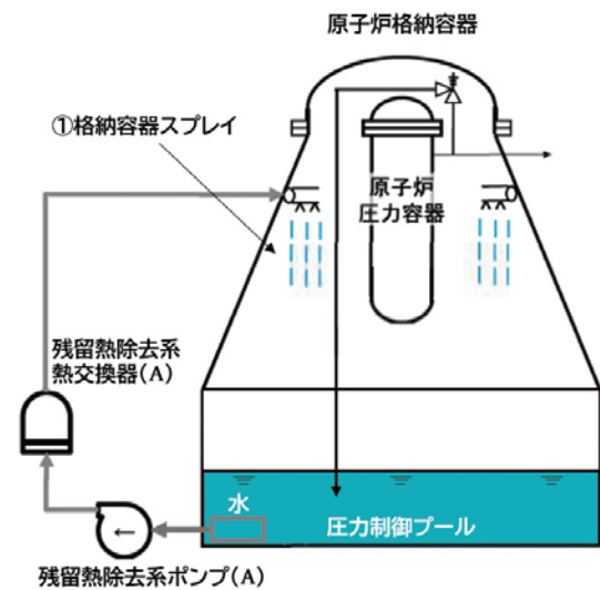
図2 既存の冷却設備(残留熱除去系)
