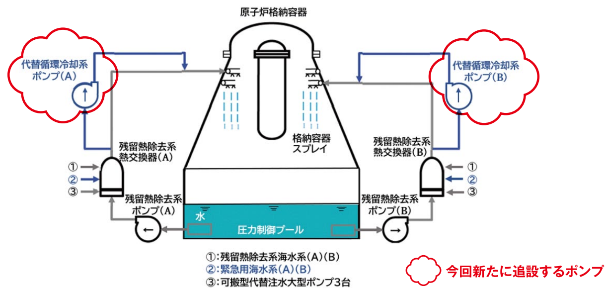
図3 新たに設置する冷却設備(代替循環冷却系)
