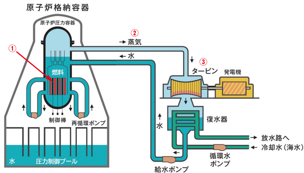
図1 原子力発電の仕組み
