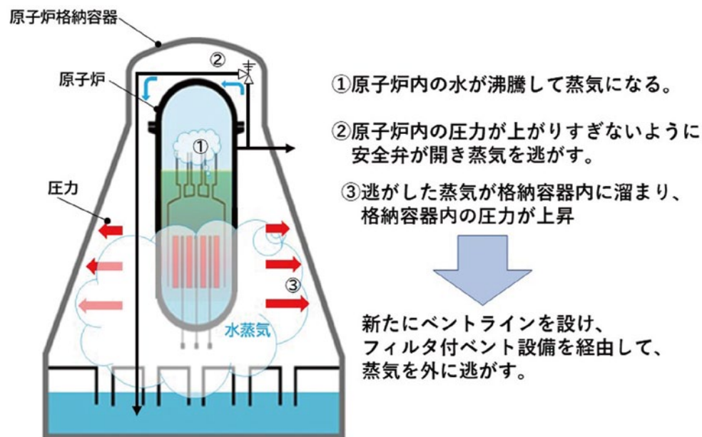
原子炉格納容器のイメージ
