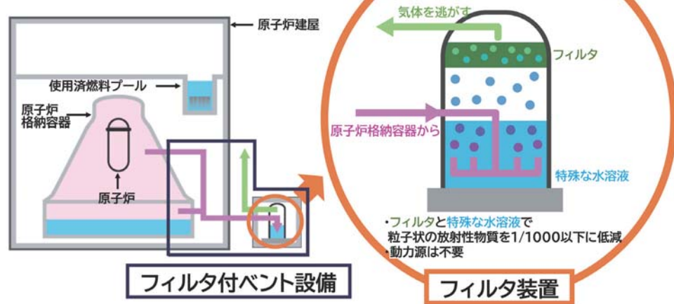
図1 東海第二発電所 フィルタ付ペント設備の概要
