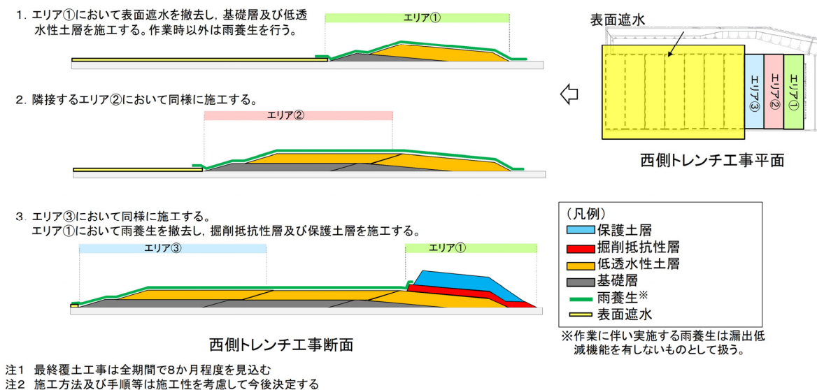
第4図 最終覆土の設置中のイメージ図
