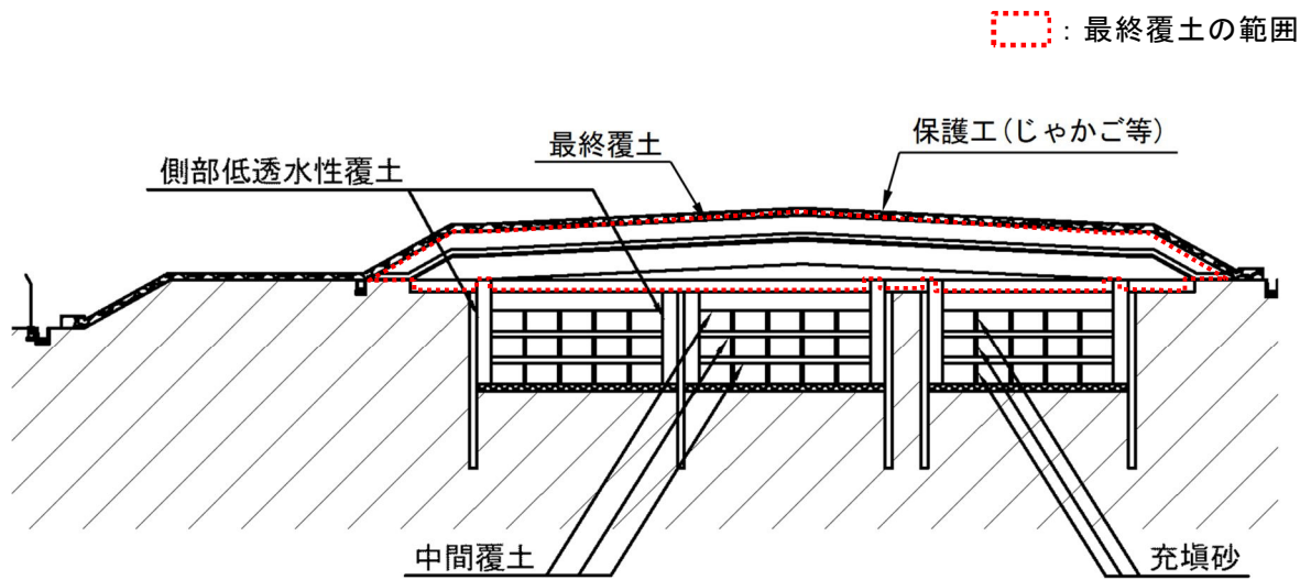
第 6 図 覆土の断面図（西側 X-X 断面）
