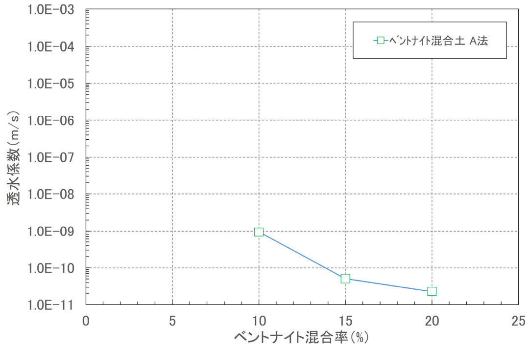
第 1 図 ベントナイト混合率と透水係数の関係
