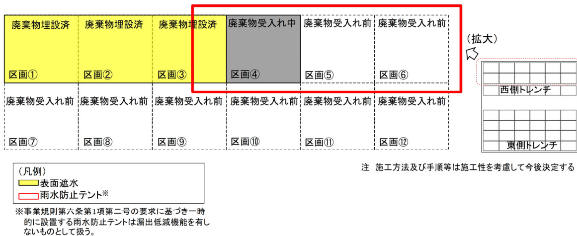
第3図 放射性廃棄物の受入れ中のイメージ図
