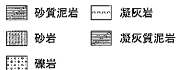
第 2. 2. 2 図 (5) 地質柱状図 (D-4-0 孔) (その 3)
