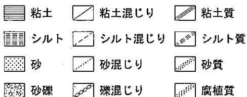
第 2. 2. 2 図 (5) 地質柱状図 (D-4-0 孔) (その 3)
