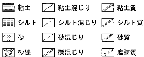
第 2.2.2 図(4) 地質柱状図 (D-4-0 孔) (その 2)
