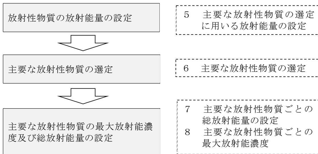
第 1 図 廃棄物の主要な放射性物質の最大放射能濃度 及び総放射エネルギーの設定フロー
