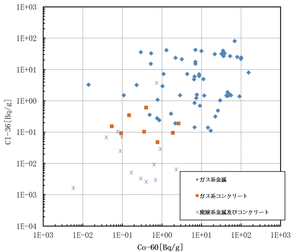
第 2 図 \text{Cl-36} と \text{Co-60} の分析データ (2019 年度まで)
