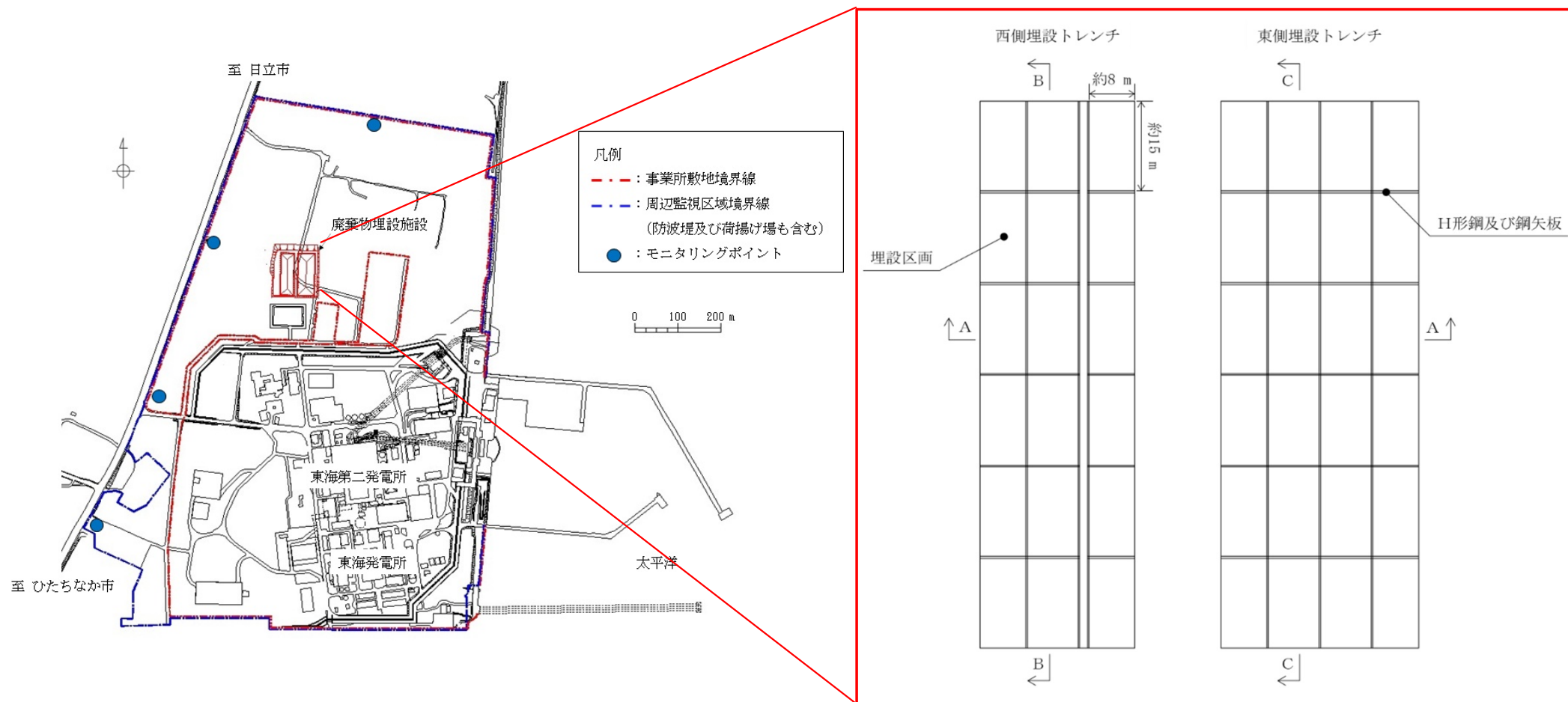
第13-1図 廃棄物埋設地の区画配置図(平面図)
