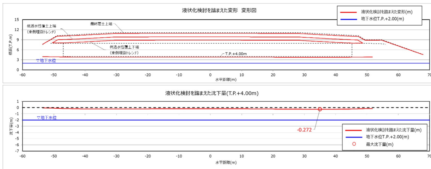
第3-1図 液状化を踏まえた検討による変形図及び沈下量分布図(N-S断面)
