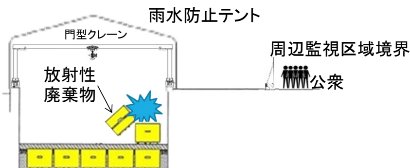
第11-1図 放射性廃棄物落下事象による被ばく評価イメージ
