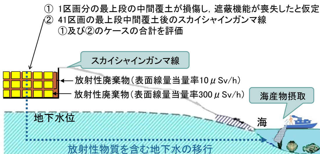
第4-1図 被ばく経路
