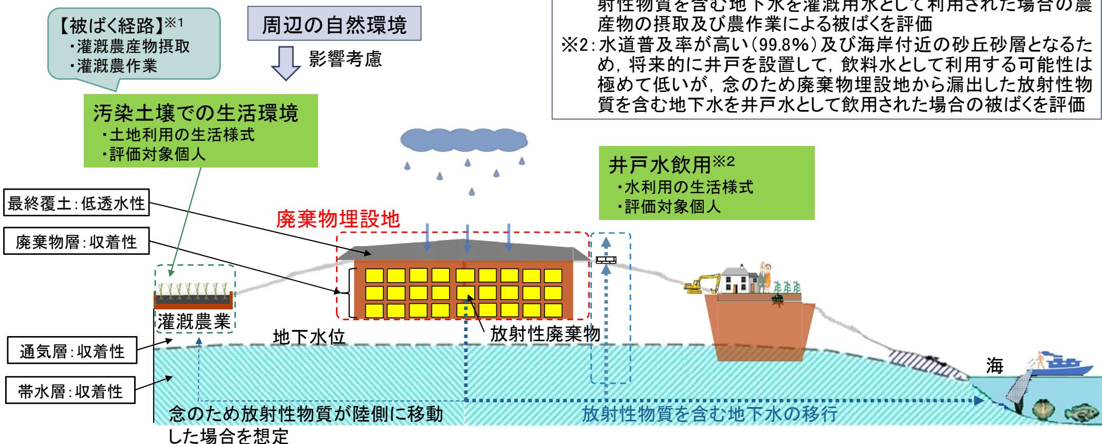
第13-6図 自然事象シナリオの評価概念図(最も厳しい自然事象シナリオのみ評価するシナリオ)
