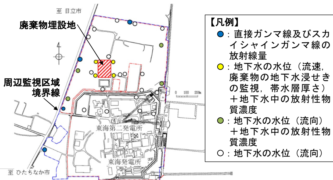
第15-1図 廃棄物埋設施設の監視測定位置の設置箇所概略図（平面図）
