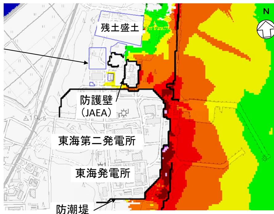
第5-1図 津波数値シミュレーション結果
