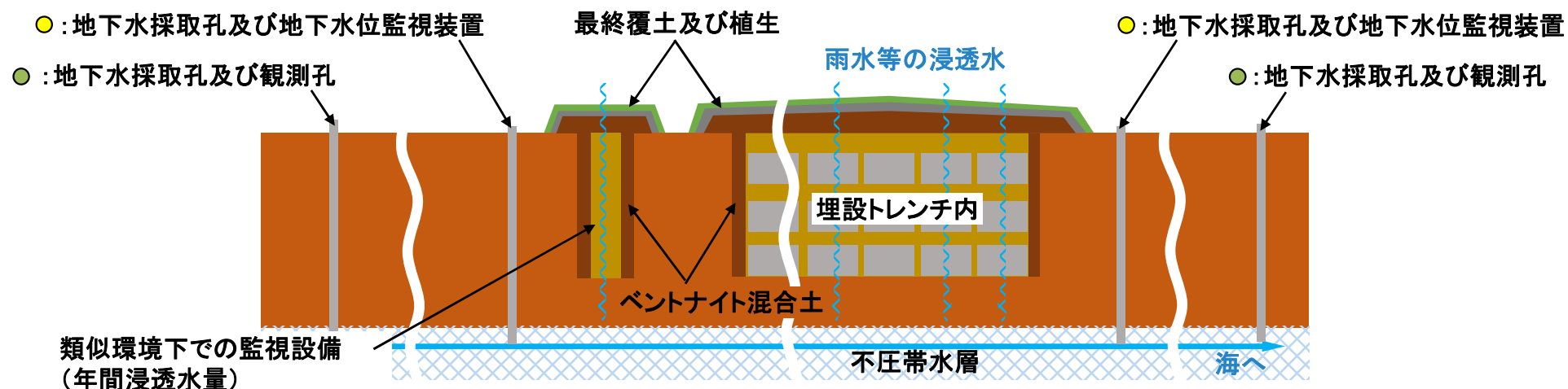
第15-2 図 監視測定設備の概略(断面図)
