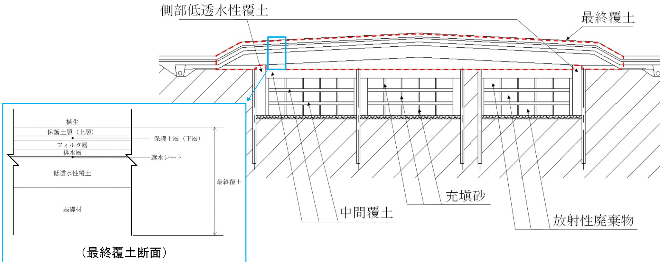
第13-3図 覆土の断面図
