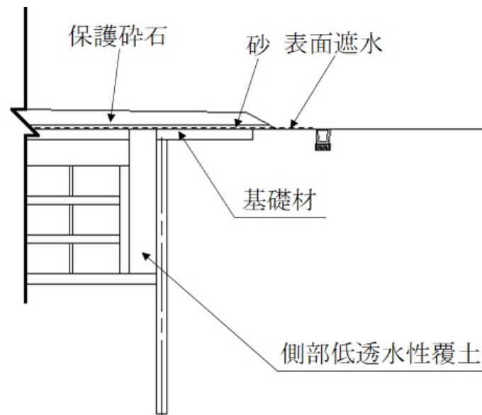
第13-4図 表面遮水の設置例
