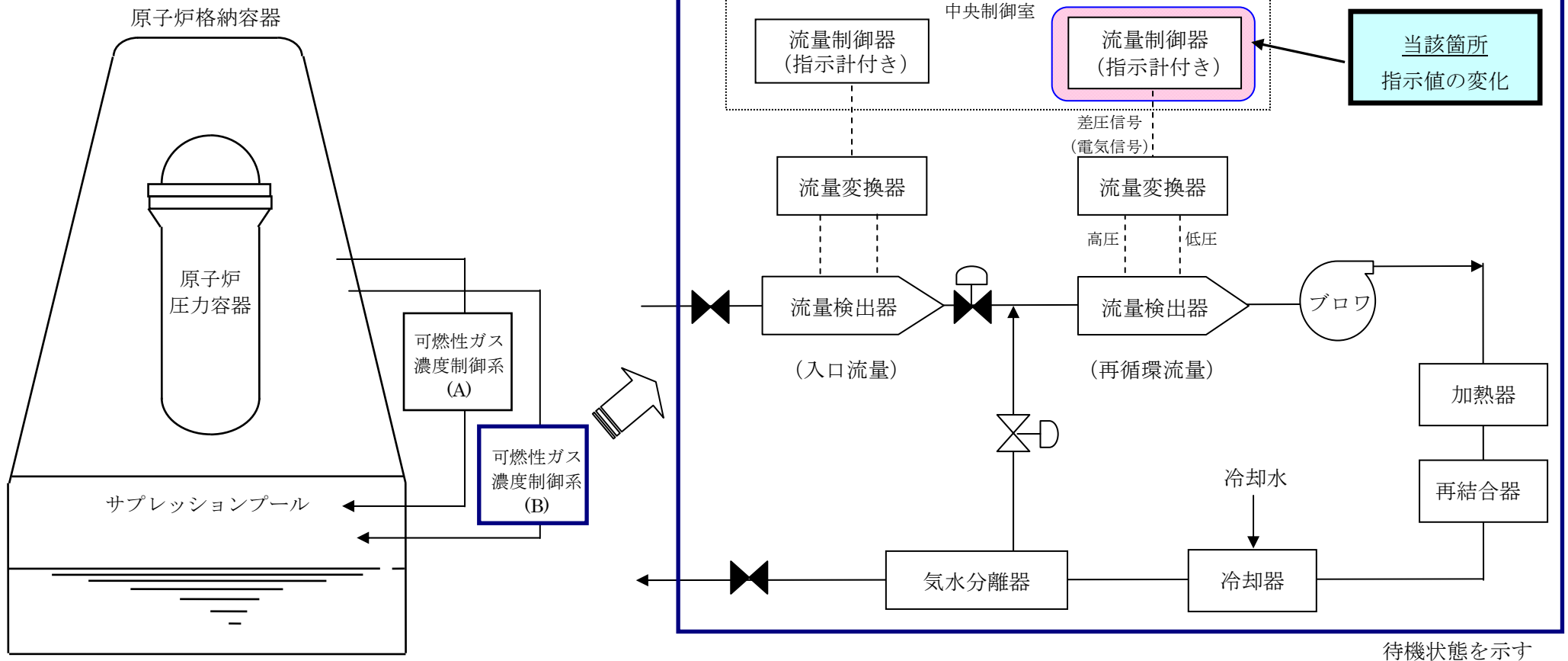
[可燃性ガス濃度制御系 (B) 拡大図]
