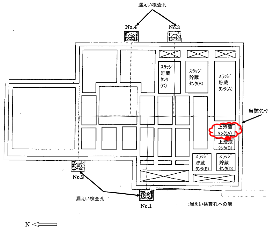
図1 地下タンク配置図
