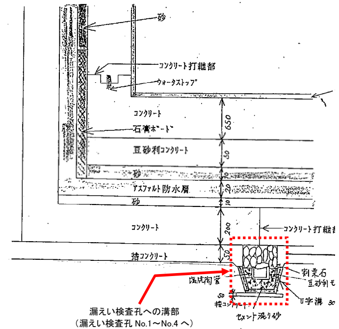
図2 漏えい検査孔への溝断面図
