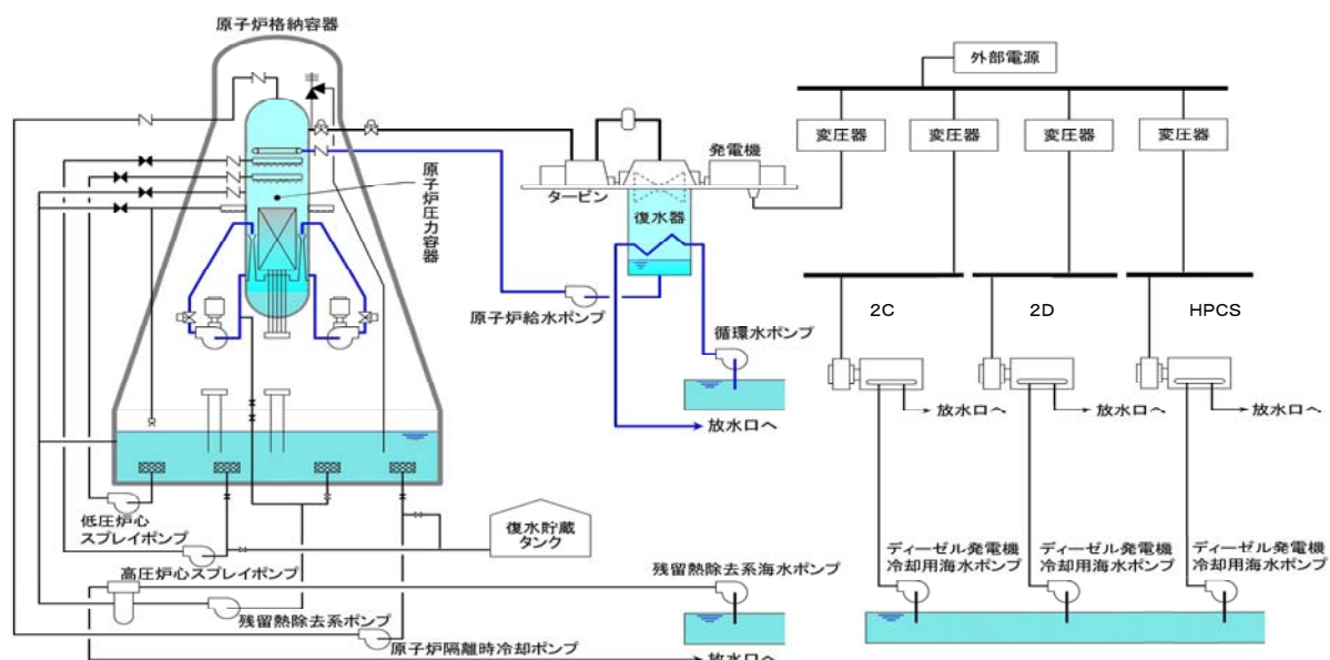
非常用ディーゼル発電機 概略図
