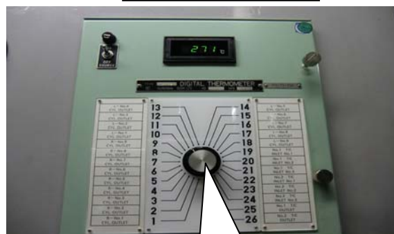
シリンダ排気温度
