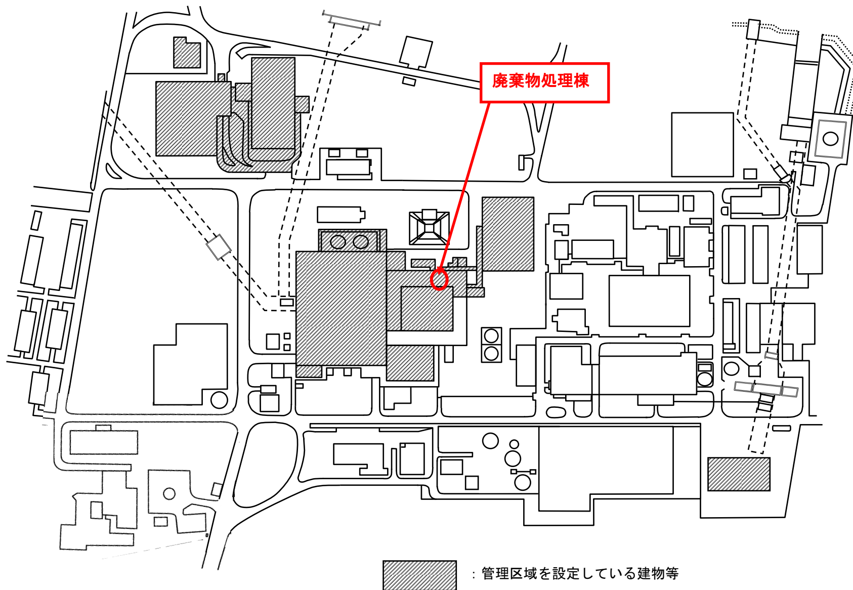
東海第二発電所 建屋配置図
