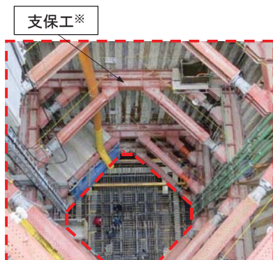
鉄筋設置状況（2021年3月）
