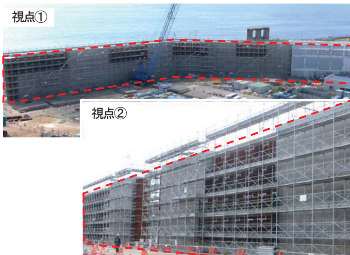
防潮堤(南・北側)の状況 赤枠: 鉄筋コンクリート施工箇所
