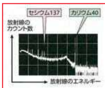
\gamma 線スペクトル
