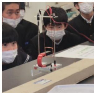
電磁力実験
