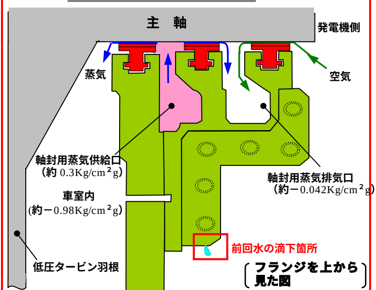
軸封部フランジ (平面図)
