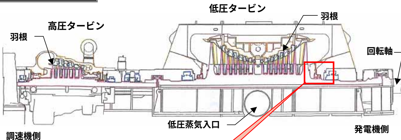
タービン断面図
