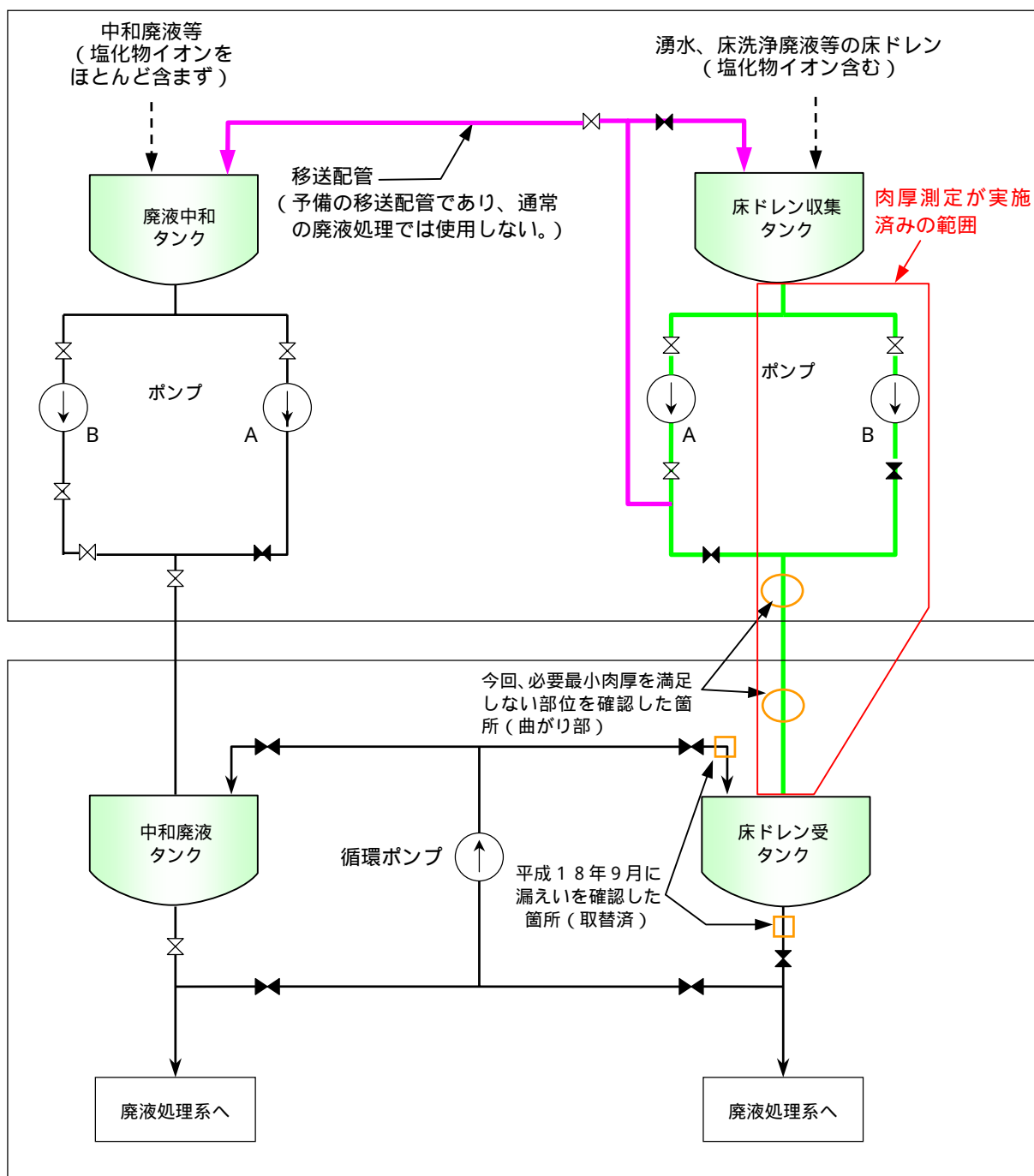
液体廃棄物処理系概略系統図
