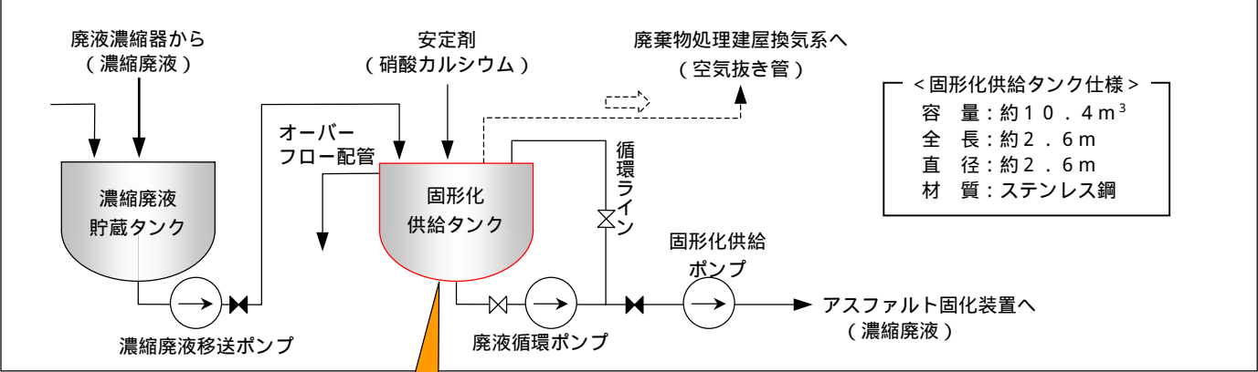
<濃縮廃液系概略系統図>
