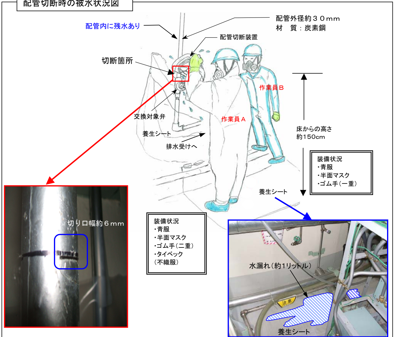
配管切断時の被水状況図
