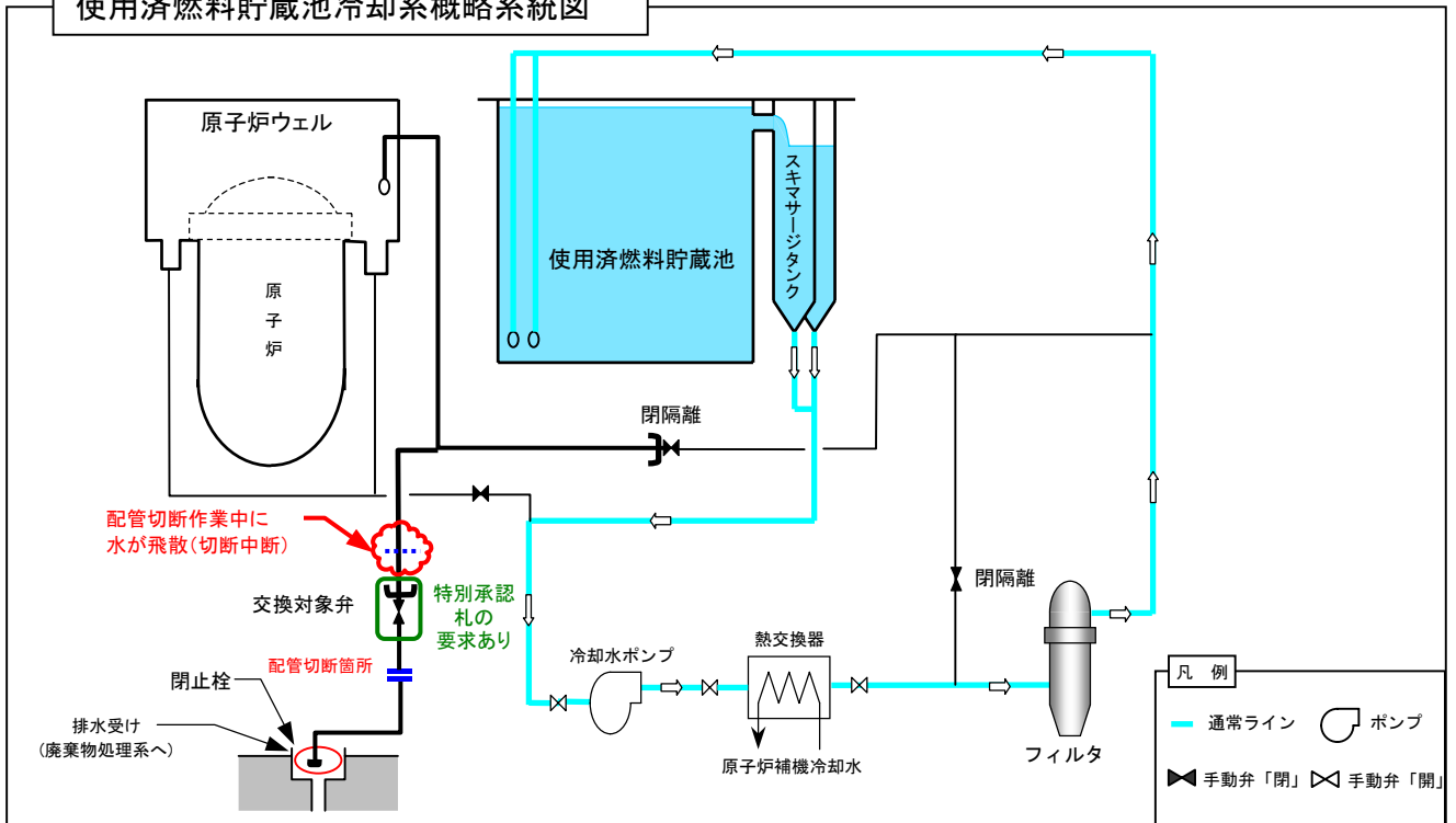
使用済燃料貯蔵池冷却系概略系統図
