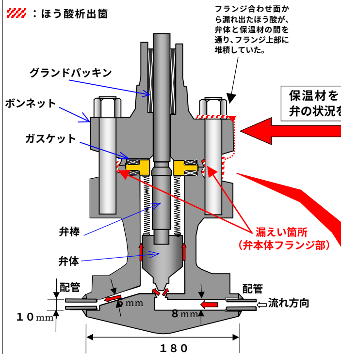
当該弁概略図
