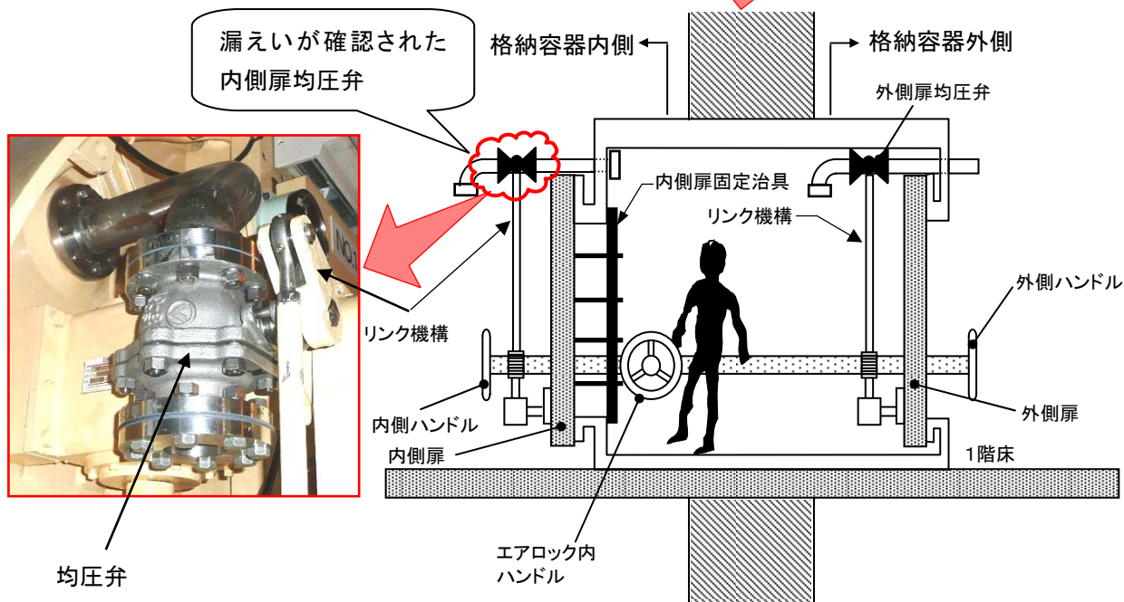
エアロック構造図
